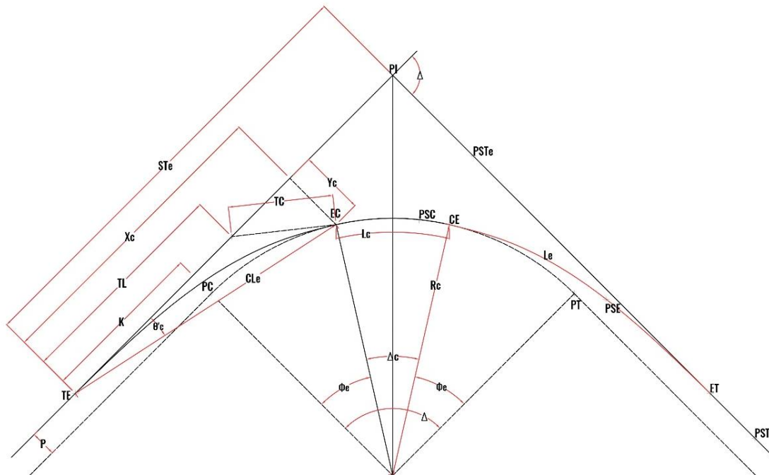
Figura 4-2. Elementos de una curva con espiral de transición.
