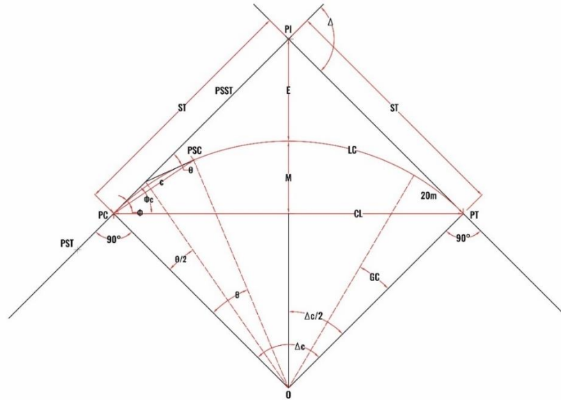
Figura 4-1. Elementos de las curvas circulares simples. (Secretaria de Comunicaciones y Transportes, 1991).
