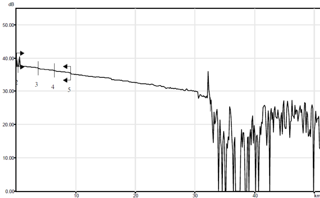
Figura 2.3. Trazo de medición de enlace B.
