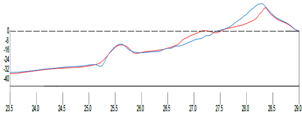
Figura 38 – Perfil con estructura a 30 cm, tormenta 1 ( H = 0.10 m, T = 1.118 s, h = 0.48 m) (Cárdenas, 2017)
