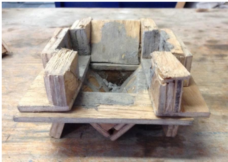
Figura 26 – Segundo prototipo de cimbra
