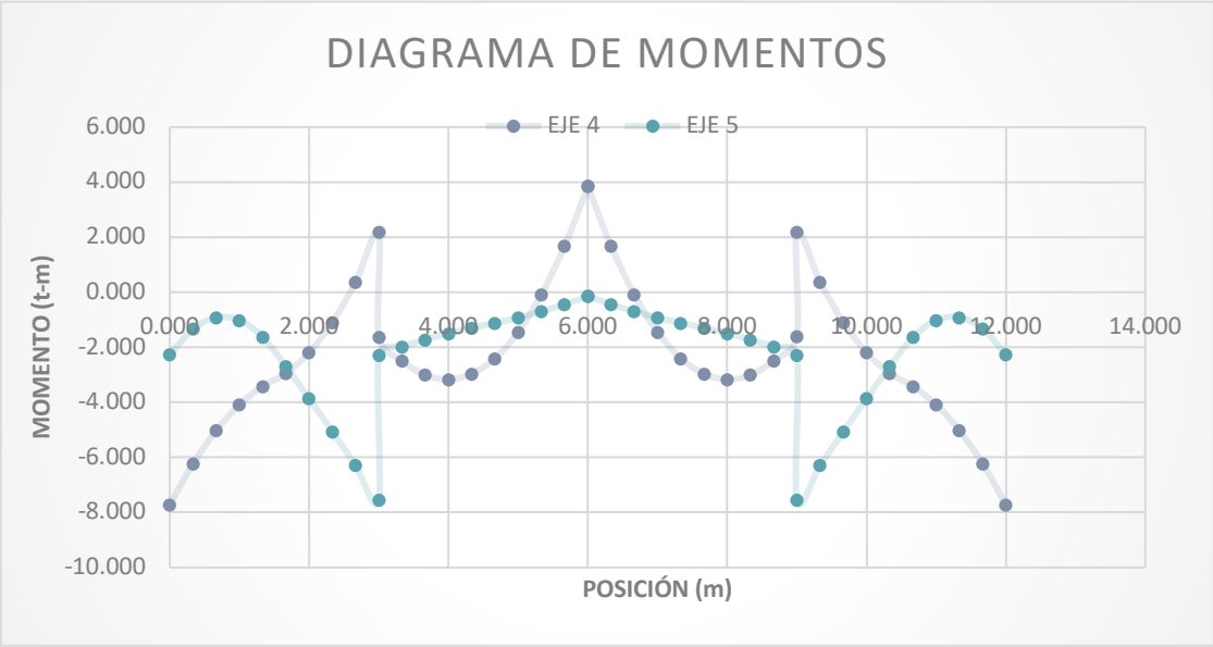
Figura 4.2.3 Momentos debidos a la excavación
