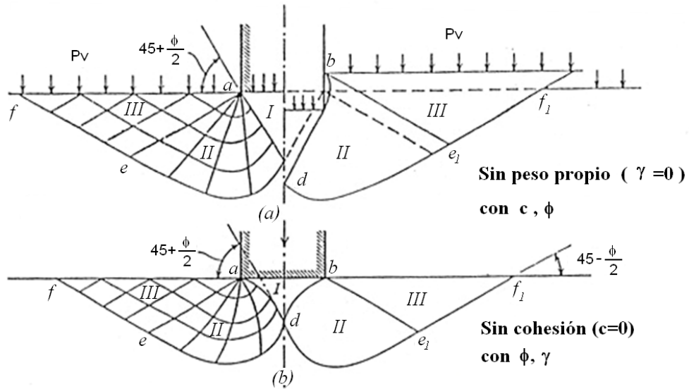
Figura 2.1 Zonas de equilibrio plástico después de la falla (Terzaghi y Peck, 1967)
