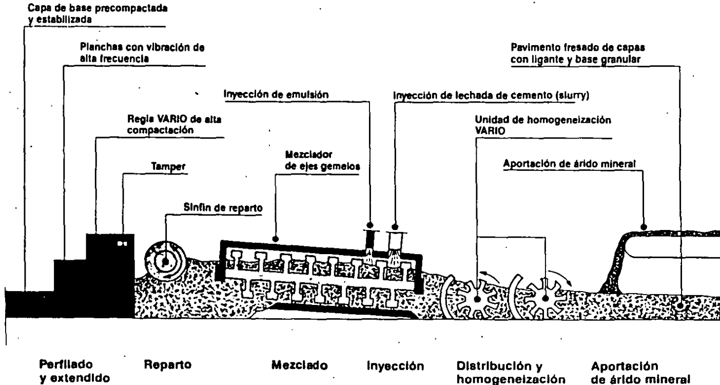
Principio de trabajo del proceso tal como lo realiza la recicladora en frío CR 4500.
