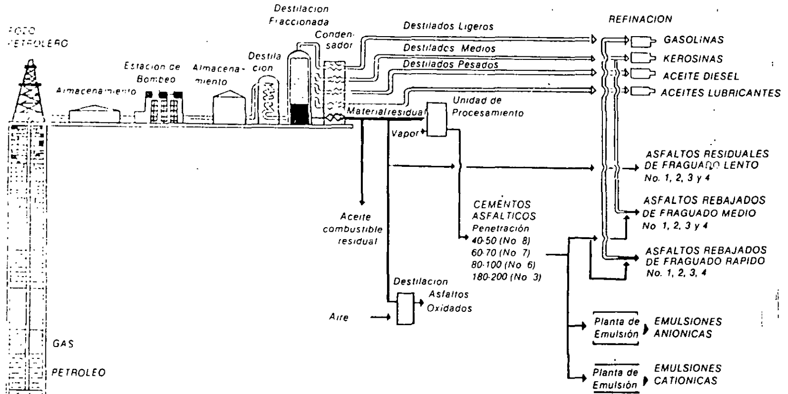
FIGURA 1. ESQUEMA DEL TRATAMIENTO DEL PETROLEO PARA OBTENER LOS DIVERSOS PRODUCTOS ASFALTICOS
