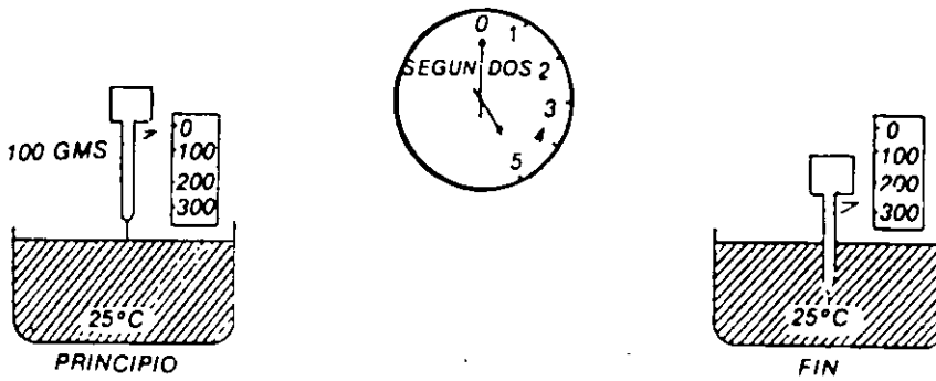
PENETRACION 25^{\circ}\text{C} , 100 GMS Y 5 SEG.
