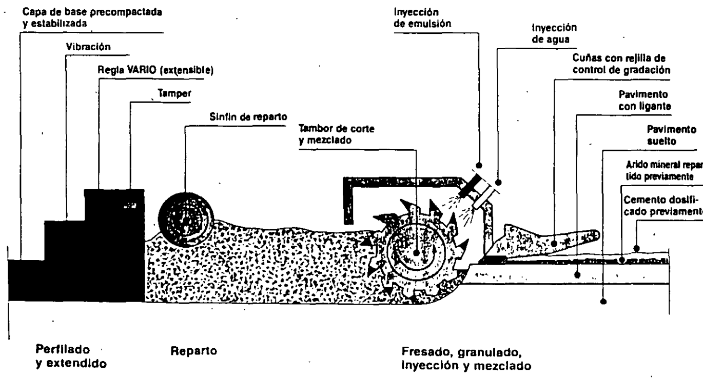
Principio de trabajo del proceso tal como lo realiza la recicladora en frío 2100 DCR.
