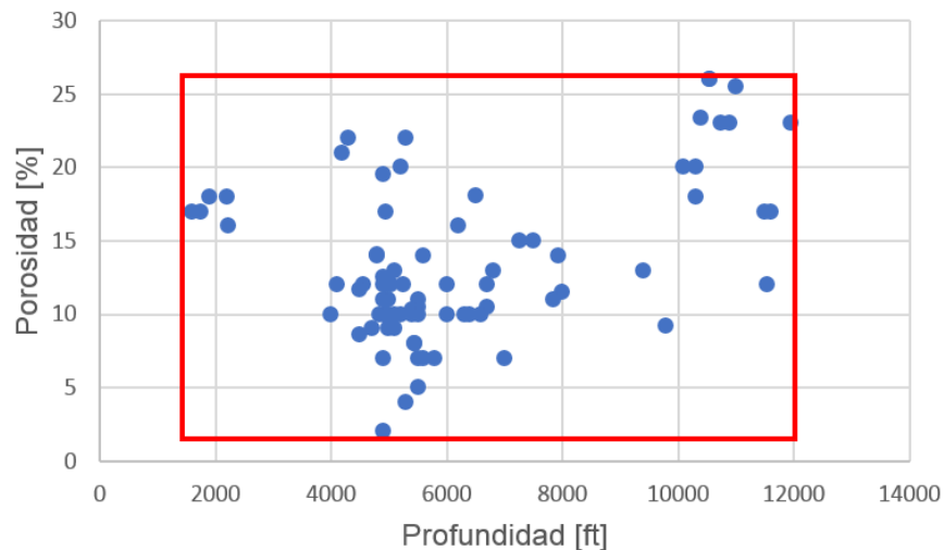
Figura 5.6 Profundidad vs porosidad de proyectos análogos exitosos. Elaboración propia con datos de Oil & Gas Journal
