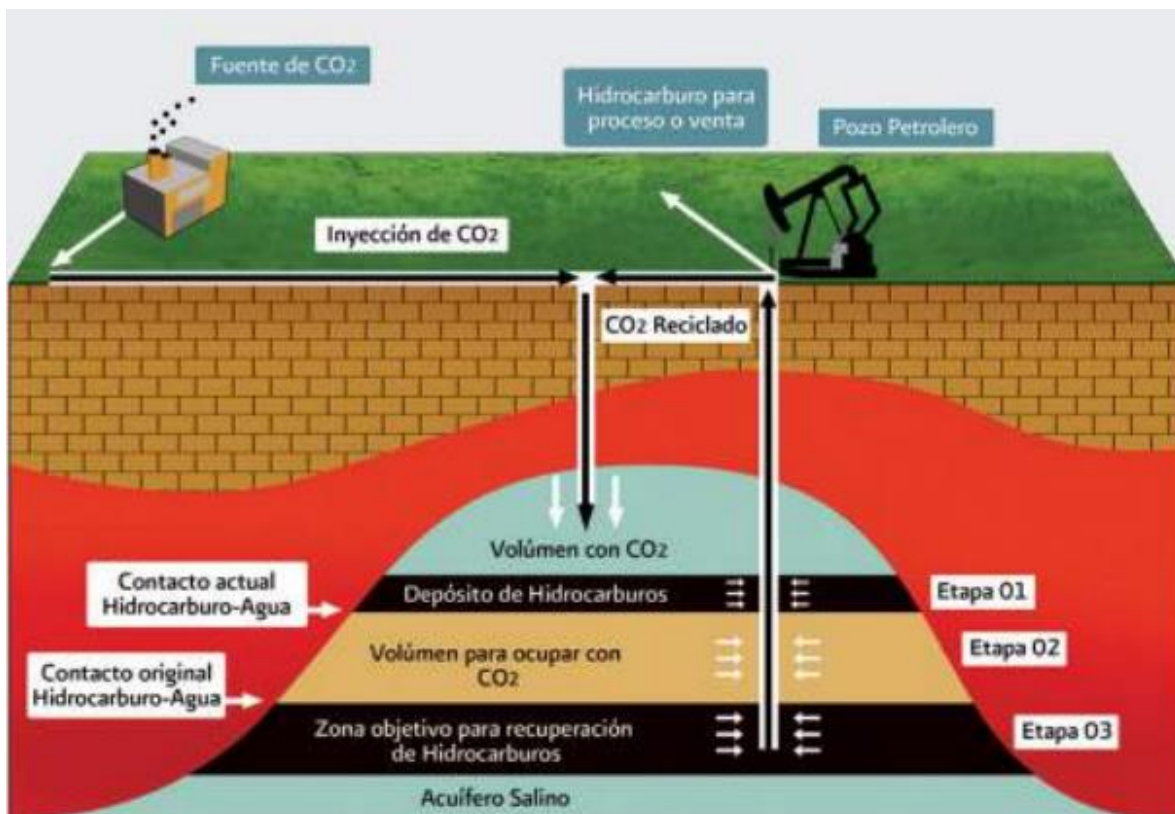
Figura 2.6 Esquema de recuperación mejorada de hidrocarburos con inyección de CO 2 , SENER (2014)
