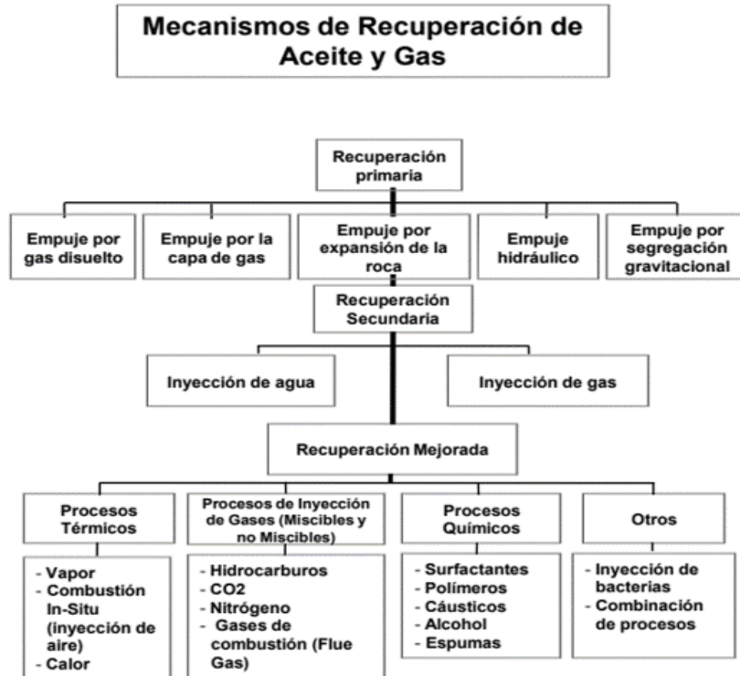
Figura 3.3 Métodos de recuperación de hidrocarburos, CNH (2012)
