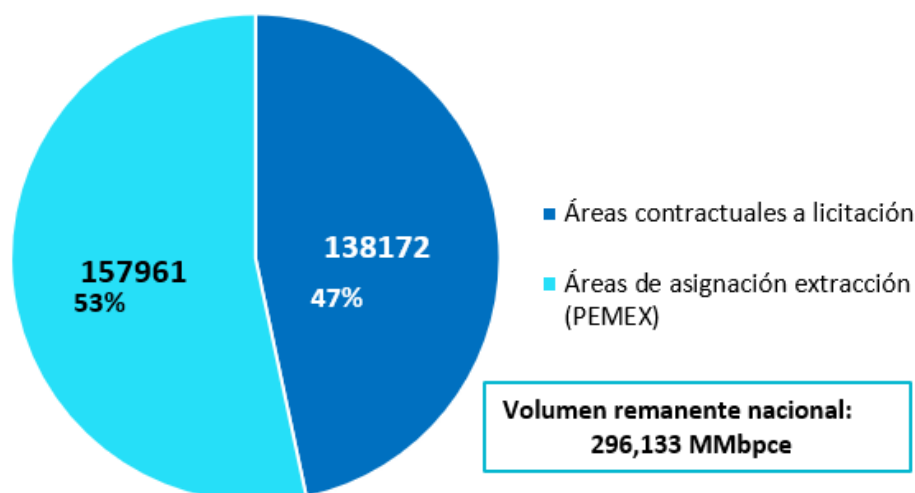
Figura 4.6 Porcentaje de volumen remanente de hidrocarburos para las áreas de asignación y contractuales, Elaboración propia con datos de CNH (2018)
