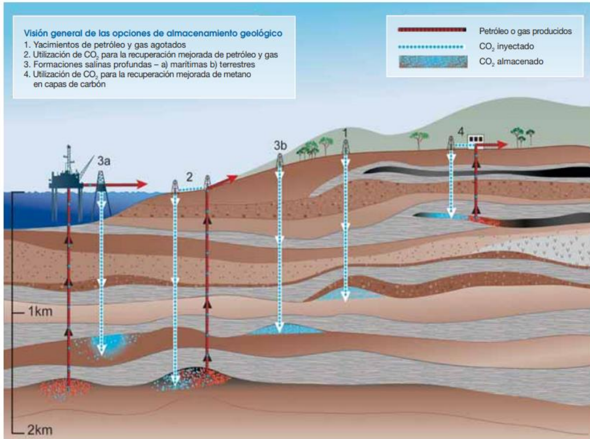
Figura 2.4 Métodos de almacenamiento geológico de CO 2 , IPCC (2005)
