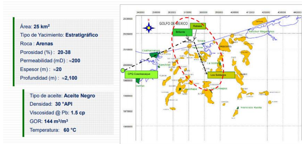
Figura 6.2 Esquema del proyecto piloto Cosoleacaque – Brillante, CONACYT (2018)
