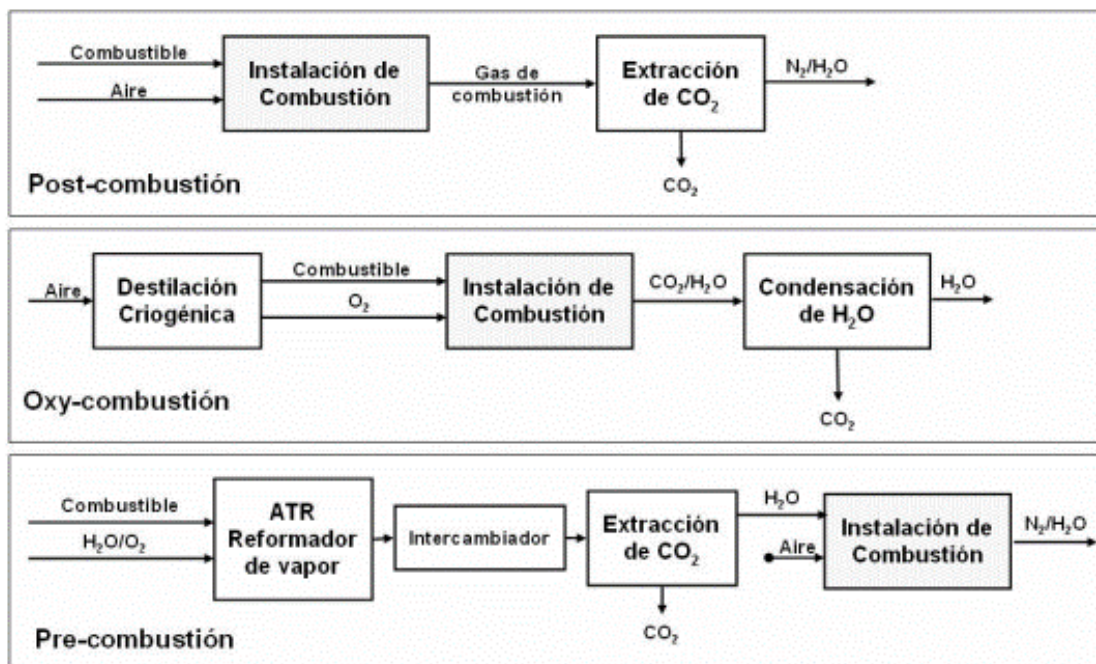
Figura 2.3 Tecnologías existentes para captura de CO 2 , Lacy (2005)
