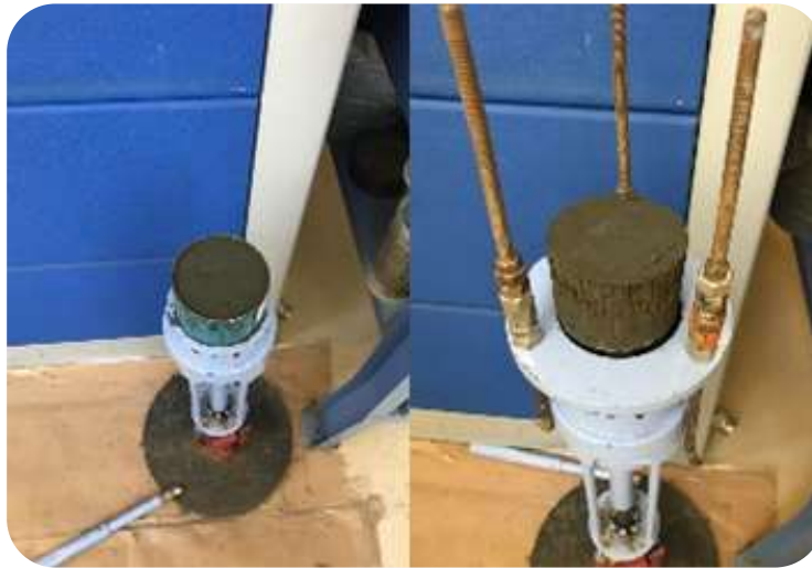
Figura A. 1 Extracción de muestra de tubo, para realizar pruebas
