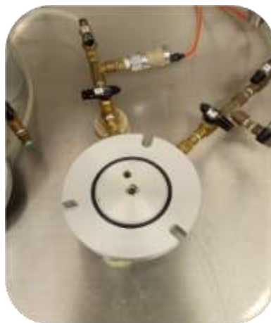
Figura 3.2 Base de la Celda Rowe con conexiones para presión de poro y contrapresión.
