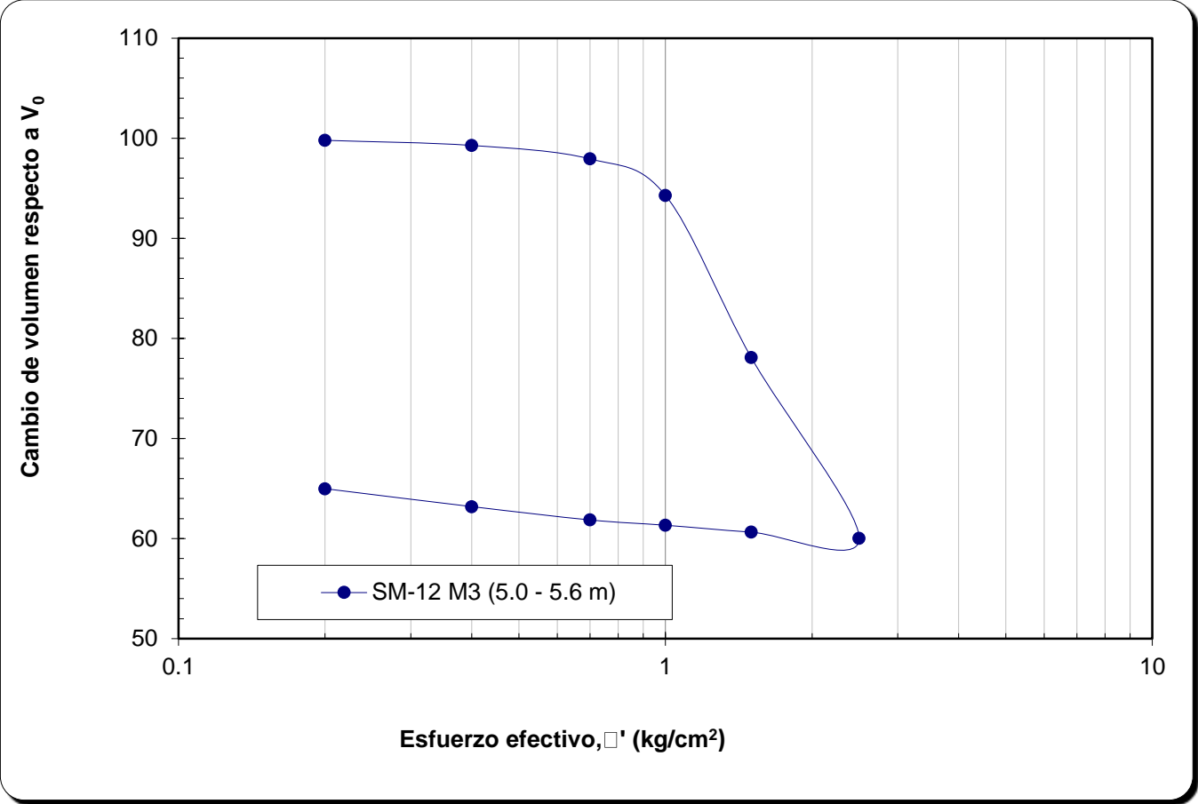
Figura 6.20 Curva de compresibilidad " Sondeo NAICM SM-12 M-3" Profundidad: 5.0 a 5.60 m
