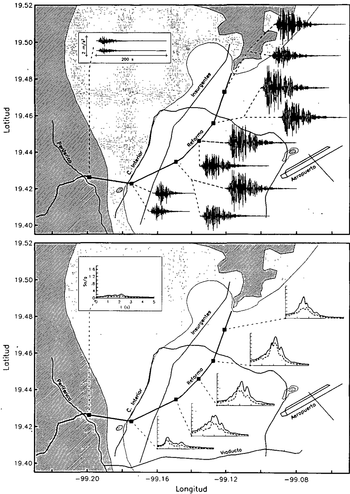
Figura 17. Parte superior: Acelerogramas sintéticos para dos sismos de subducción ( M=8 generados en las brechas de San Marcos (arriba) y de Michoacán (abajo). Parte inferior: Espectros de respuesta. Con líneas continua y discontinua se indican los espectros para San Marcos y Michoacán, respectivamente.
