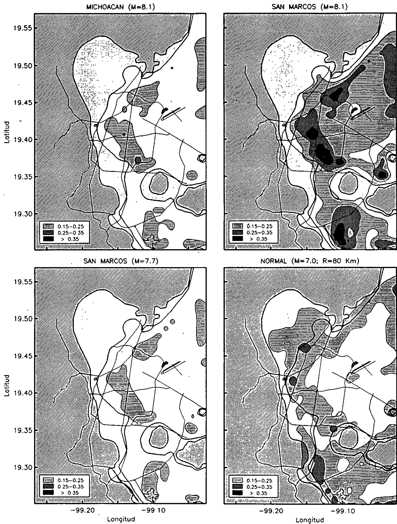
Figura 13. Distribución de aceleraciones máximas del terreno ( S_a/g ) en el valle de México, correspondientes a posibles sismos de subducción de magnitud M=8.1 originados en las costa del Pacífico Mexicano y en el interior del continente.
