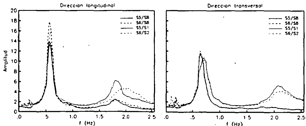
Figura 6 Funciones de transferencia de azoteas relativas a a) campo libre (líneas gruesas) y b) sótanos (líneas finas)
