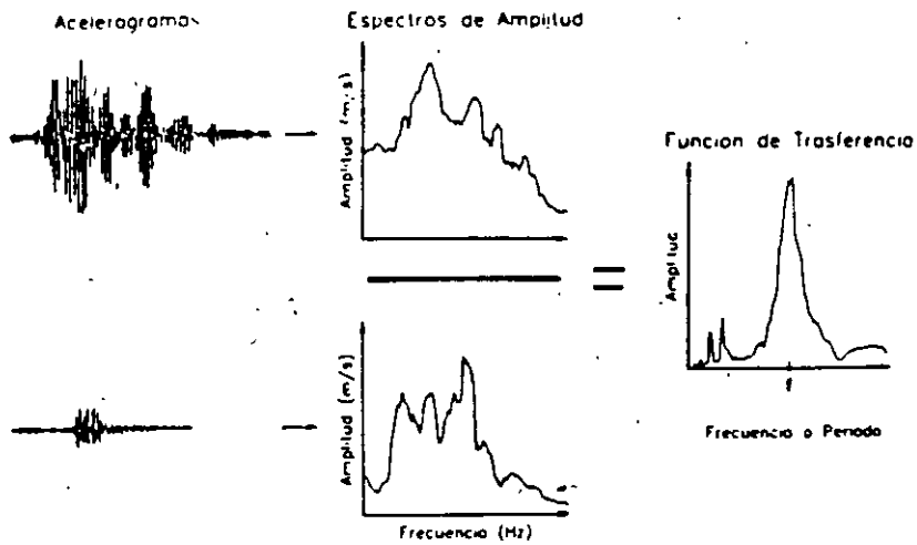
Fig 23 Obtención de un cociente espectral o función de trasferencia empirica
