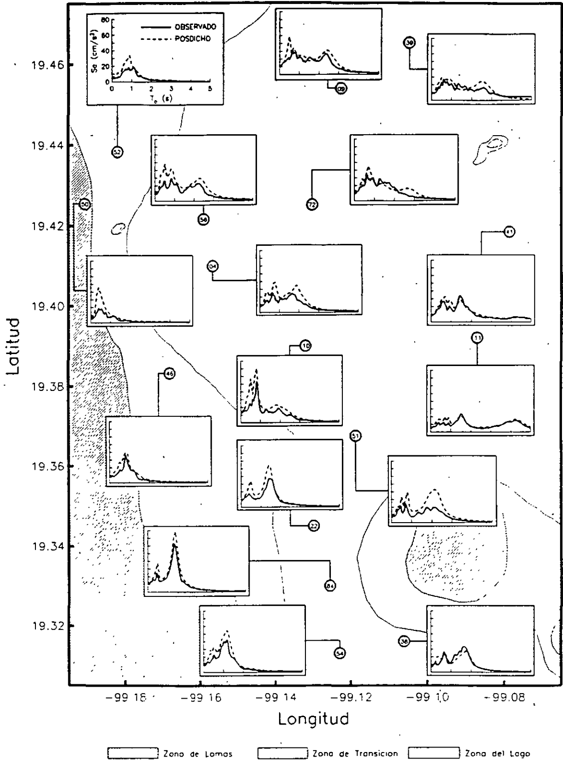
Fig 3 Espectros de respuesta observados para el sismo del 23 de mayo (línea discontinua) y espectros de respuesta obtenidos con las FTE y el espectro de Fournier observado en CU (línea continua)
