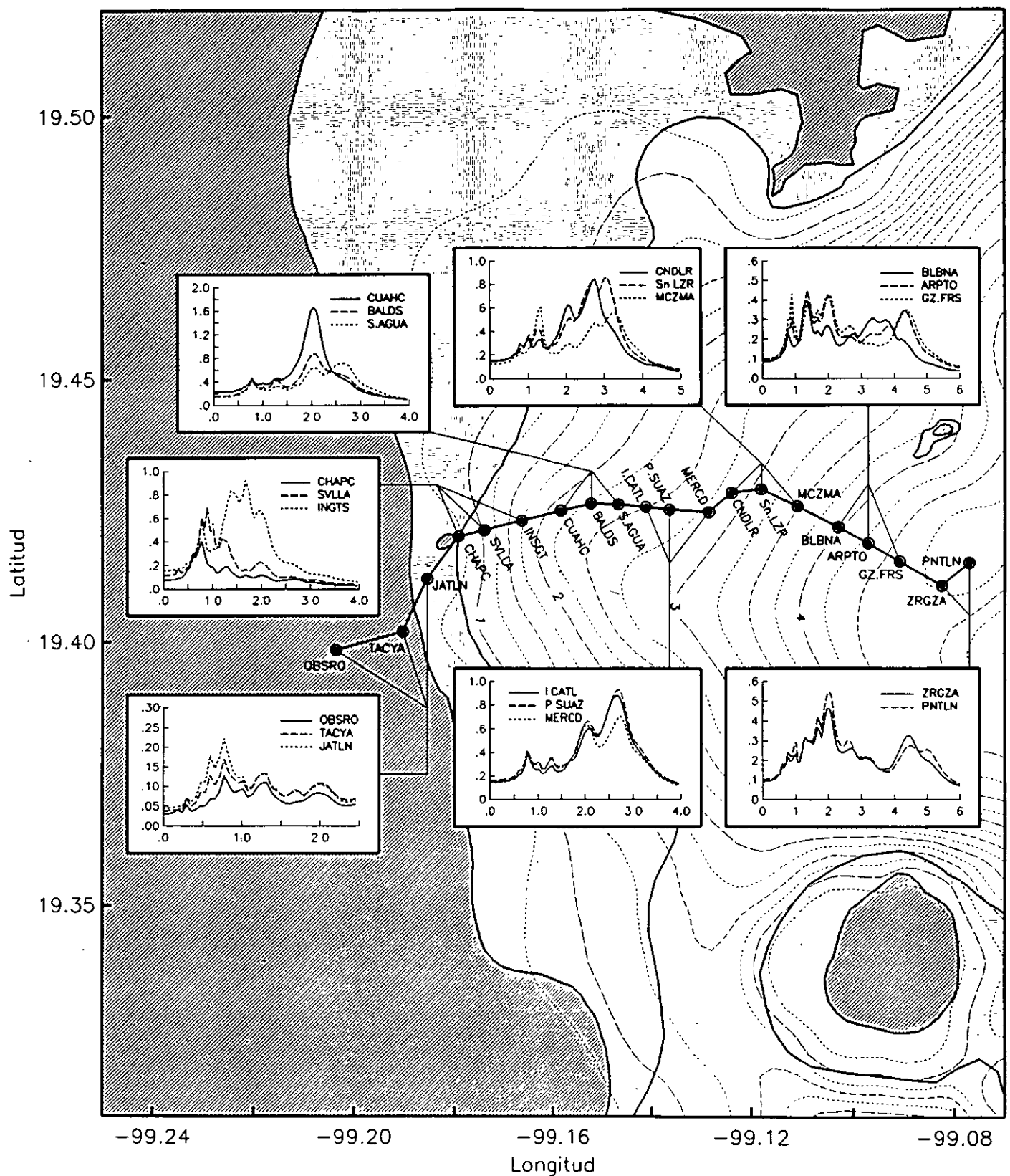
Figura 9. Espectros de respuesta para las estaciones de la Línea 1 del Sistema de Transp. Colectivo de la Ciudad de México. Se indican algunas curvas de isoperiodos dominantes del Terreno como referencia adicional.
