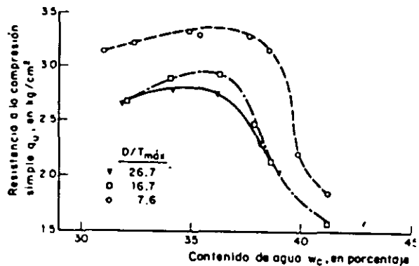
Fig. 11 Variación de la resistencia q_u y el efecto de escala
