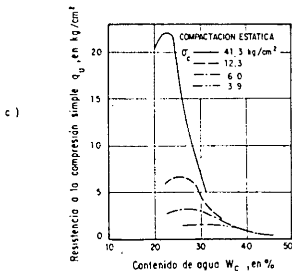
Fig 7. Resistencia a la compresión simple q_u para distintos tipos de compactación, en función del contenido de agua de compactación w_c (Ref. 1).
