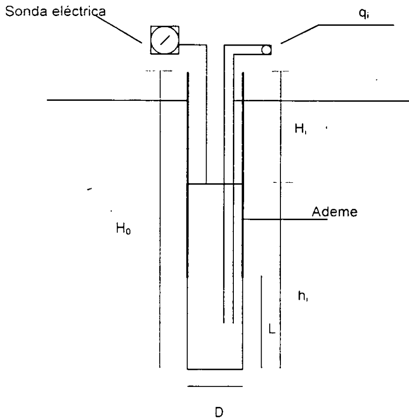
FIG 59 PRUEBA DE PERMEABILIDAD NASBERG
