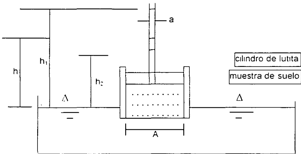
Fig. 5.2 Permeámetro de carga variable
