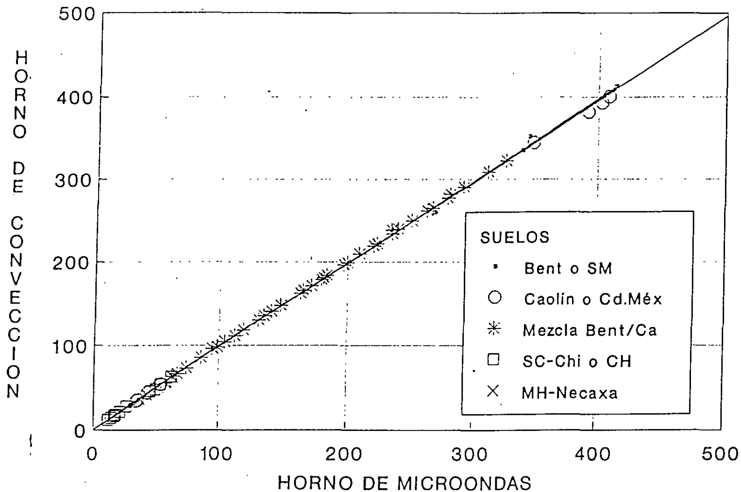
Fig 3.3 Correlación entre los contenidos de agua de diversos suelos, obtenidos con el HMO y el HC
