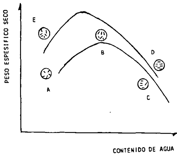
FIG 4 EFECTO DE LA COMPACTACION EN LA ESTRUCTURA DEL SUELO
