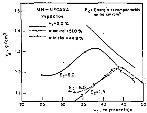
Fig. 14 Curvas de compactación por impacto del suelo MH-Necaxa con y sin secado previo
