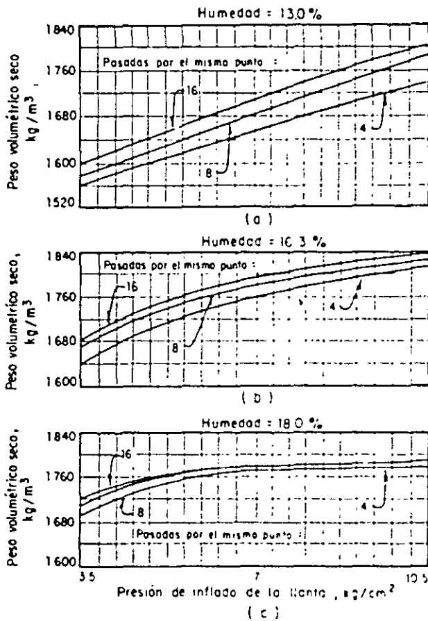
Fig 2. Efecto de la presión de inflado, del número de pasadas y de la humedad de compactación.
