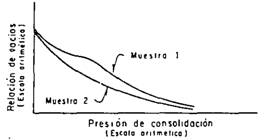
b) Curvas relación de vacíos - presión
