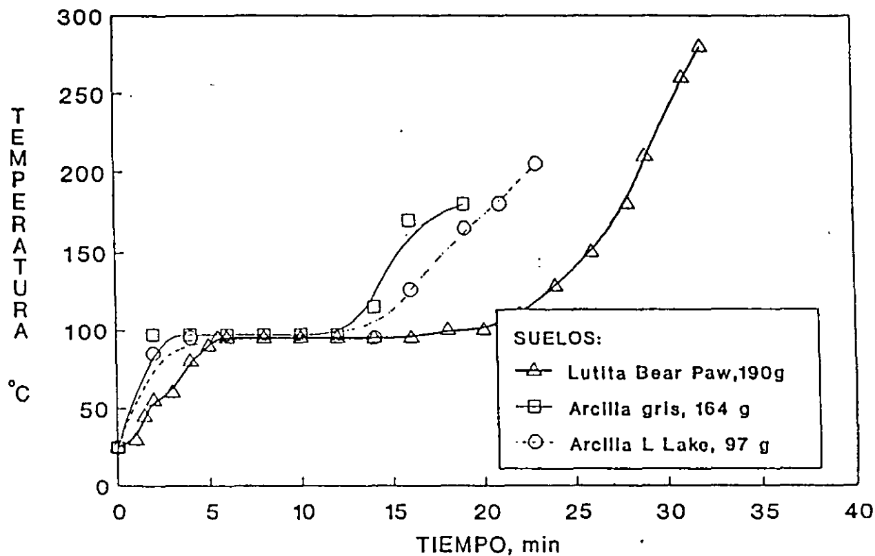
Fig 2.3. Variación de la temperatura con el tiempo, de diversos suelos con el HMO (Charlie, et al, 1982)
