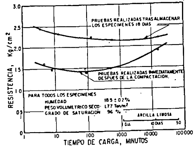
Figura 12 Efectos de tiempo en la resistencia de una arcilla limosa con alto grado de saturación
