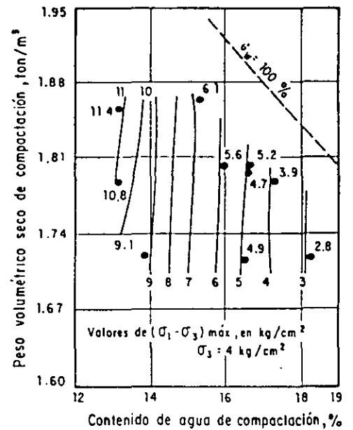
Fig 9. Líneas de igual resistencia a la compresión en prueba rápida, sin saturación previa y con presión confinante de 4 kg/cm².
