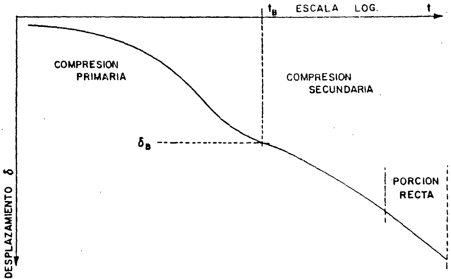
FIG- 2 CURVA DE CONSOLIDACION ANTES DEL ESFUERZO CRITICO
