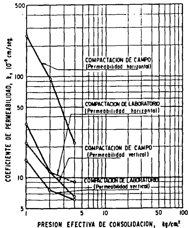
Figura 6 Diferencias de permeabilidad vertical y horizontal en muestras compactadas en el campo y en el laboratorio
