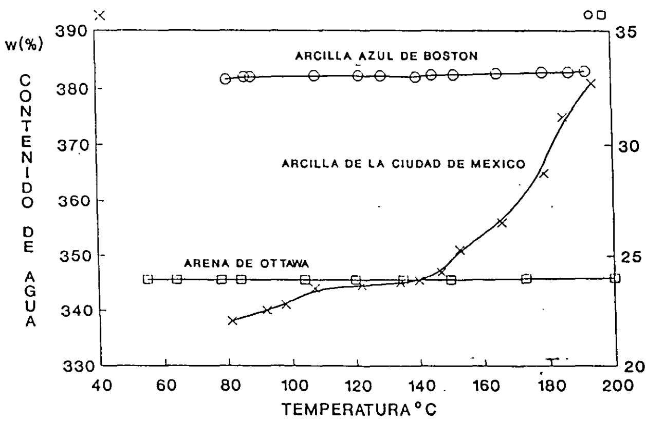
Fig 2.4. Variación del contenido de agua con la temperatura de diversos suelos en el HC (Lambe, 1949)
