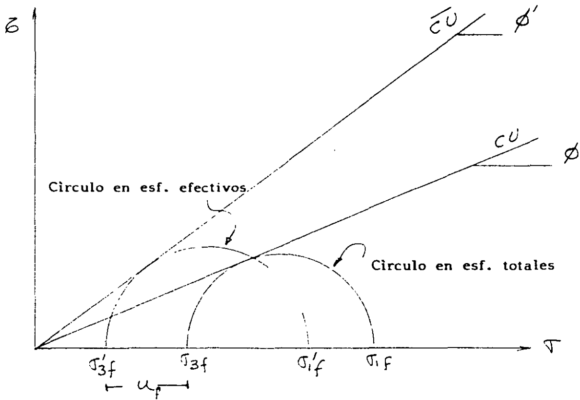
Fig. 7.3.8 Prueba triaxial de compresión CU
