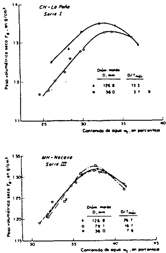
Fig. 10 Variación de las curvas de compactación por el efecto de pared
