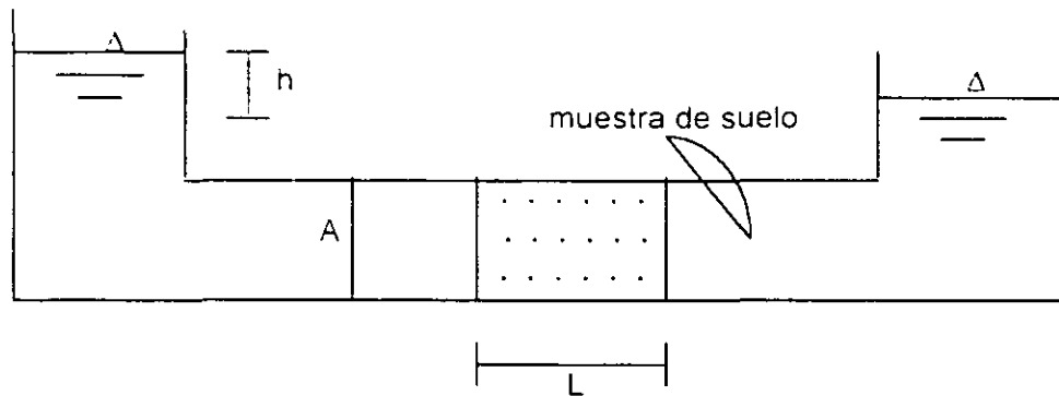
Fig. 5.1 Permeámetro de carga constante.
