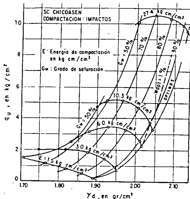
Fig 6. Resistencia no confinada en función de \gamma_d para valores diferentes de G_w .
