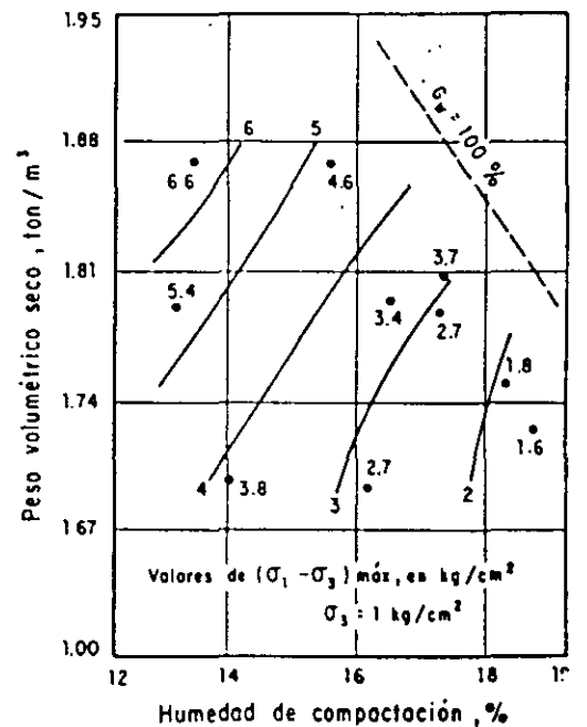
Fig 10. Líneas de igual resistencia a la compresión en prueba rápida, sin saturación previa y con presión confinante de 1 kg/cm².
