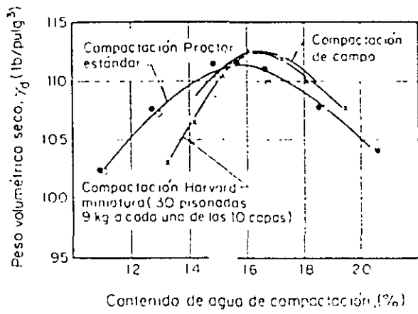
Fig. 1 Comparación de curvas de compactación de laboratorio y campo (en %)
