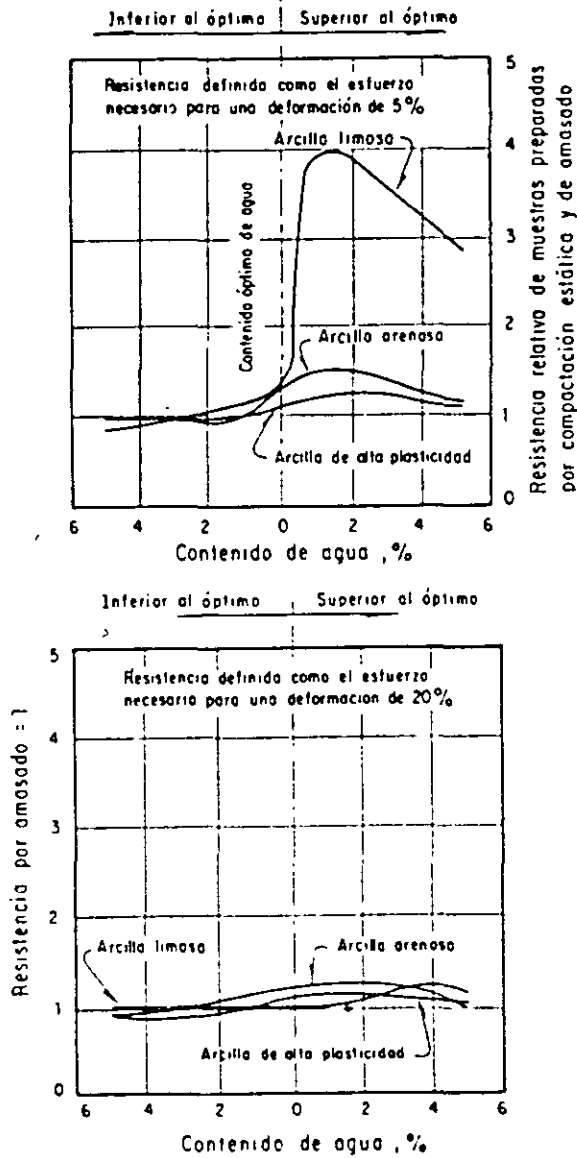
Fig 11. Efectos de procedimientos de compactación en la resistencia en prueba rápida (saturación previa de muestras compactadas a mismos \gamma_d y w ) con compactación estática y de amasado.
