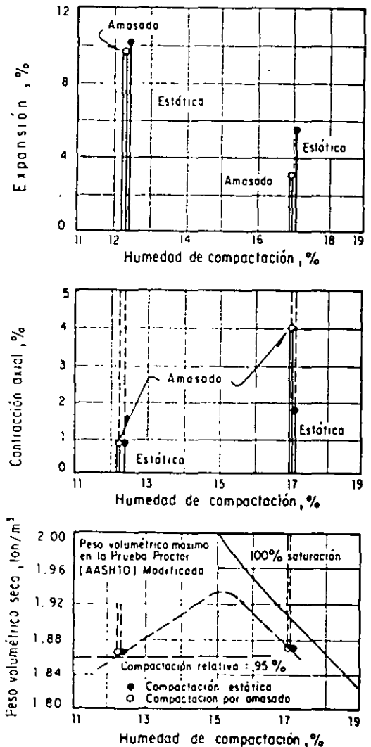
Fig 4. Expansión y contracción de una arcilla arenosa compactada estáticamente y por amasado.
