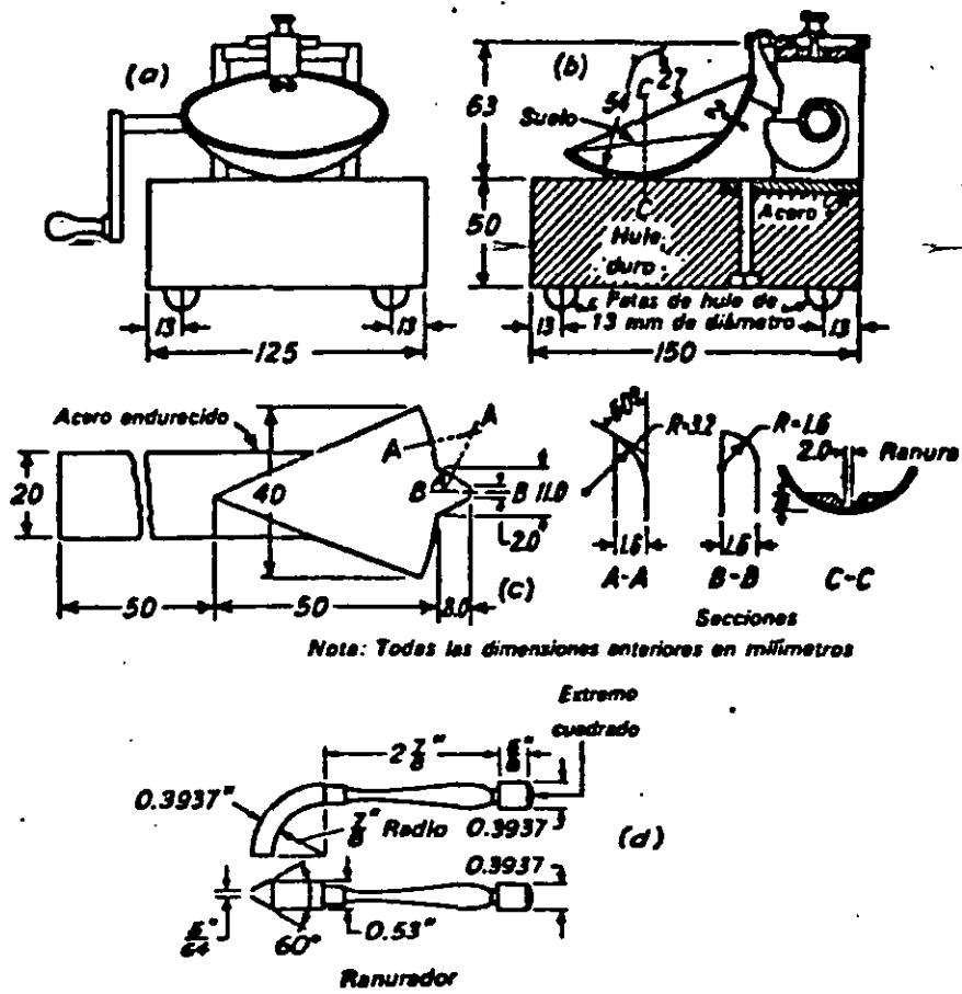
Figura 4 a) y b) Aparato mecánico para determinar el límite líquido. c) Ranurador de Casagrande. d) Ranurador estándar de la ASTM.
