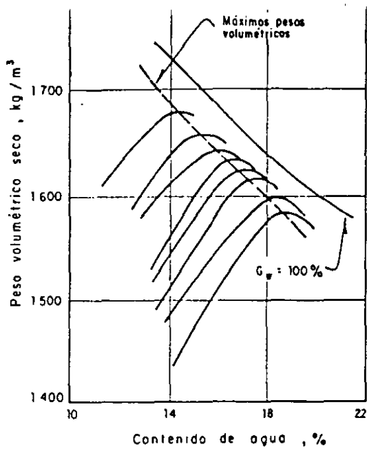
Fig 1. Diagrama cualitativo de \gamma_d vs. w para diversas energías de compactación.
