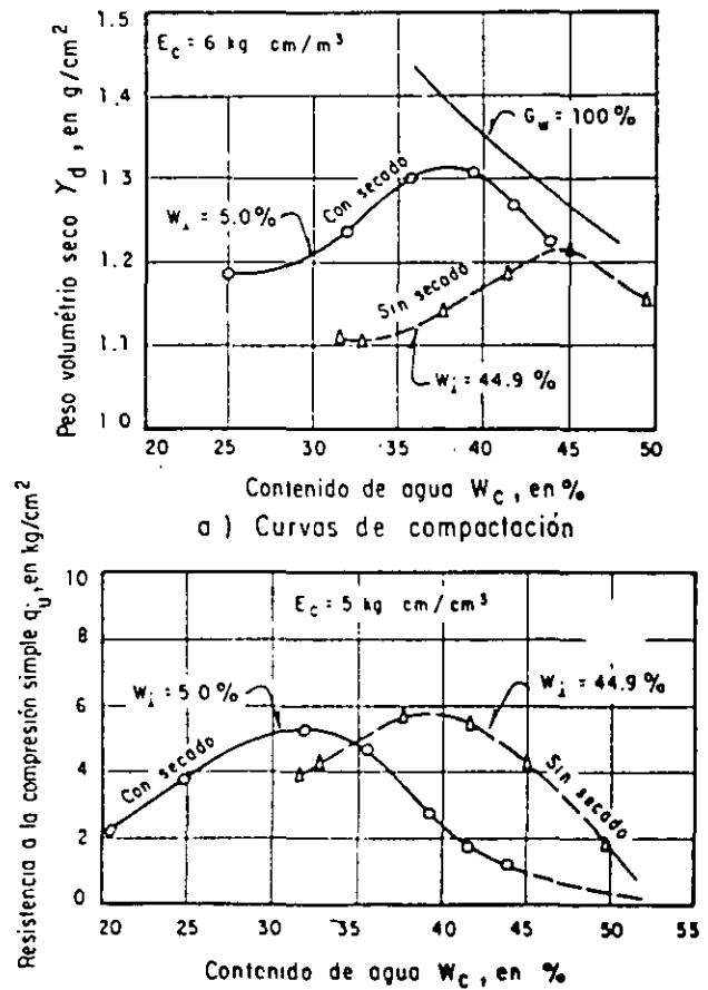
Fig 12. Efecto del contenido de agua inicial en los resultados de la compactación. (Ref. 1).
