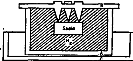
Figura A. 1 Método de Terzaghi para la determinación del volumen de muestra de suelo.
