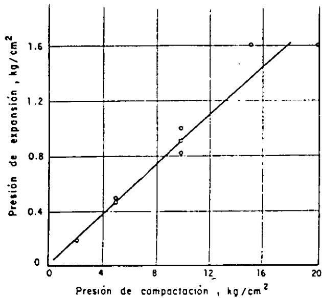
Fig 5. Relación entre presión estática de compactación y la presión de expansión en una arcilla.
