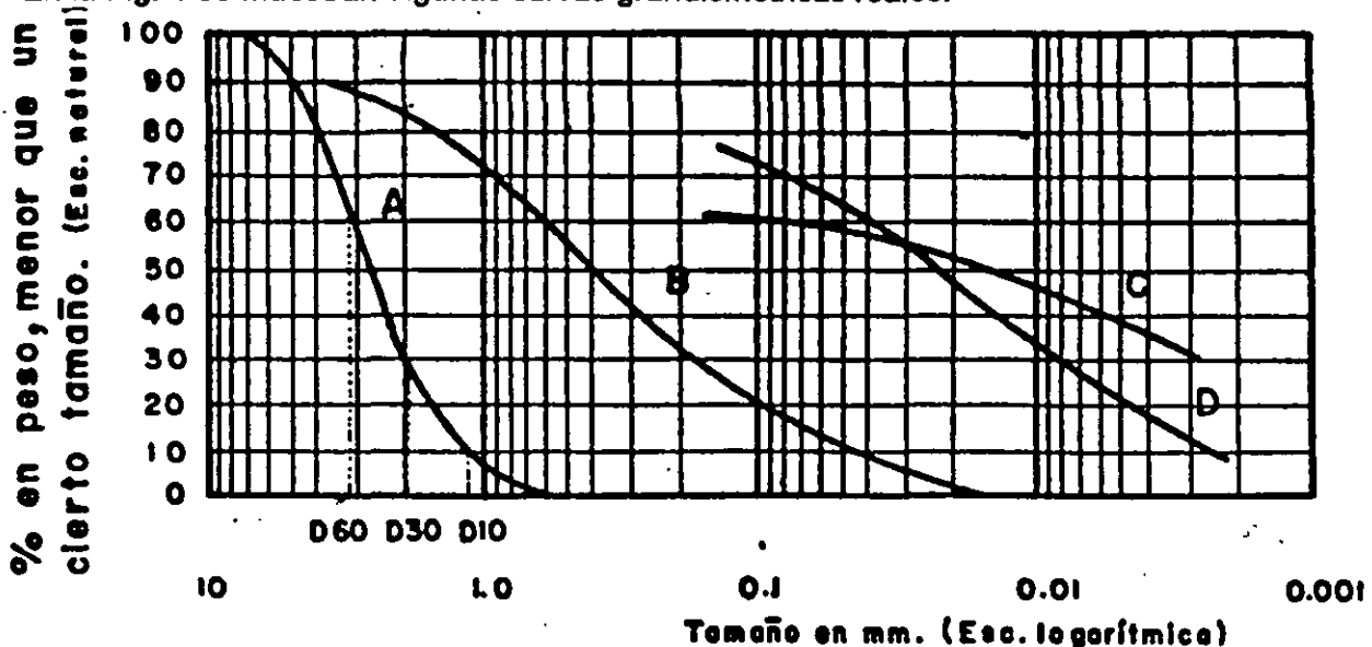
Figura 1. Curvas granulométricas de algunos suelos. A) Arena muy uniforme de Ciudad Cuauhtémoc, México. B) Suelo bien graduado, Puebla, México. C) Arcilla del Valle de México (curva obtenida con hidrómetro). D) Arcilla del Valle de México (curva obtenida con hidrómetro).
