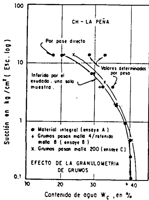
Fig 8. Ensayes de succión en un suelo fino activo [CH] (Ref. 1).
