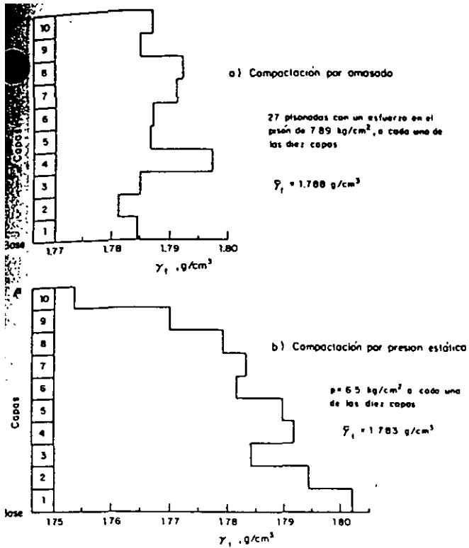
Fig. 12 Variación a través de la altura del peso volumétrico total de especímenes compactados por amasado y estáticamente. MH-Necaxa
