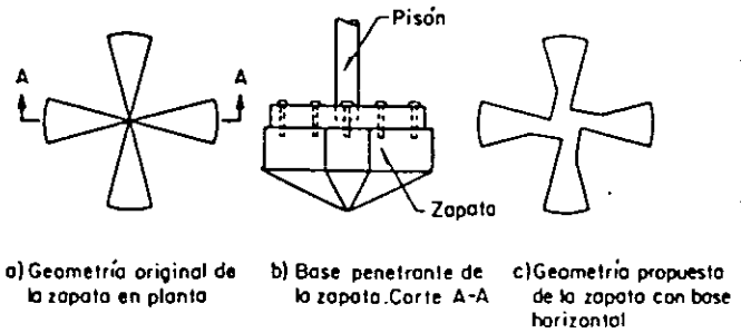
Fig. 13 Pisón de sectores para compactación por amasado
