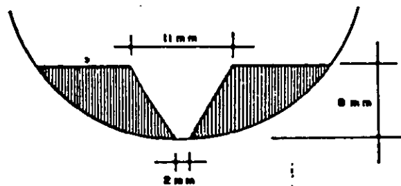
Figura 3 Dimensión de la ranura en la copa de Casagrande.
