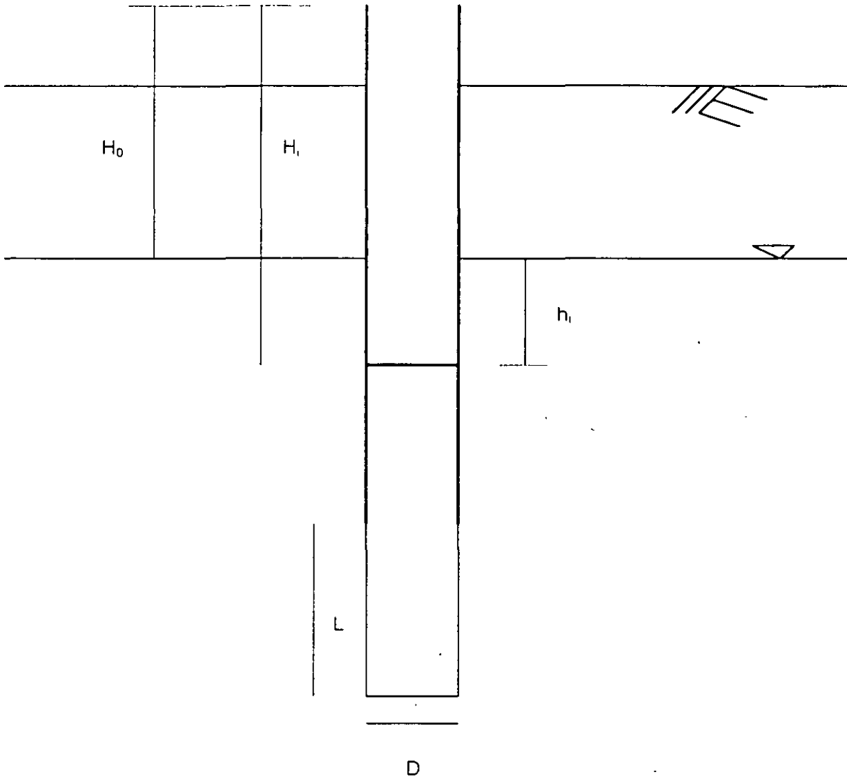
FIG. 56 PRUEBA LEFRANC DE EXTRACCION CON CARGA VARIABLE
