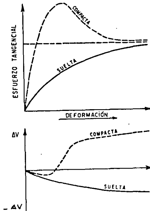
Figura 13 Diferencias de comportamiento entre una suelta y una compacta
