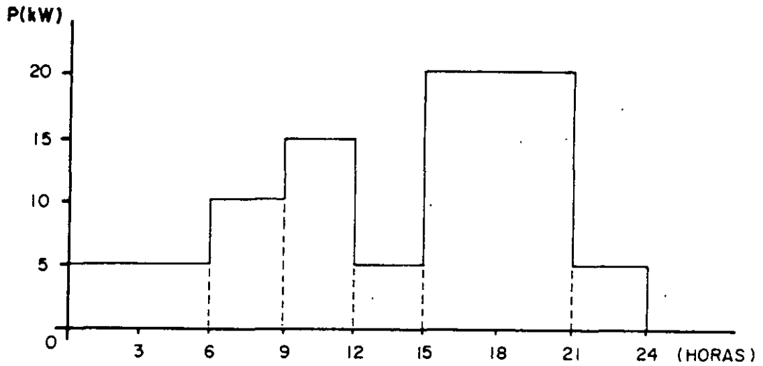
Figura 3.31 Curva de carga diaria.
