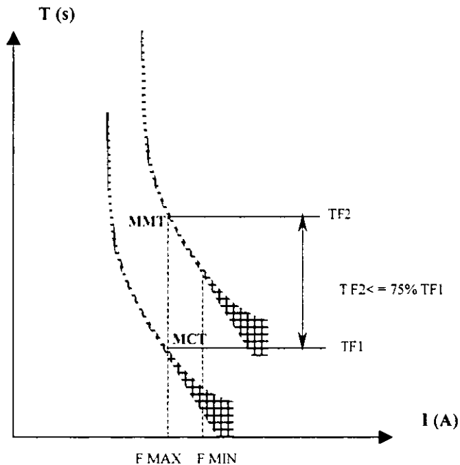
Figura 1-5 Coordinación Fusible–Fusible
