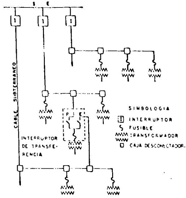
Fig.14 ESQUEMA DE PROTECCION DE UN ALIMENTADOR SUBTERRANEO
