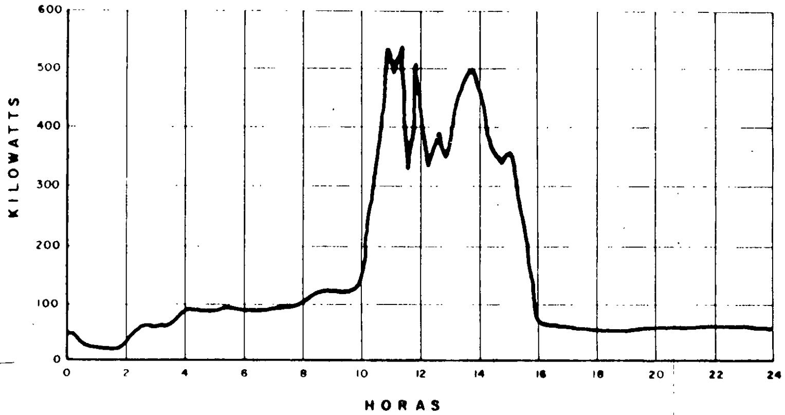
FIGURA 53 PERFIL DE DEMANDA (UN TURNO DE OPERACION)
