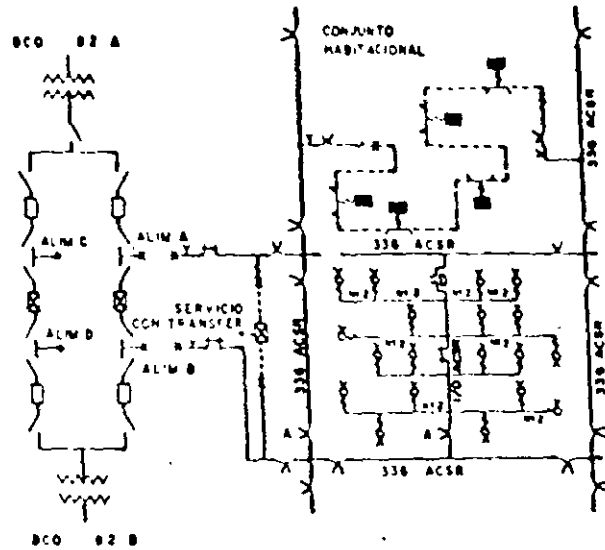
Fig 13 ESQUEMA DE PROTECCION DE UN ALIMENTADOR TIPO AEREO DE 23 KV
