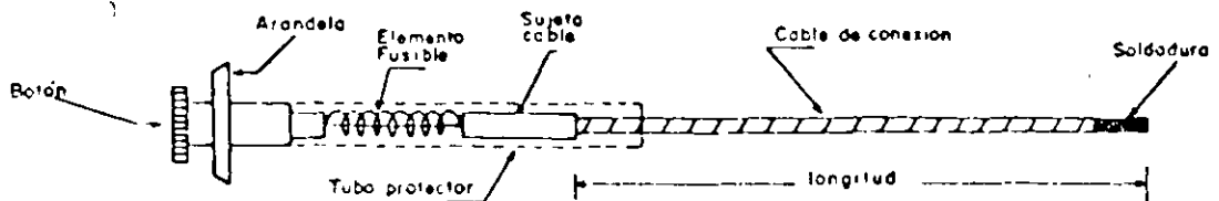
FIG. 4 Fusible de eslabón, tipo universal
