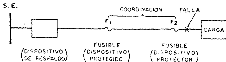
Fig 20 COORDINACION FUSIBLE-FUSIBLE
