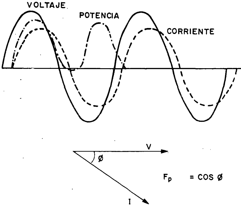
Figura 3.14 Factor de potencia.
