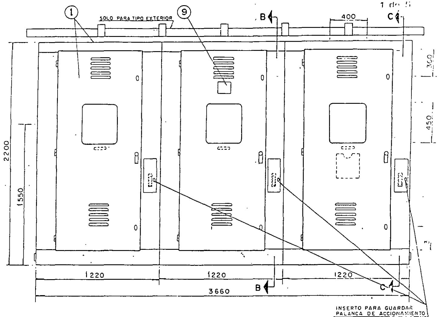
ELEVACION
