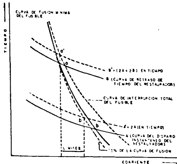
Fig 19 COORDINACION RESTAURADOR-FUSIBLE
