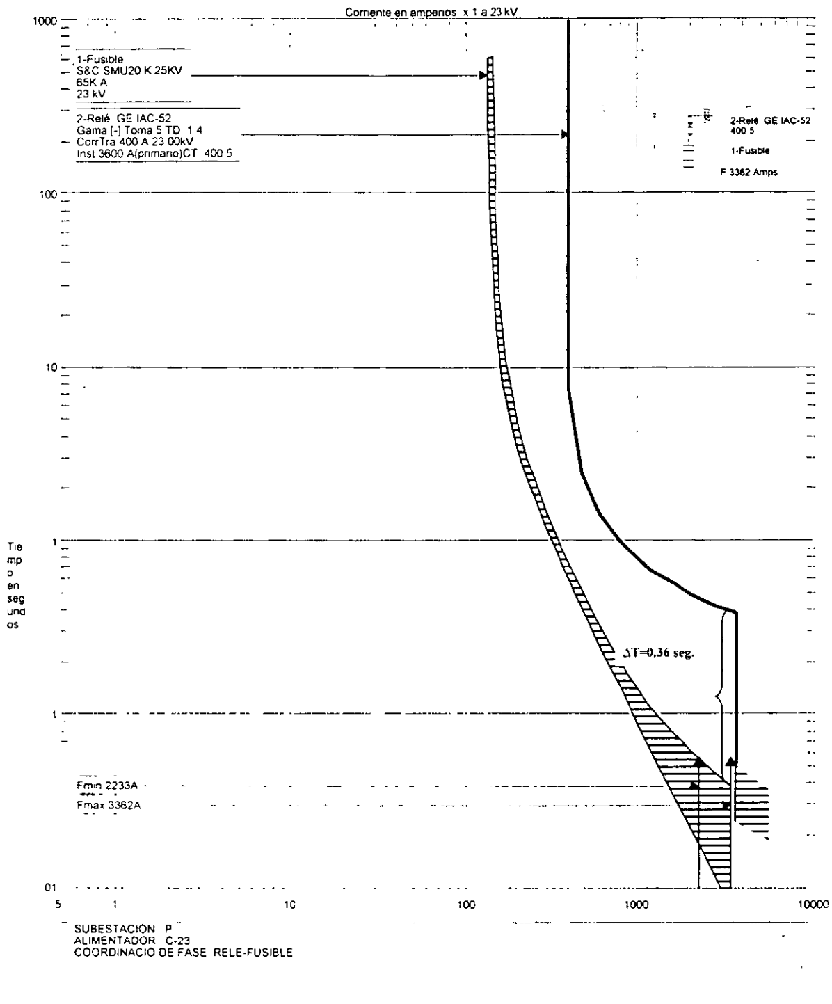
Gráfica 4-3 Coordinación de fase Relevador-fusible.
