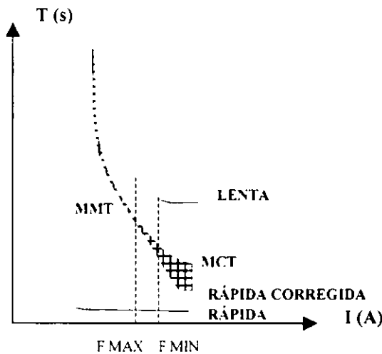
Figura 1-4 Coordinación Restaurador-Fusible
