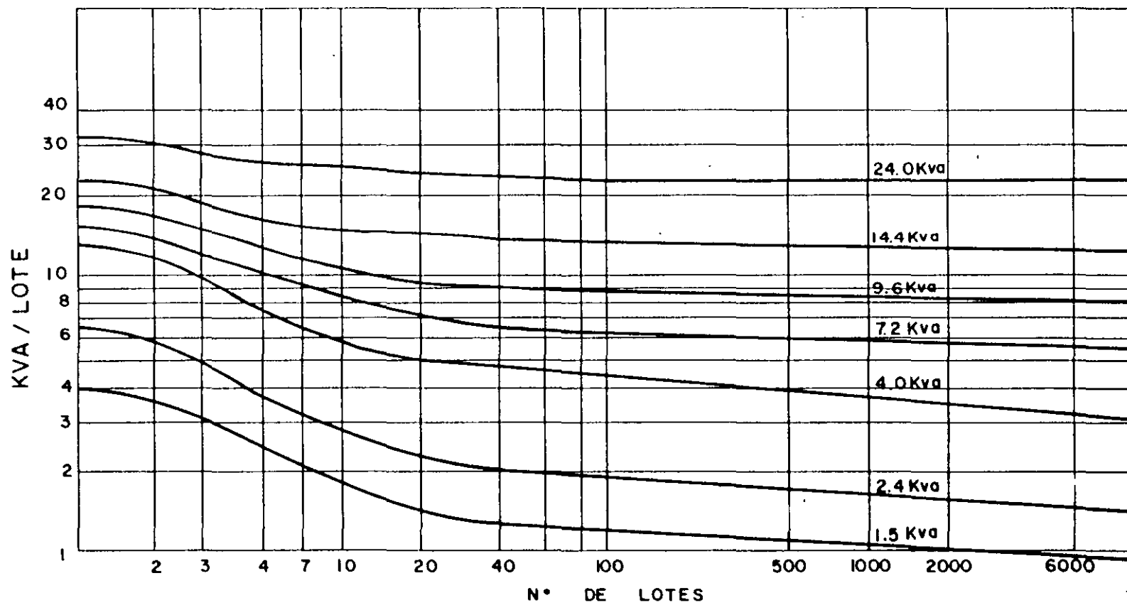
Figura 3.21 Máxima demanda diversificada probable para cargas residenciales.
