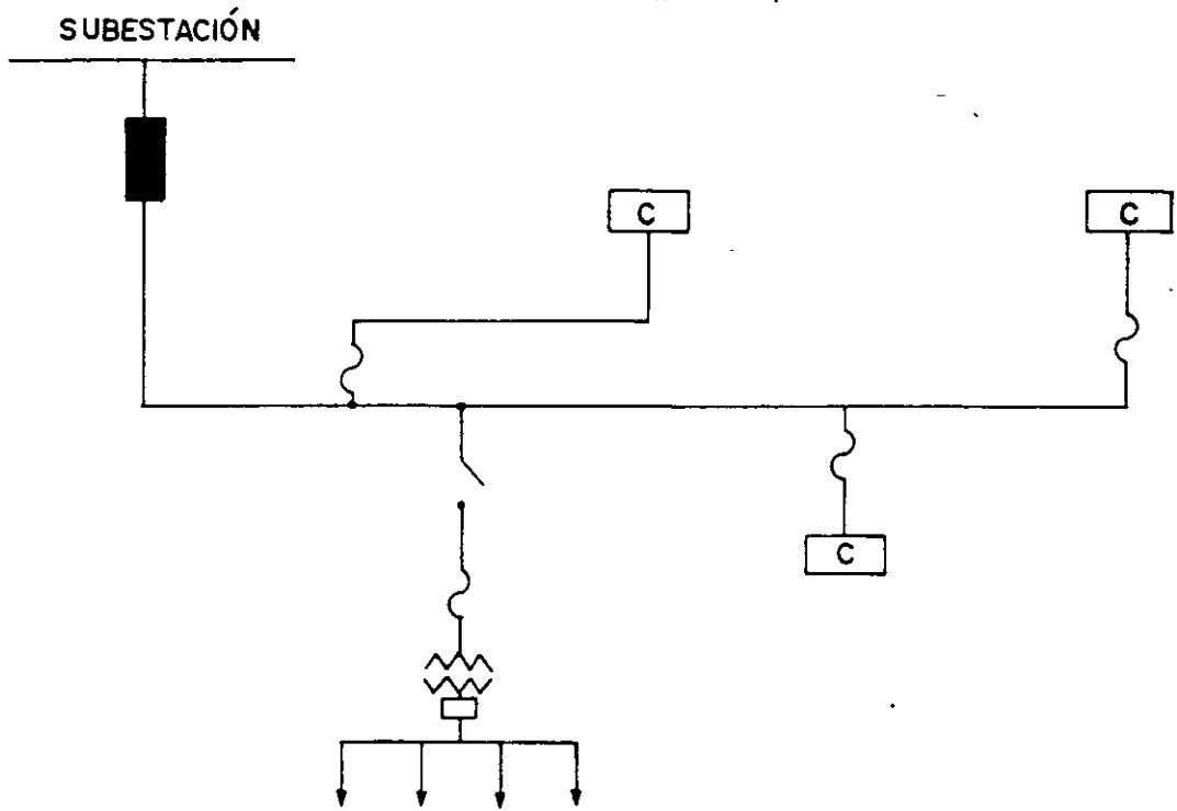
Figura 2.1 Red de operación radial sirviendo cargas en mediana y baja tensión.
