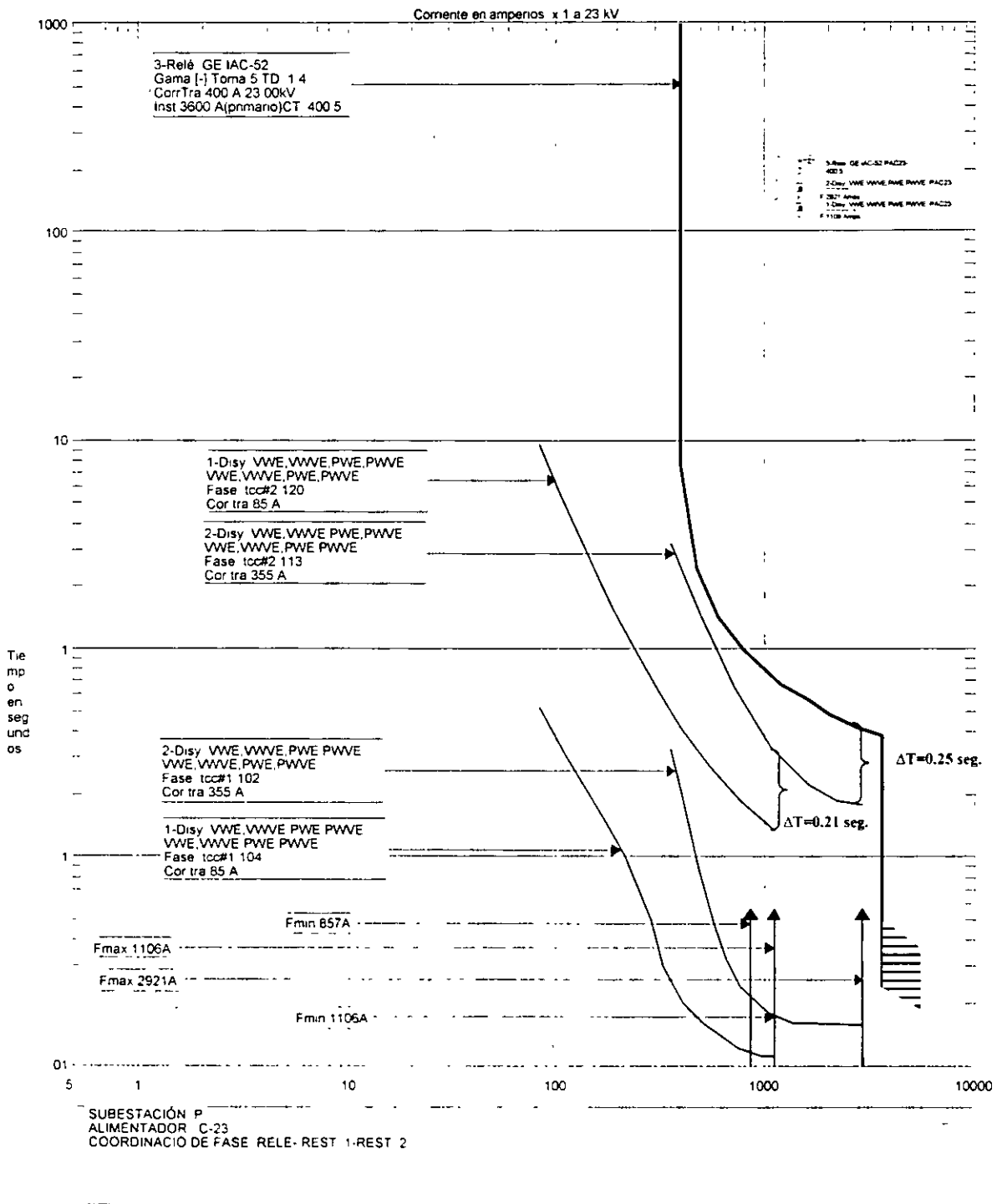
Gráfica 4-1. Coordinación de fase Relevador-Restauradores
