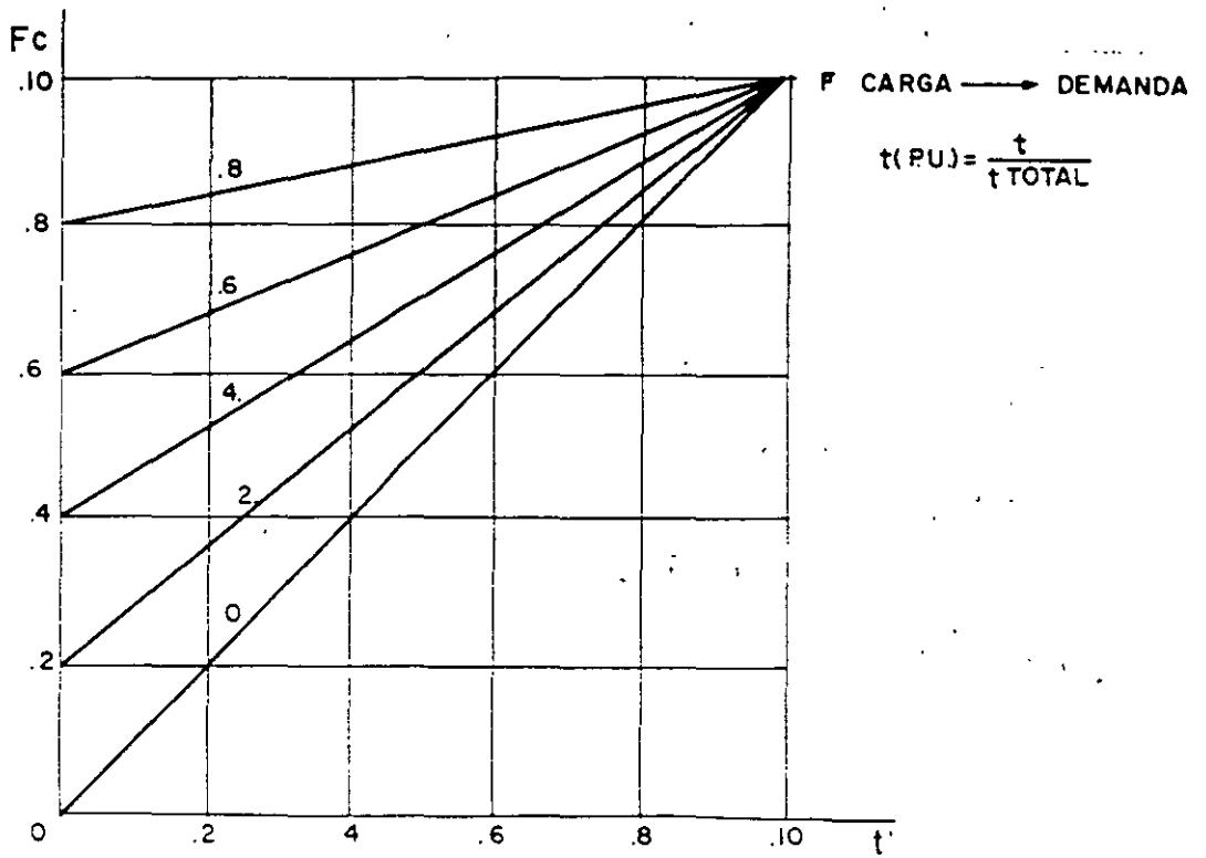
Figura 3.17 Relación entre F_c y t .
