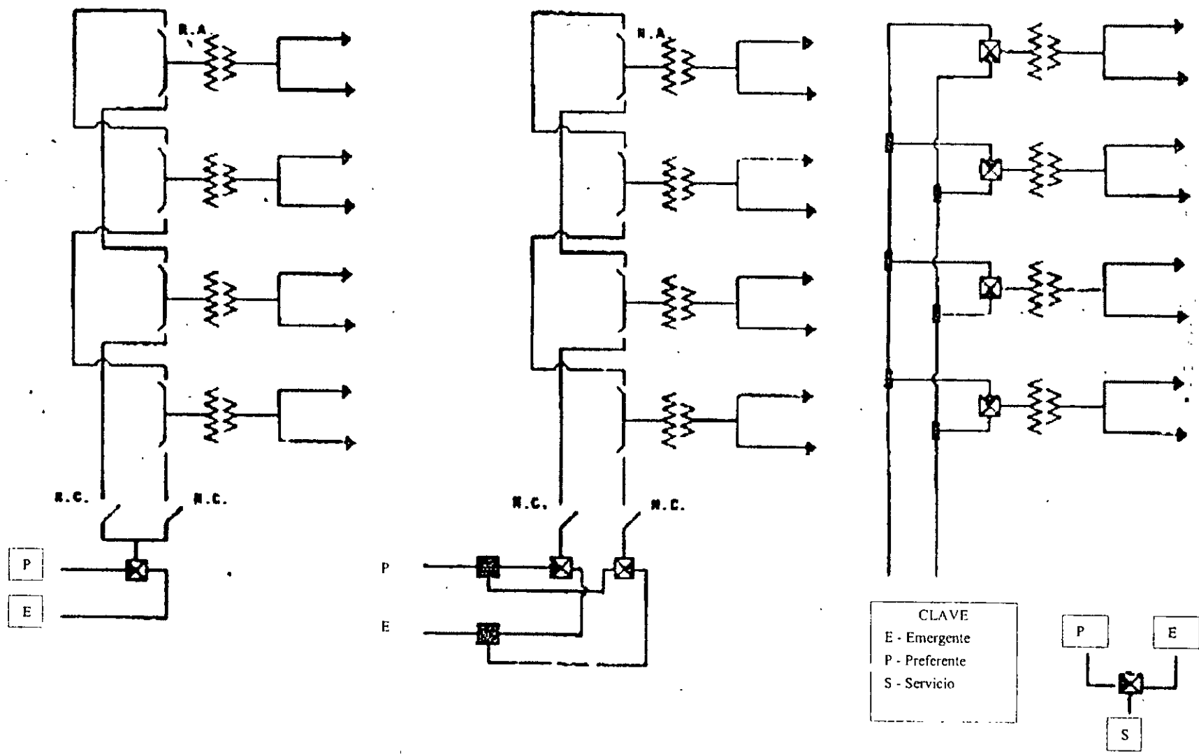
Figura 4.- Sistema en derivación doble para suministro de energía a edificios altos:
