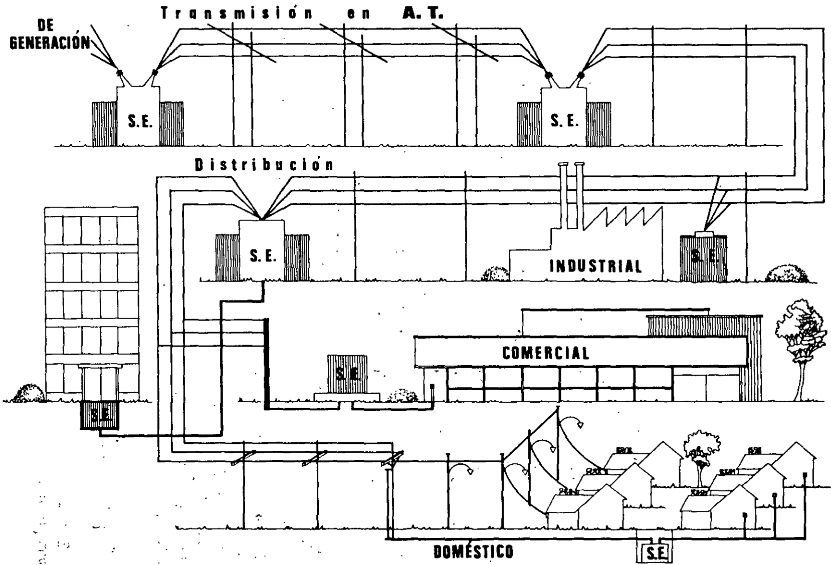
Figura 1.1 Sistema de distribución (aéreo y subterráneo).
