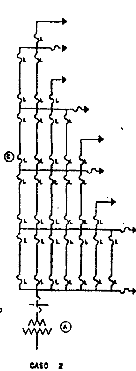
Figura 5.- Estructura de una mancha de red automática
