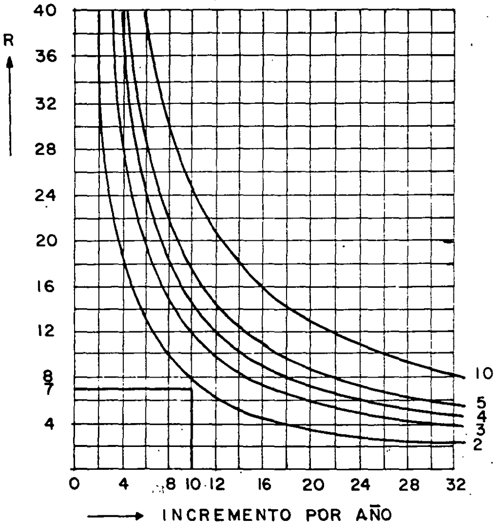
Figura 3.13 Tasa de crecimiento.
