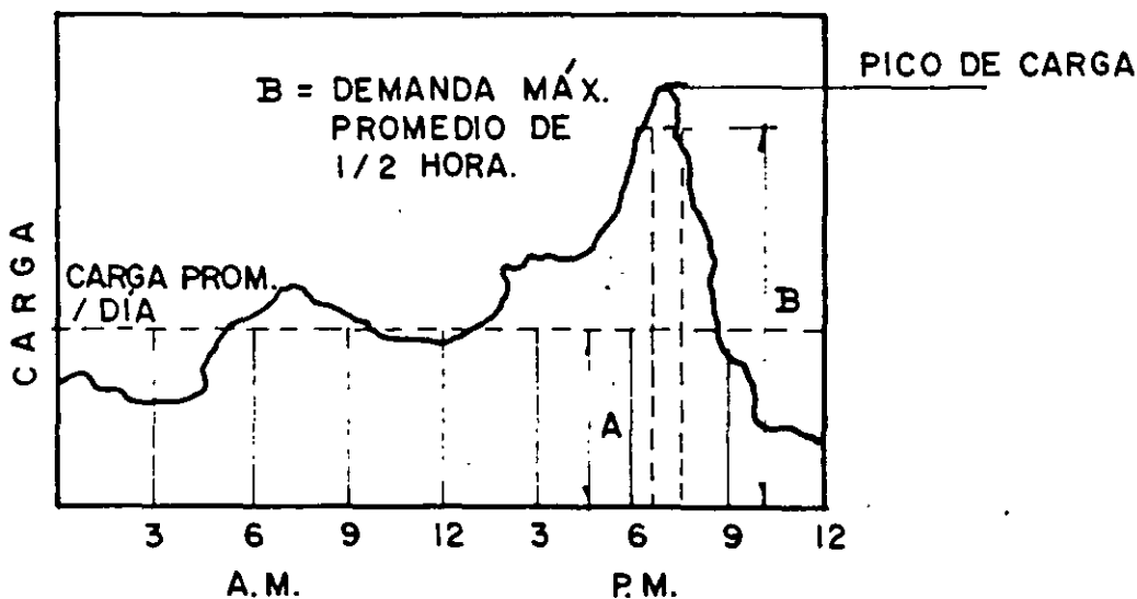
Figura 3.4 Factor de carga F_c .
