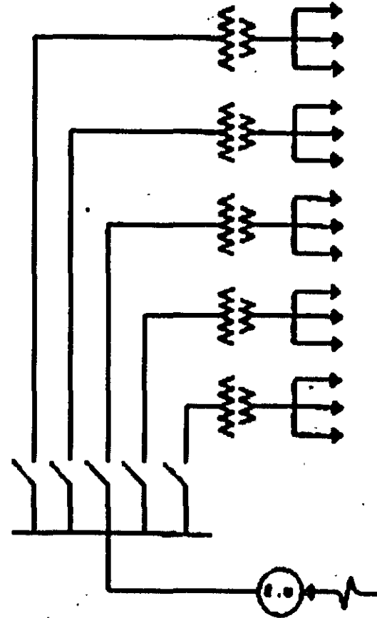
b) Un cable en S.T. con transformadores en varios niveles, alimentador radial, varios alimentadores.
