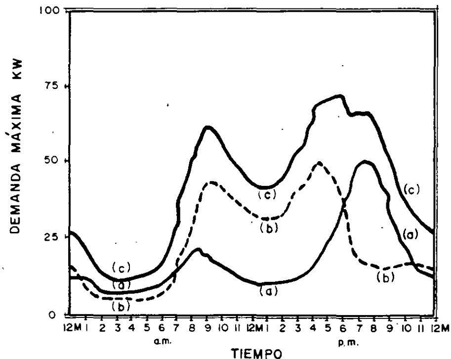
Figura 3.8 En cualquier instante la carga total c es igual a la suma de las cargas a y b . Debido a la diversidad, el máximo de la carga c será menor que la suma de los máximos de las cargas a y b .
