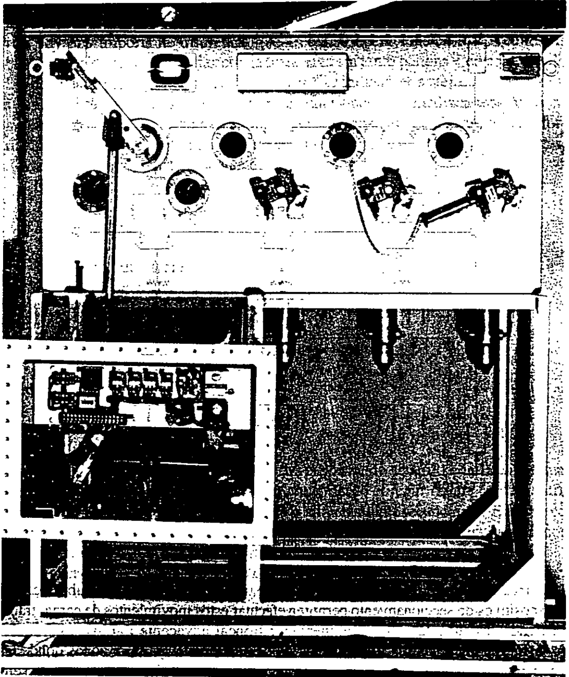
Figura 2.13 Interruptor de transferencia de carga.
