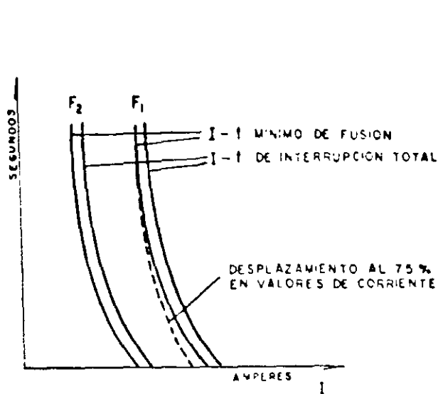
Fig.22 COORDINACION ENTRE F.L.C Y F.L.C.
