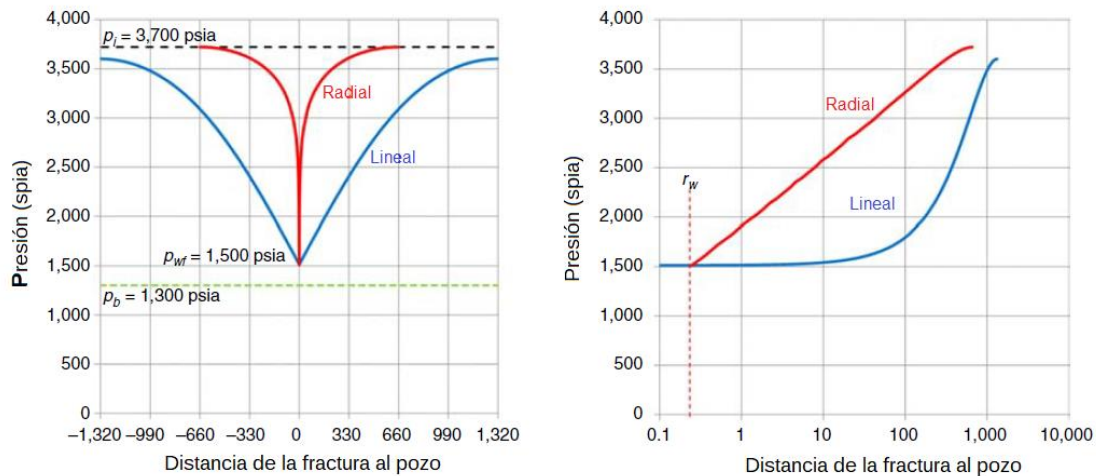
Fig. 36 Perfiles de presión simulados en un yacimiento de aceite de 5 mD con flujo monofásico después de producir 30 días a una P_{wf}=1,500 psia para un flujo radial y lineal. La gráfica de la derecha tiene una escala logarítmica en la distancia.
