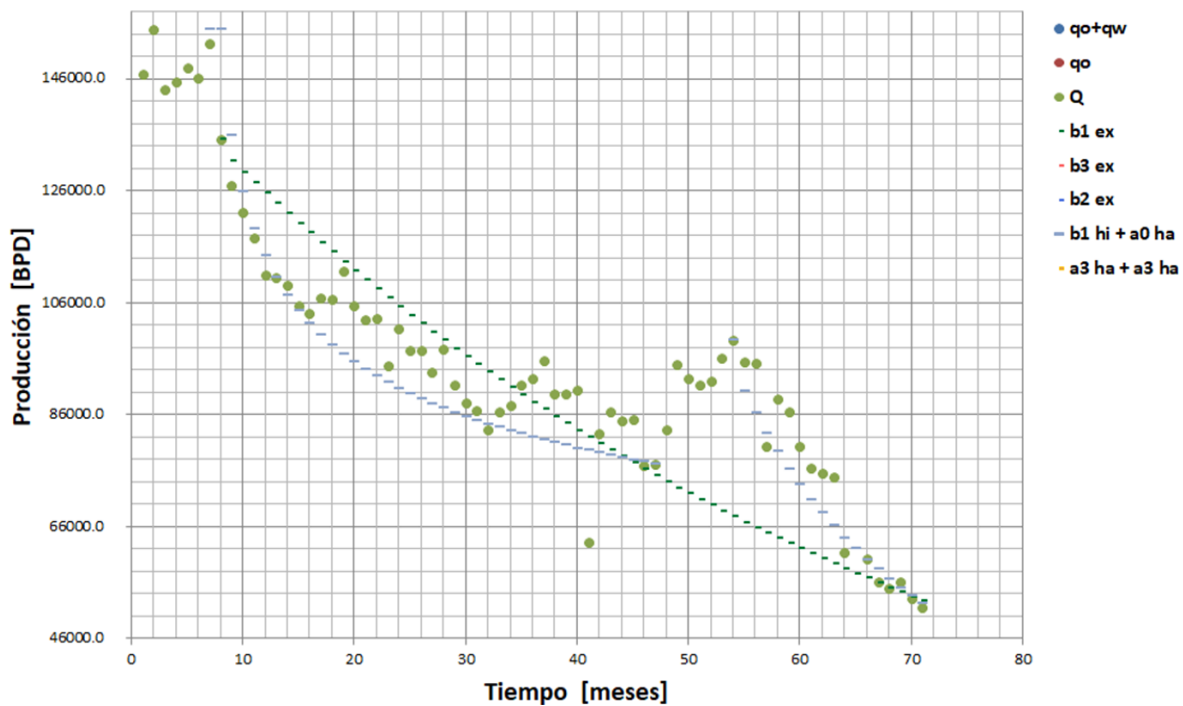
Fig. 48 Q vs t en escala normal con curvas de declinación ajustadas
