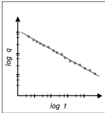
Fig. 45 Comportamiento típico de la declinación Hiperbólica grafica con escala logarítmica (New Mexico Tech, 2010)
