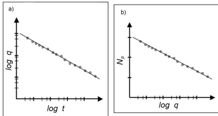
Fig. 46 Comportamiento típico de declinación armónica a) historial de producción escala logarítmica b) Producción acumulada gasto en escala logarítmica (Modificado de New Mexico Tech, 2010)
