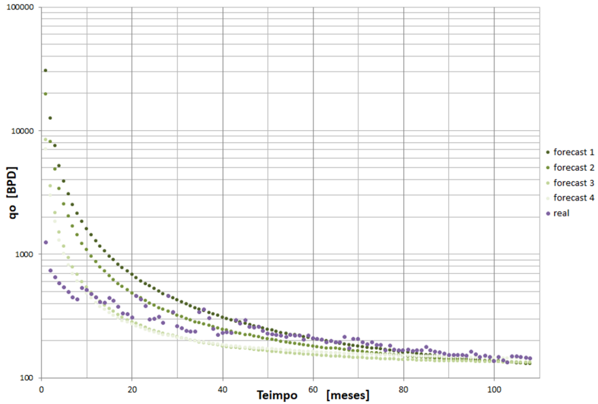
Fig. 57 Cuatro pronósticos de producción comparados contra el perfil de producción original. Se usa escala semilogarítmica para apreciar más fácil el ajuste.
