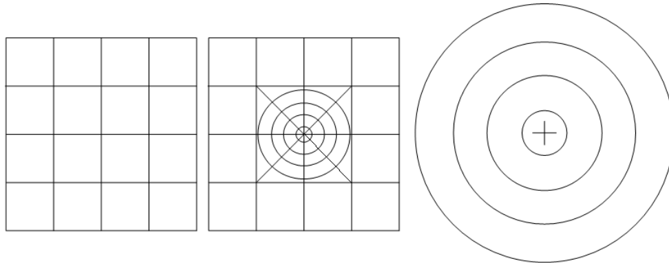
Fig. 29 Tipos de malla que pueden usarse para simular matemáticamente un yacimiento
