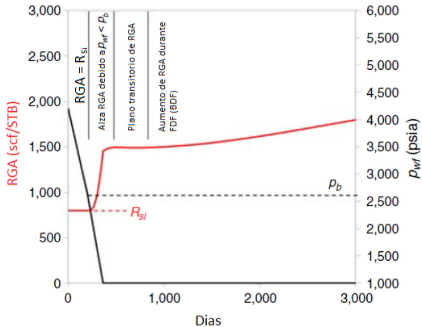
Fig. 35 Etapas de producción de un pozo horizontal con varias etapas de fracturamiento (modificado de Stevens J., 2016, pg.5)
