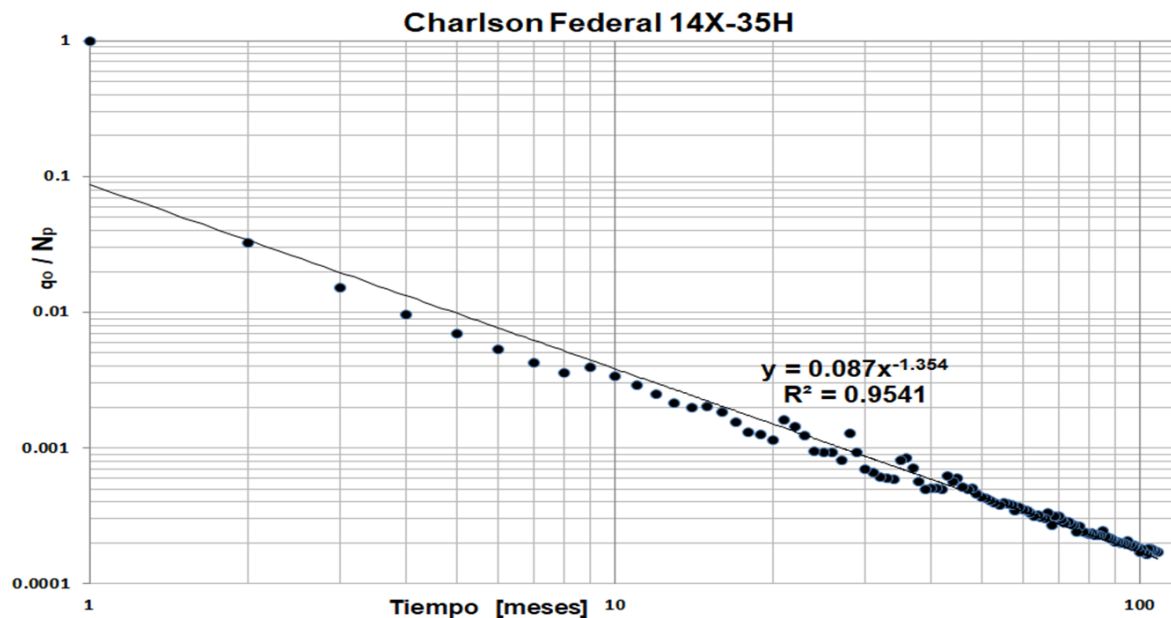
Fig. 55 Gráfica \log \frac{q_0}{N_p} vs \log t del pozo Charlson Federal 14X-35H para encontrar a y m .
