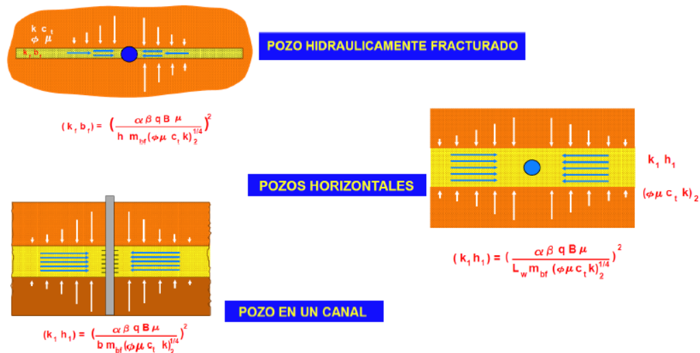
Fig. 24 Flujo Bilineal (Gallardo, 2015)
