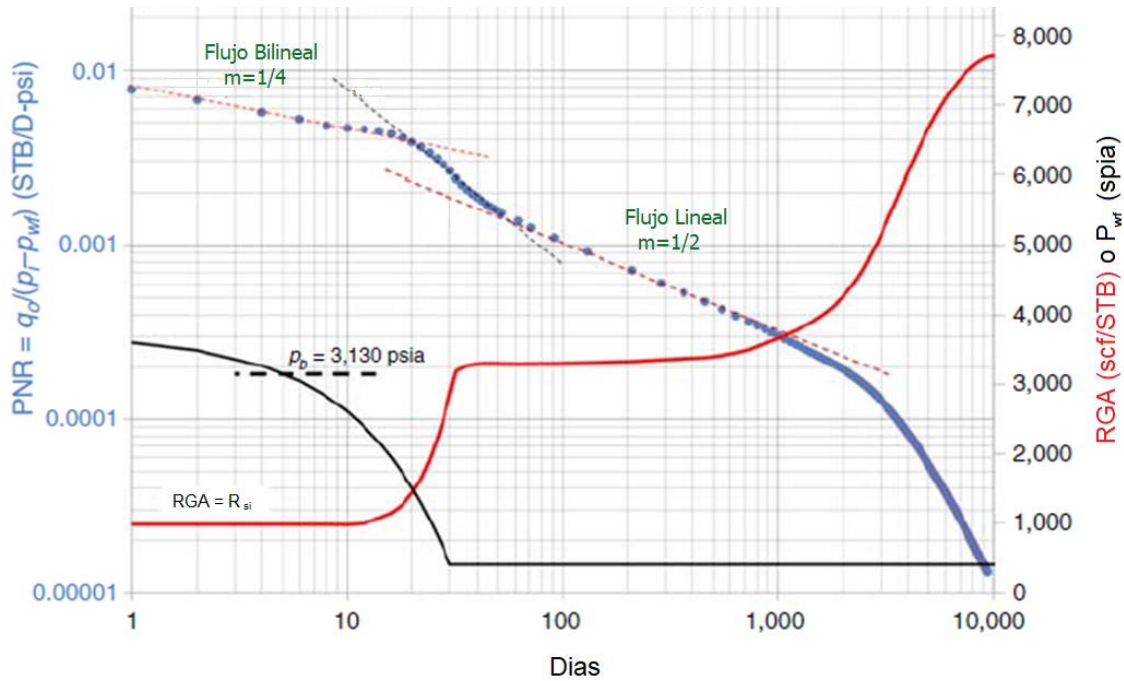
Fig. 37 Gráfica diagnóstica donde se pueden ver las geometrías presentes. Simulación de un caso con una fractura k=150 nd, x_f=240 ft, espaciamento de la fractura= 100 ft y k_f w_f=8 md-ft. Pressure normalized Oil Ratio, PNR = \frac{q_o}{P_i - P_{wf}} . (modificado de Stevens, 2016)
