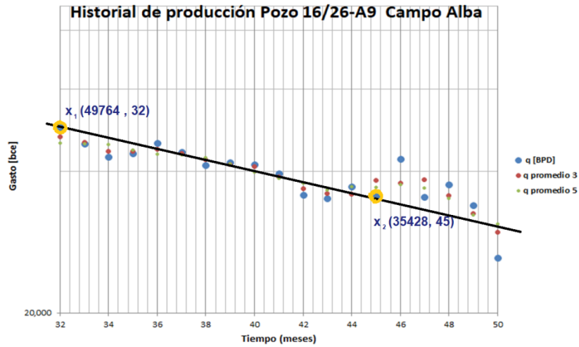
Fig. 43 Sección del historial de producción de pozo 16/26 A9 con línea de tendencia para ejemplificar como obtener el coeficiente b
