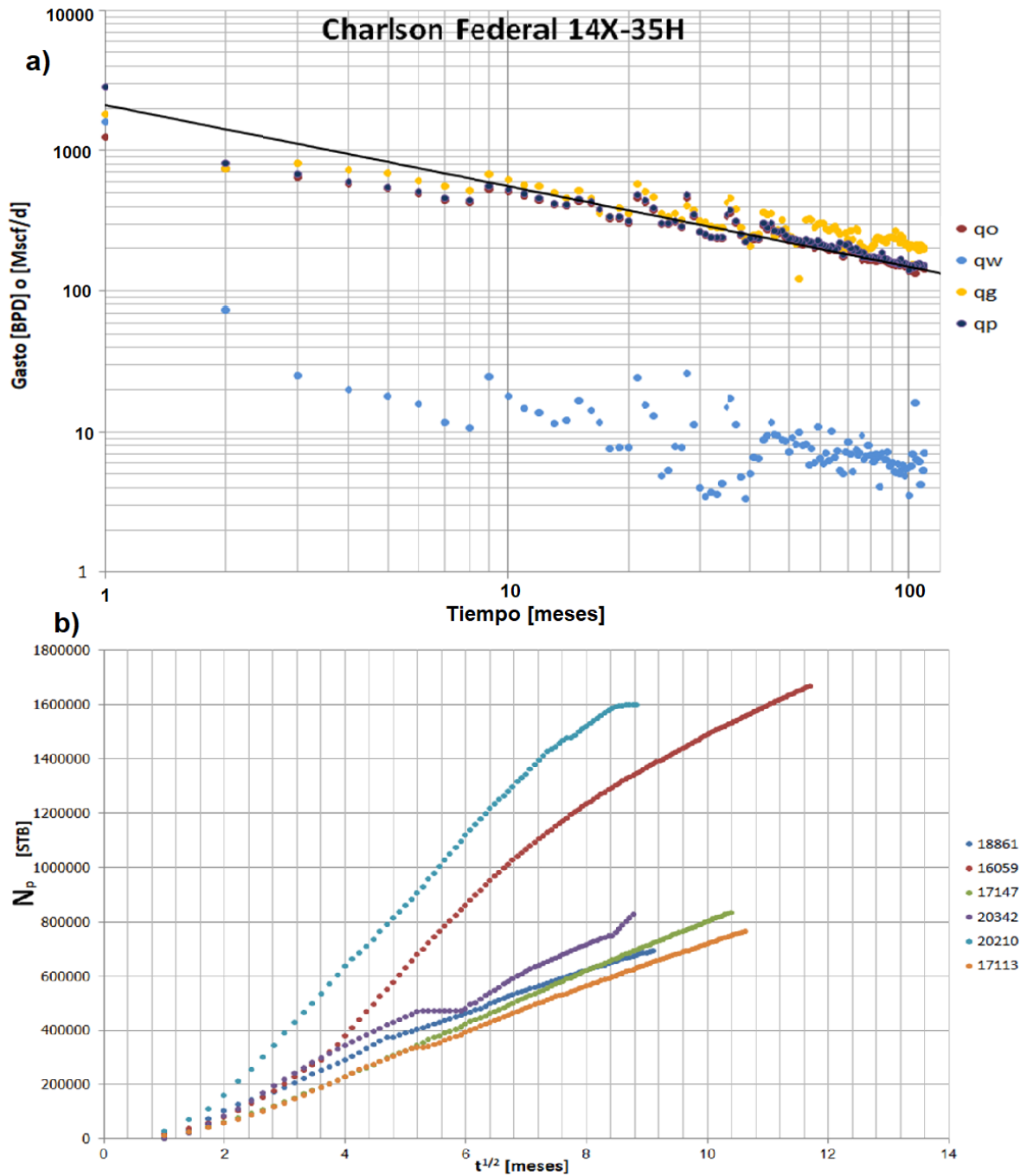
Fig. 53 a) \log\{q_o, q_w, q_g, q_p(q_o + q_w)\} vs \log t con una pendiente de \frac{1}{4} que es característico de flujo lineal de pozo Charlson Federal 14X-35H. b) N_p vs t^{1/2} usada para ver que pozos producen en flujo lineal y en el periodos de tiempo. 18861 (Carson Peak 2-35H), 16059 (USA 2D-3-1H), 17147 (Boucher 41X-21), 20342(USA 153-95-4B-9-1H), 20210 (Whitman 2-3H), 17113 (Charlson Federal 14X-35H). (MDND, 2018)
