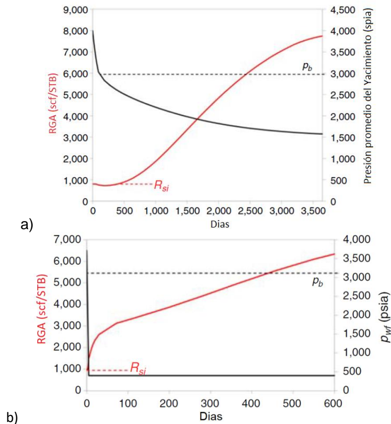
Fig. 32 a) Comportamiento de RGA vs \bar{P} yacimiento convencional con un pozo vertical sin fracturar, b) Comportamiento de un yacimiento no convencional con pozo horizontal fracturado (Stevens, 2016)
