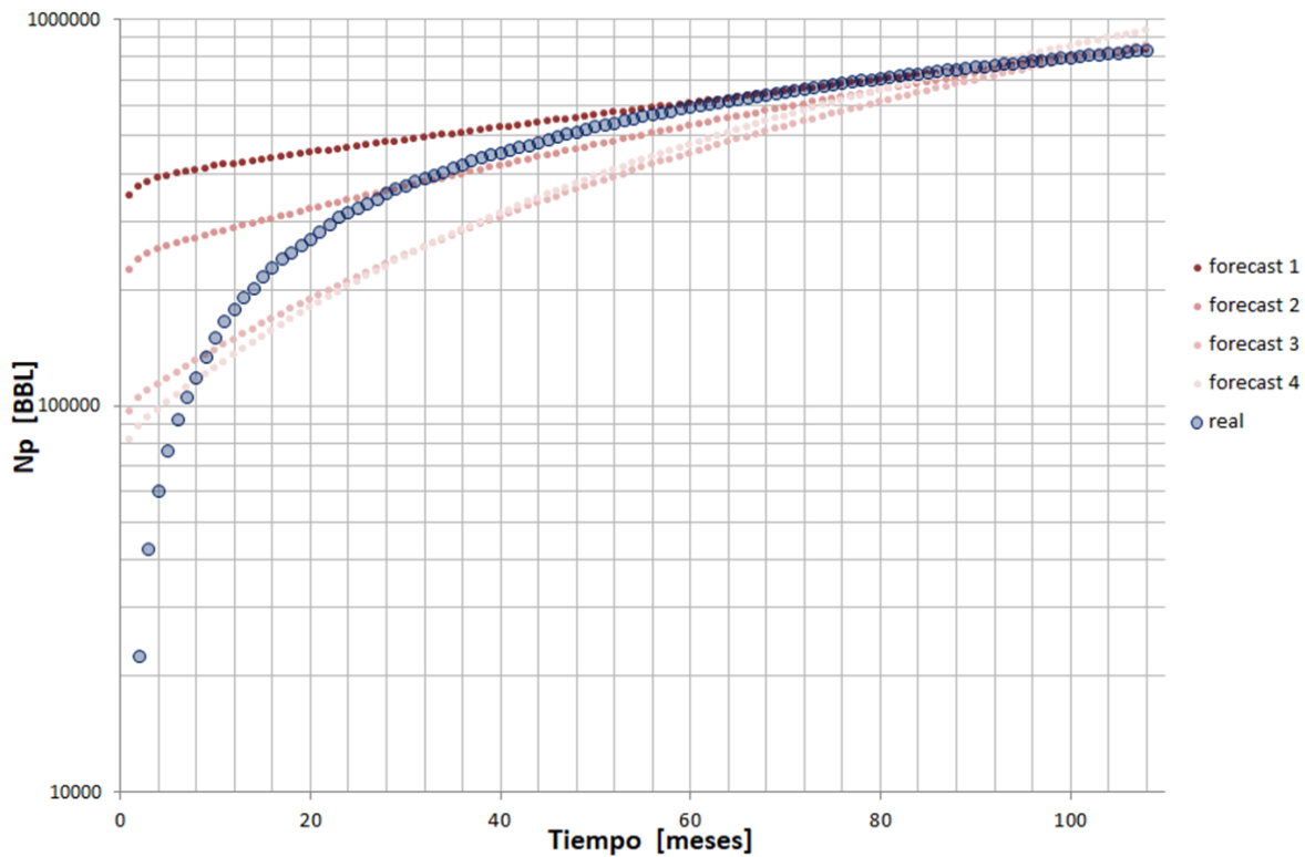
Fig. 58 Estimación de reservas usando los cuatro pronósticos de producción determinados con el método de Duong.
