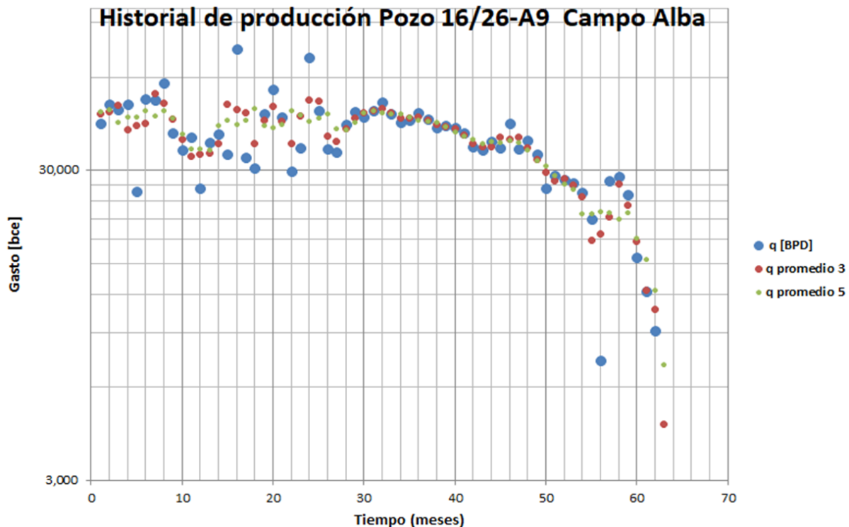
Fig. 41 Historial del producción del Pozo 16/26 A9. Se grafica la producción normal y el promedio de 3 puntos y puntos para poder ajustar mejor una línea de tendencia. Para más información consultar el anexo B para saber cómo se llegó a la gráfica.
