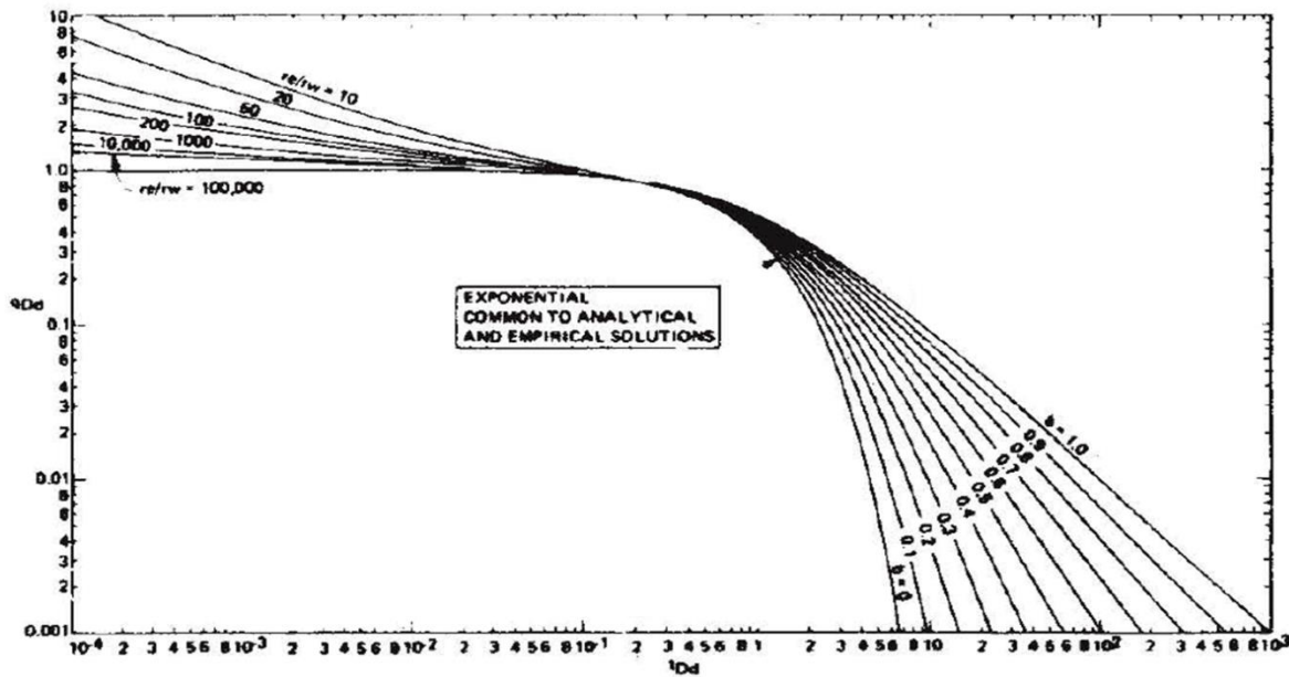
Fig. 51 Familia de curvas tipo graficadas en escala logarítmica. (Modificado de Fetkovich. 1980)
