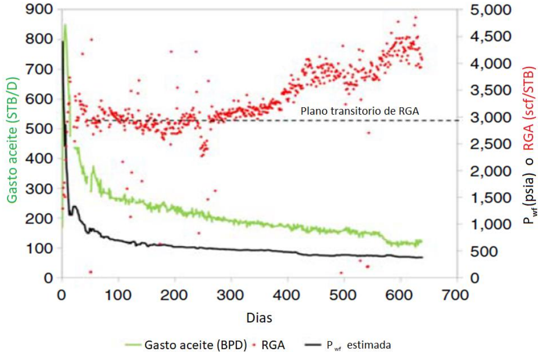
Fig. 34 Historial de producción de un pozo tipo tight oil de la formación Meramec de la cuenca Anadarko. (Modificado de Stevens, 2016).
