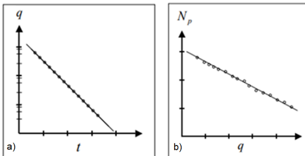
Fig. 42 Comportamiento típico de la declinación exponencial a) en gráfica semilogarítmica q vs t b) gráfica de producción acumulada escala normal (New Nexico Tech, 2010)
