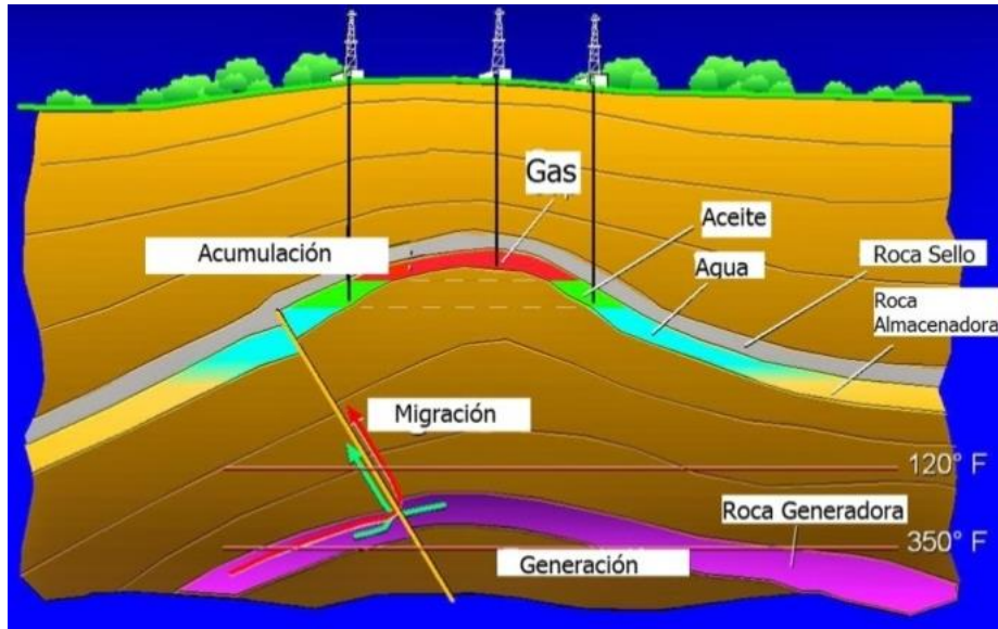
Fig. 5 Sistema Petrolero Convencional
