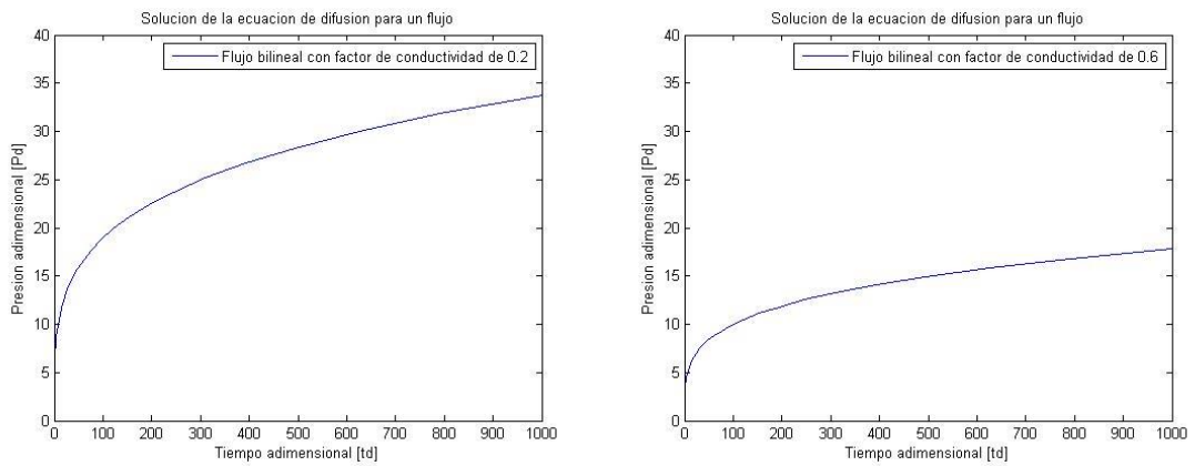
Fig. 25 Comportamiento del Flujo Bilineal en variables adimensionales con un Factor de Conductividad de 0.2 y 0.6
