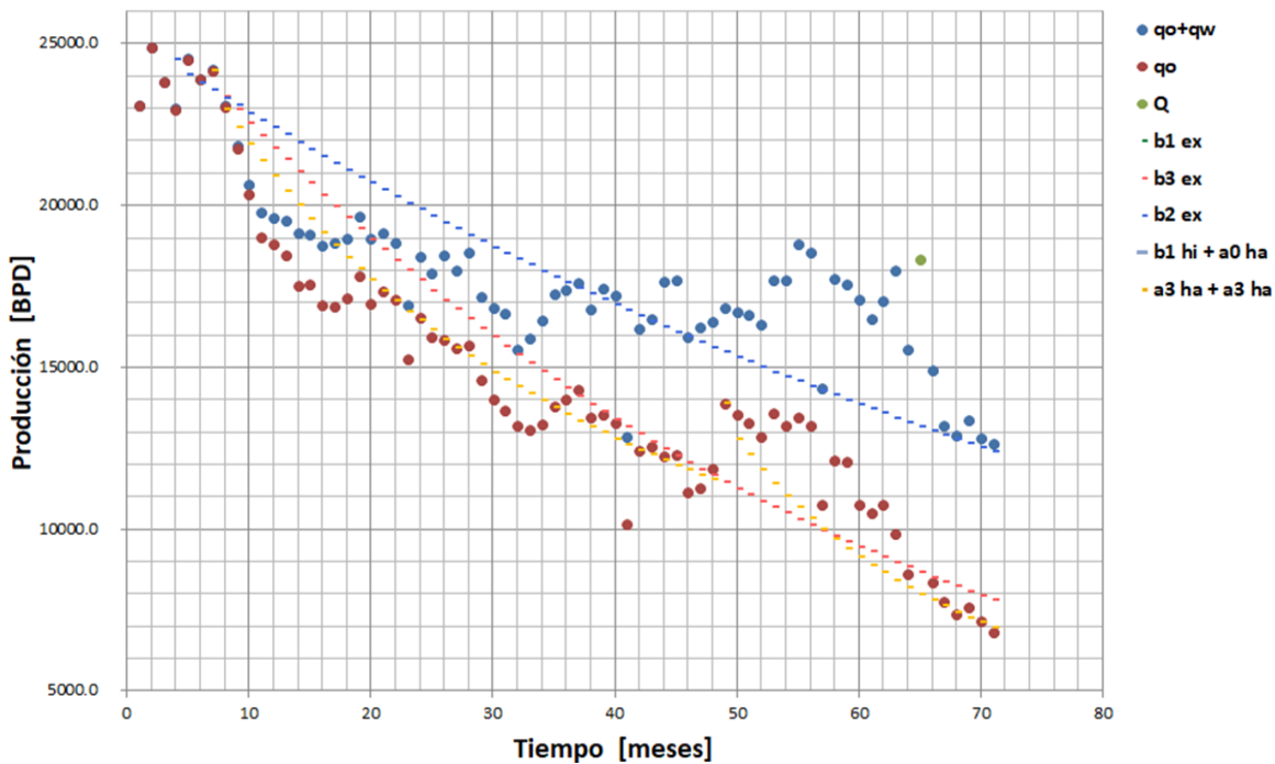
Fig. 49 q_o+q_w y q_o vs t en escala normal con curvas de declinación ajustadas
