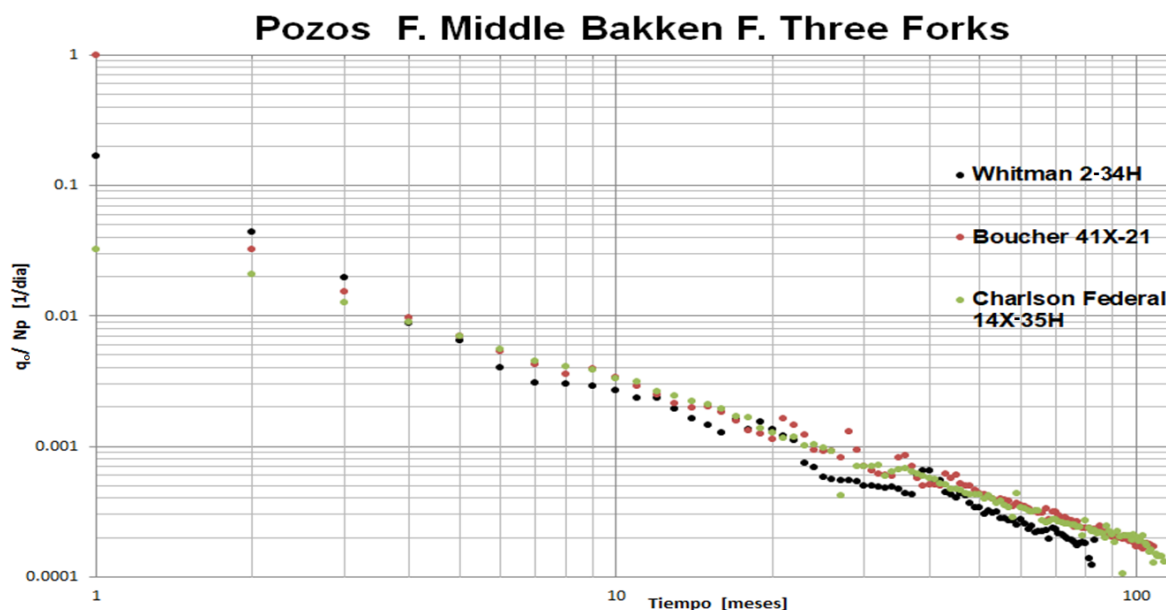
Fig. 52 Gráfica de \log \frac{q_o}{N_p} vs \log t de los pozos Whitman (F. M. Bakken), Boucher (F. Three Forks) y Charlson (F. Three Forks) . (MDND, 2018)
