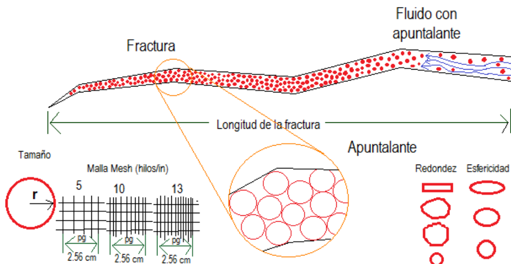
Fig. 2 Fractura y características del apuntalante
