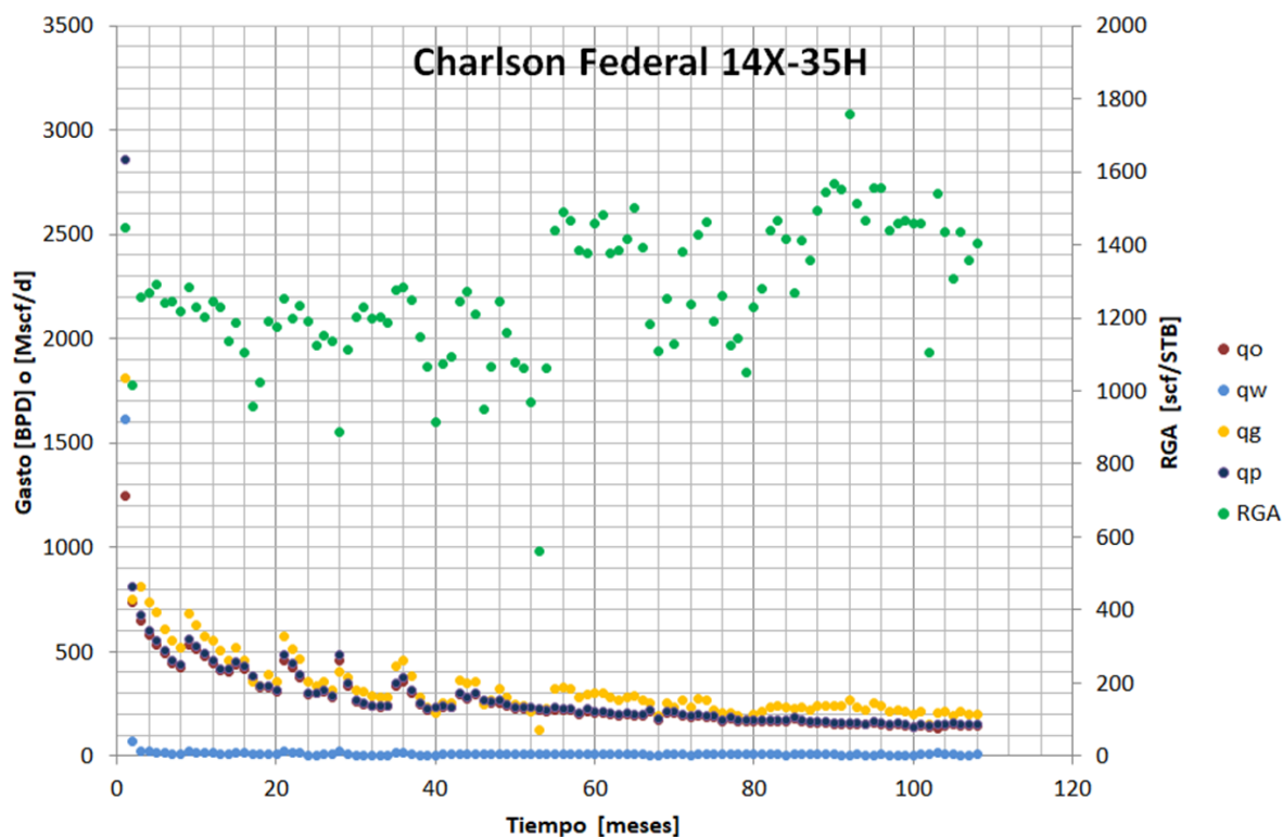
Fig. 54 Historial de producción del pozo Charlson Federal 14X-35H para usarse como ejemplo. (MDND, 2018)
