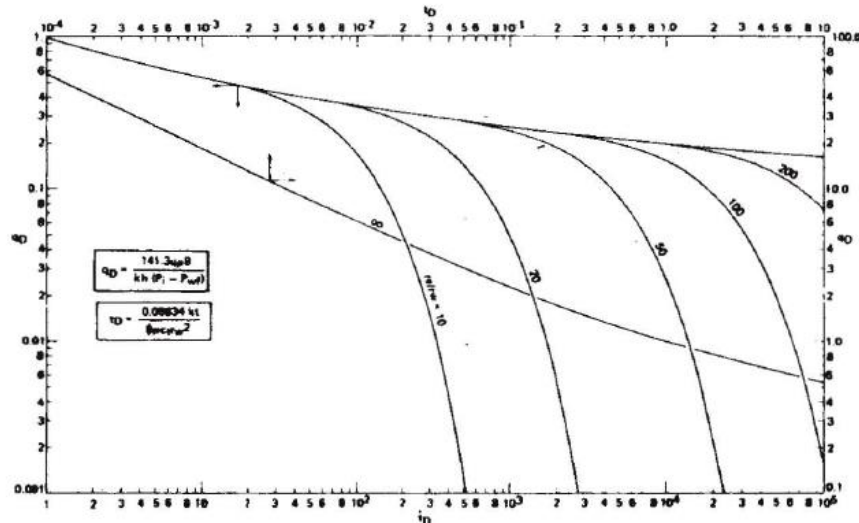
Fig. 50 Efecto del radio de drenaje en la duración del régimen transitorio de las curvas tipo (Fetkovich, 1980)
