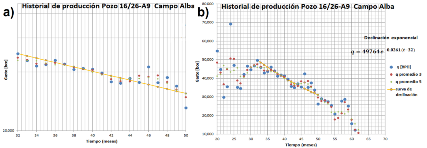
Fig. 44 a) Historial de producción en escala semilogarítmica con curva de declinación ajustada b) historial de producción en escala normal con curva de declinación ajustada
