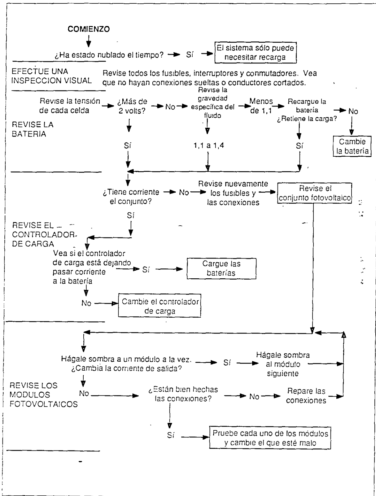
Figura 22. Guía de localización de fallas.
