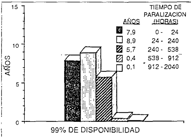
Figura 7. Tiempo de paralización anual (99%).
