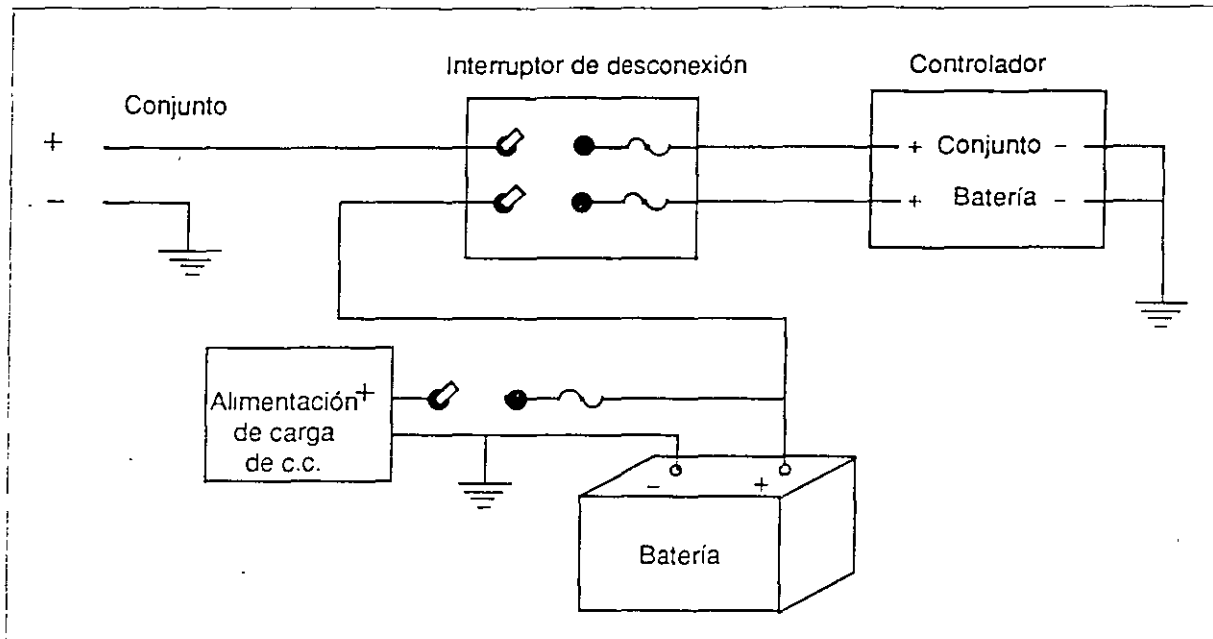
Figura 12. Alambrado del interruptor de desconexión con fusibles.
