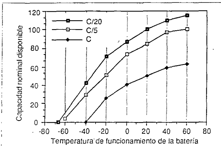
Figure 5. Capacidad en función de la temperatura de una batería de plomo-ácido.
