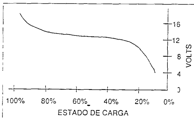
Figura 15. Curva del estado de carga de una batería típica de 12 V.
