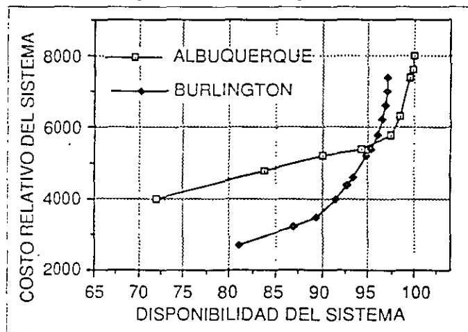
Figura 8. Costo en función de la disponibilidad Albuquerque, Nuevo México y Burlington, Vermont.
