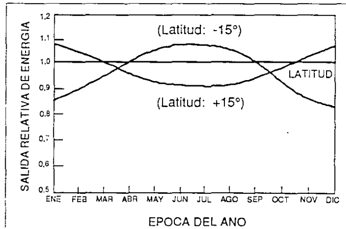
Figure 13. Efecto del ángulo de inclinación del conjunto sobre la producción anual de energía.
