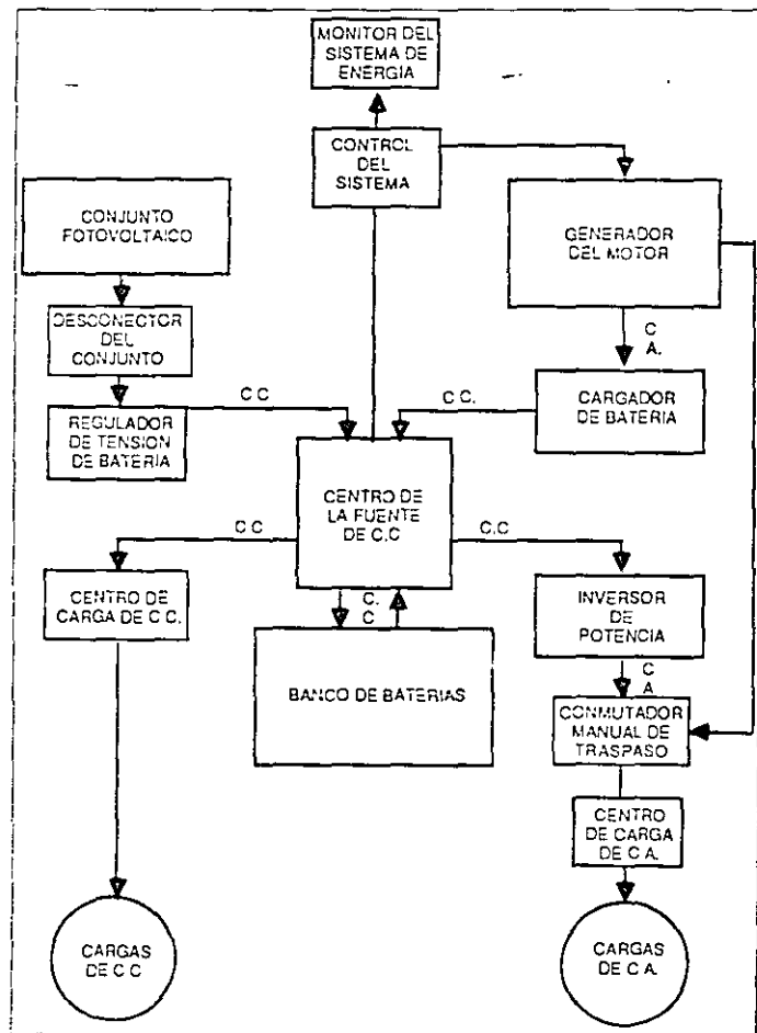
Figura 24. Esquema simplificado de la configuración de un sistema fotovoltaico híbrido.
