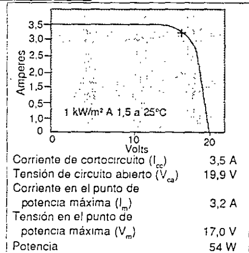
Figura 9. Especificaciones de un módulo fotovoltaico.
