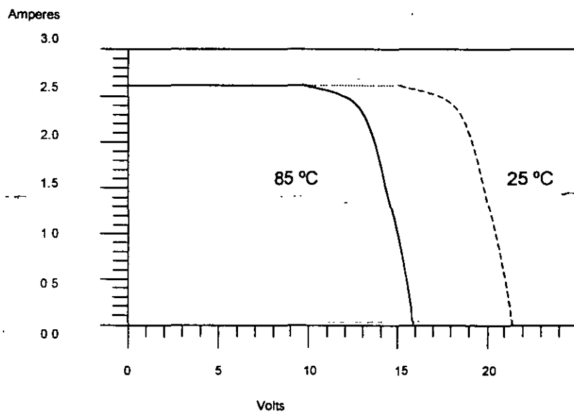
Figura 3.- Curva Típica Corriente - Voltaje de un módulo fotovoltaico a 25 y a 85 °C
