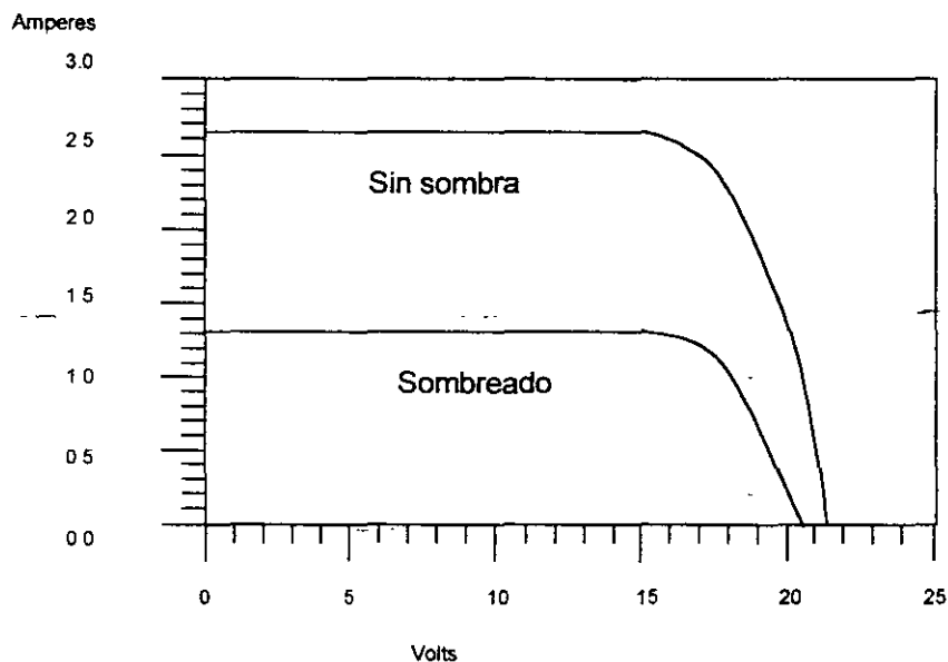
Figura 4.- Curva Típica Corriente.- Voltaje de un modulo fotovoltaico sin sombra y un módulo con una celda sombreada
