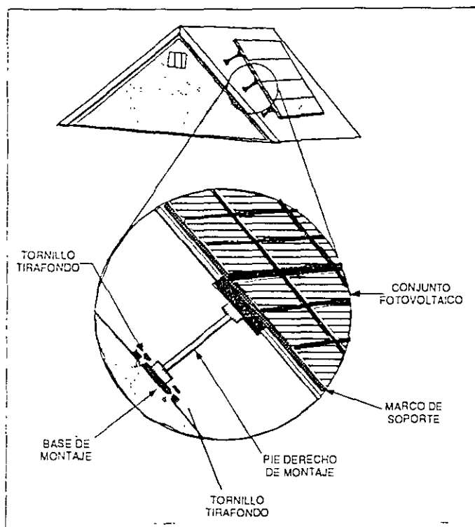
Figura 21. Conjunto fotovoltaico de montaje en el techo.
