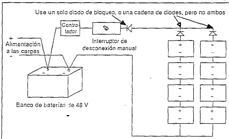
Figura 11. Conjunto de 48 V con el uso de diodo de bloqueo.
