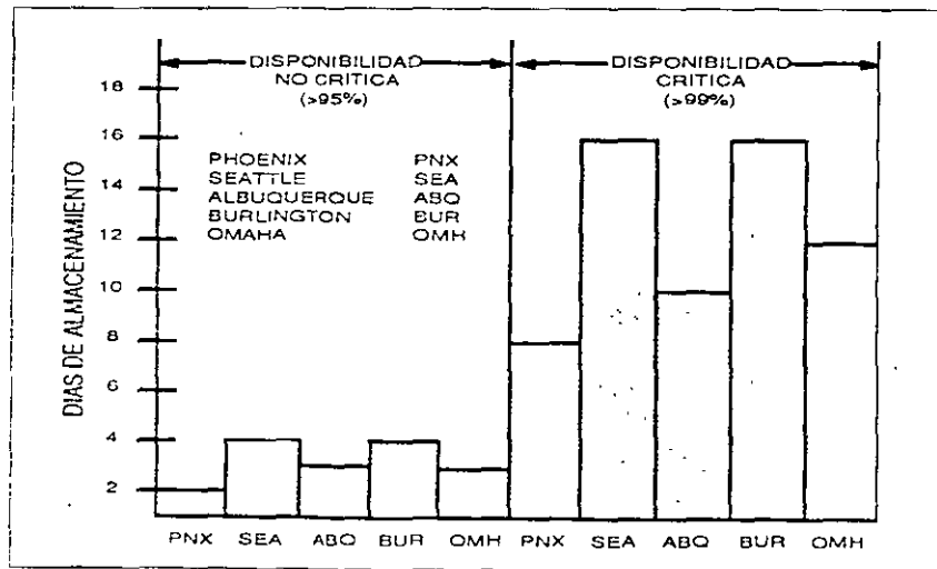
Figura 4. Días de almacenamiento para cinco ciudades.
