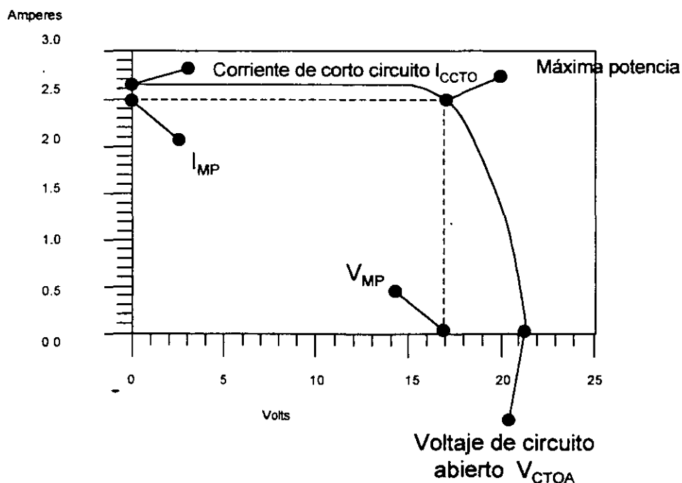
Figura 1.- Curva Típica Corriente - Voltaje de un modulo fotovoltaico
