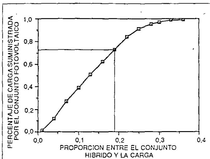
Figura 26. Curva del conjunto fotovoltaico-generador para Omaha.
