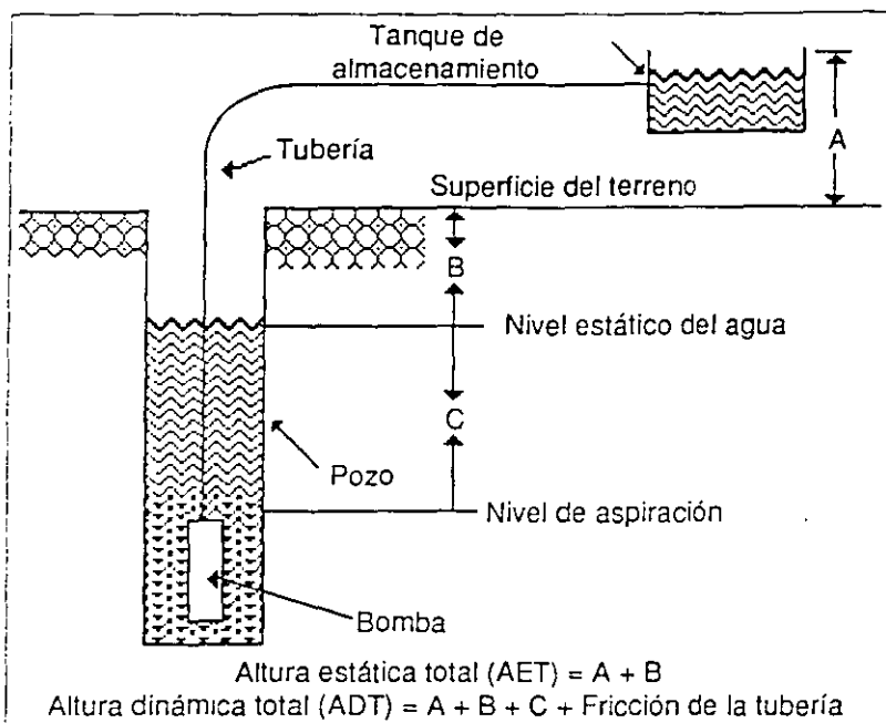
Figura 23. Términos de sistemas de bombeo.
