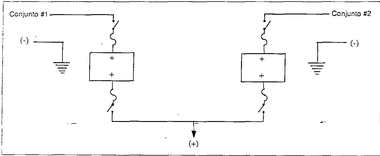
Figura 16. Conexión en paralelo de dos controladores.
