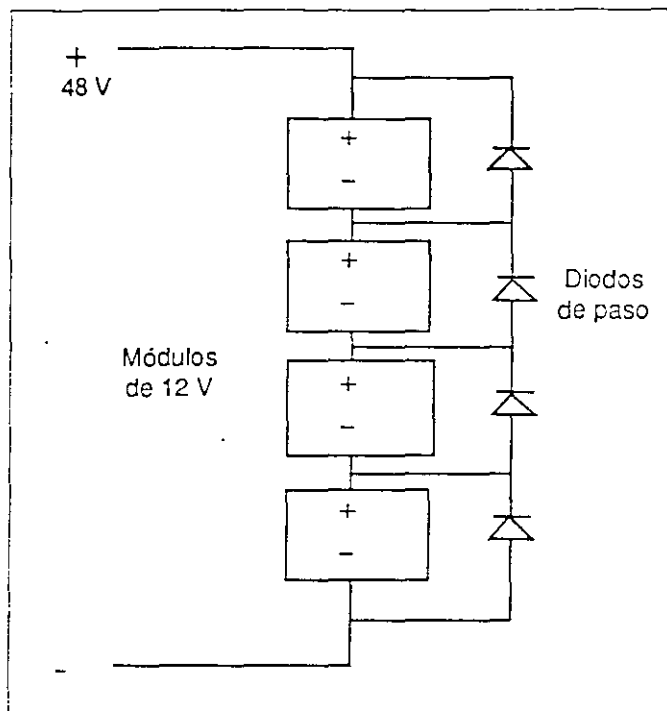
Figura 10. Cadena en serie con diodos de paso.
