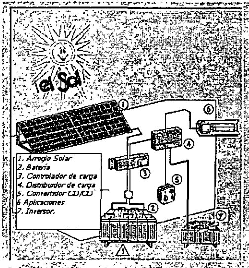
Fig 1.1. Componentes de un sistema fotovoltaico aislado de baja potencia.
