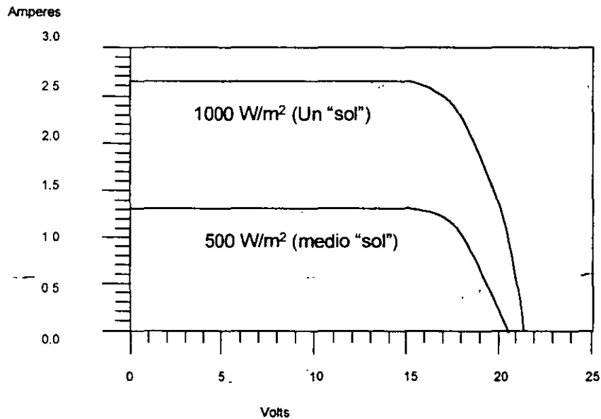
Figura 2.- Curva Típica Corriente - Voltaje de un modulo fotovoltaico a uno y a medio "sol"
