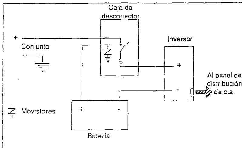
Figura 14. Se usan movistores para protección contra sobretensiones.
