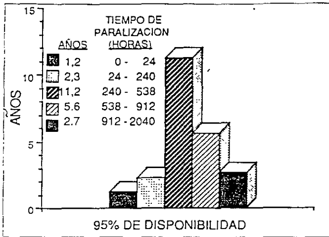
Figura 6. Tiempo de paralización anual (95%).
