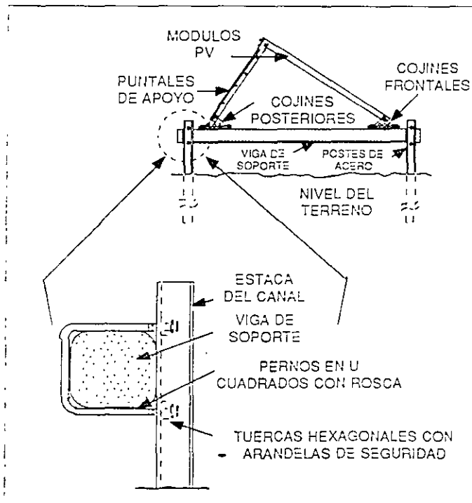
Figura 19. Montaje sencillo a nivel del terreno para conjuntos fotovoltaicos.
