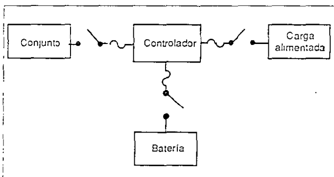
Figura 18. Ubicación de interruptores y fusibles.
