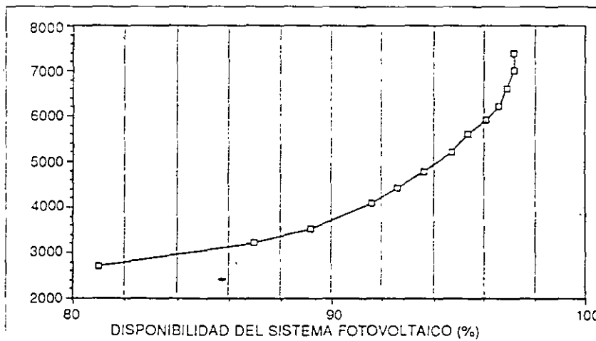
Figura 25. Costo en función de la disponibilidad de un sistema fotovoltaico solo (no híbrido) instalado en el noreste de Estados Unidos.
