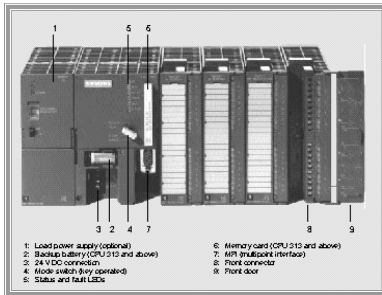
Figura 3.12. Principales Componentes del PLC.
