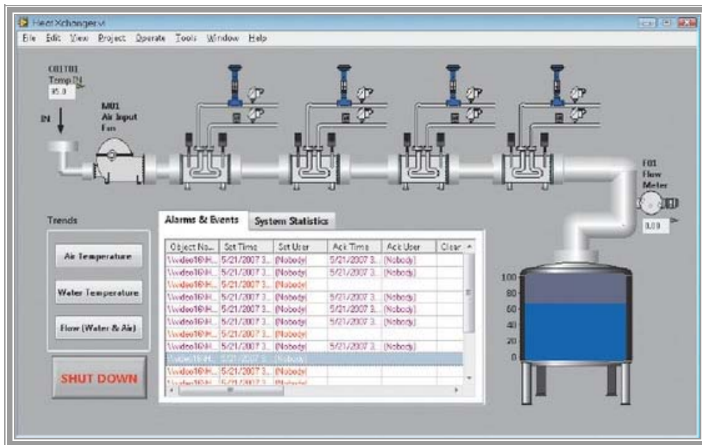
Figura 2.2. Visualización grafica de un sistema SCADA.
