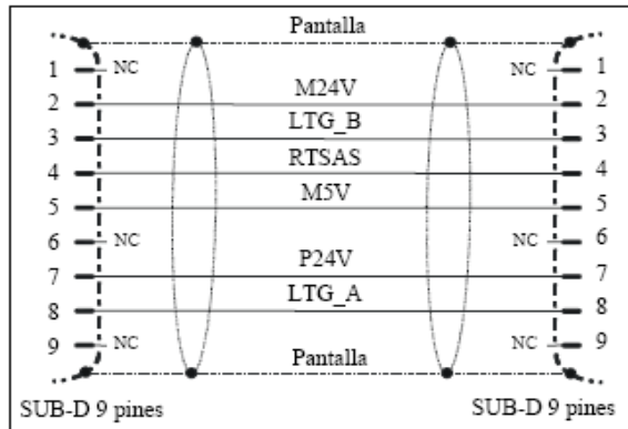
Figura 2: Cable MPI (0,3 m)
