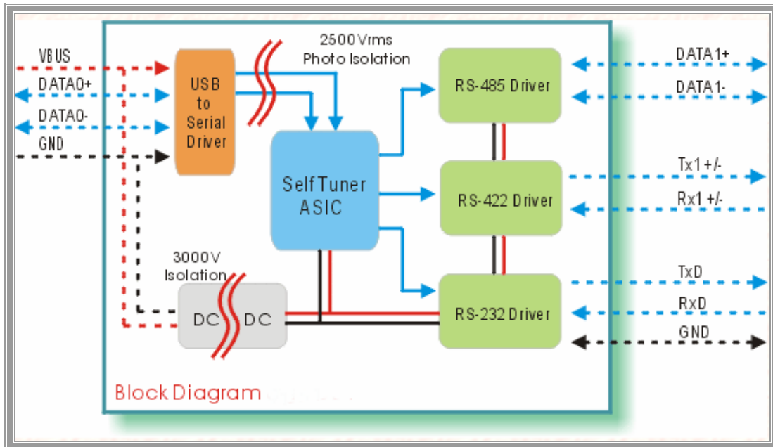
Figura 3.2. Diagrama básico convertidor USB a RS232/RS485.
