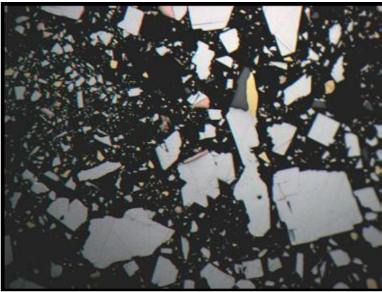
Fotografía 1. Superficie pulida de la muestra, se observan abundantes partículas de galena gris oscura con asociaciones de pirrotita rosa y escasas partículas de calcopirita amarilla.
