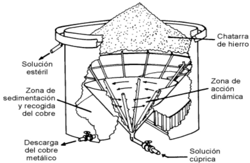
Figura 16. Esquema de un cono rotatorio para la cementación de cobre (Biswas A. K., 1993)
