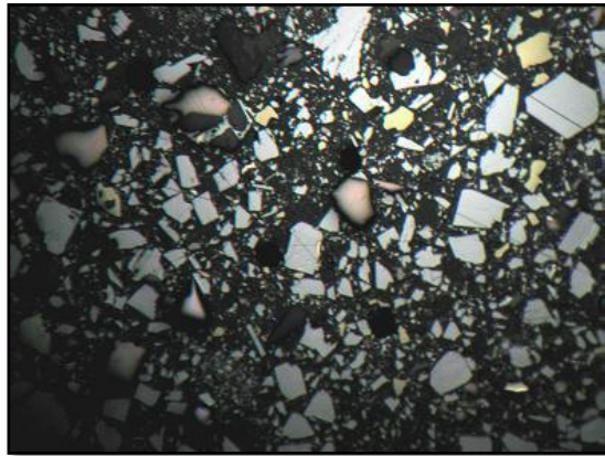
Fotografía 2. Superficie pulida de la muestra, se observan partículas libres de galena y asociadas a pirrotita y múltiples de esfalerita-calcopirita. Las partículas más pequeñas corresponden a galena, calcopirita y pirrotita.
