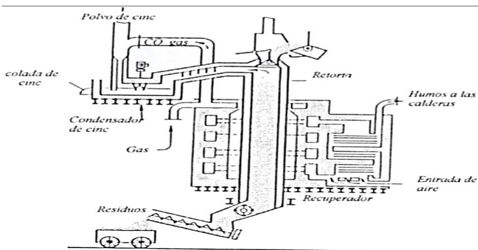
Figura 10. Esquema de un horno de retorta utilizado en el proceso de destilado de zinc (Lagos de la F. 2017)
