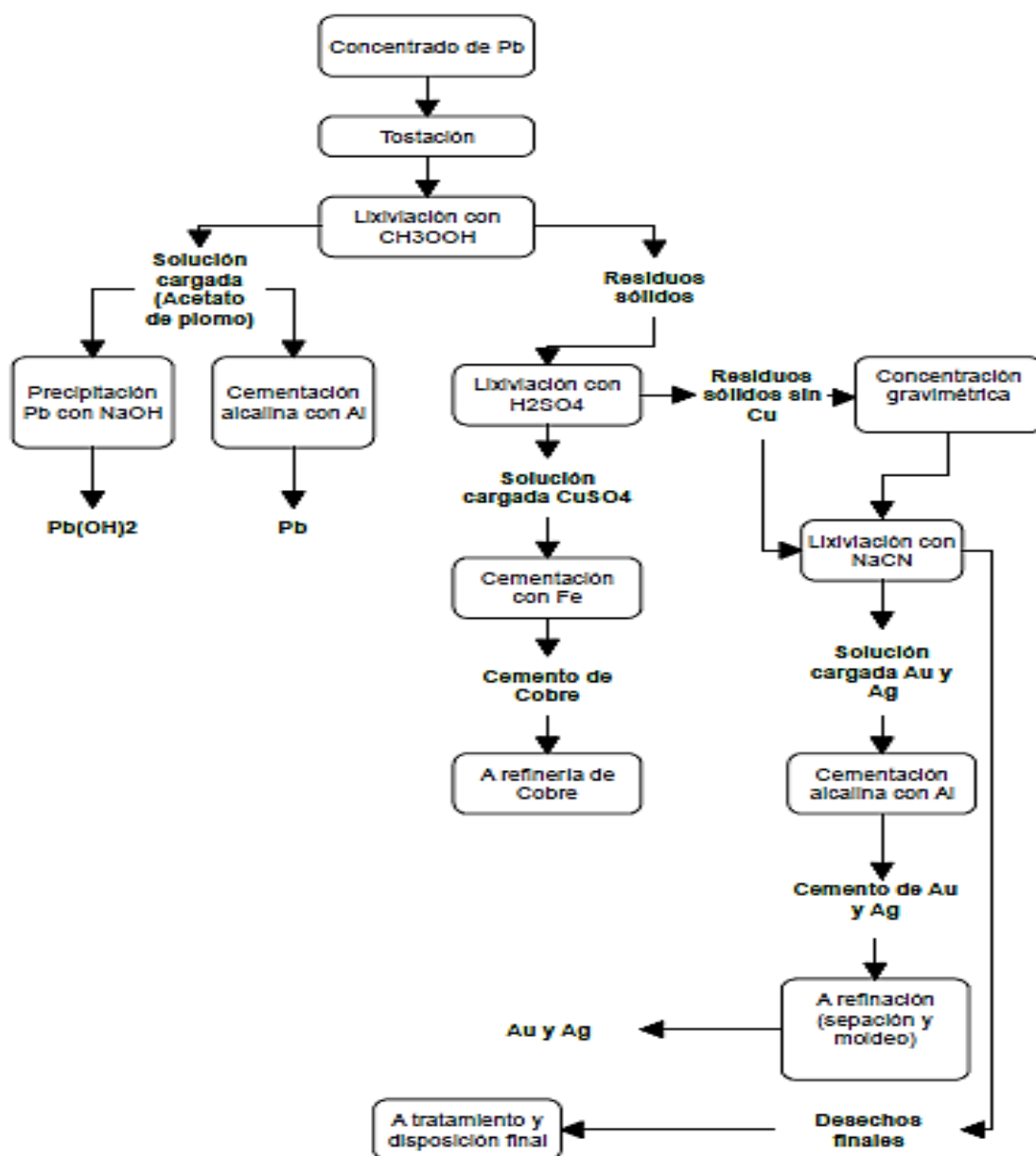
Diagrama 7. Proceso propuesto para el tratamiento de los residuos de la lixiviación ácida de Pb
