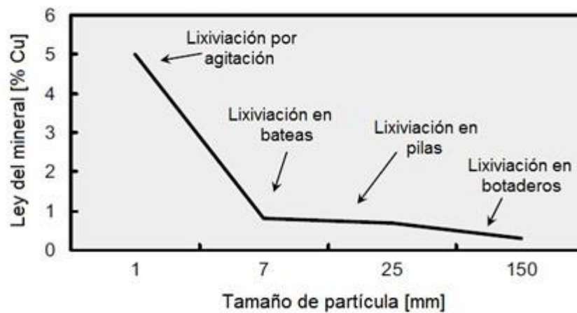
Gráfica 5. Selección del método de lixiviación al comparar tamaño de partícula vs ley mineral (Hinojosa O., 2016)
