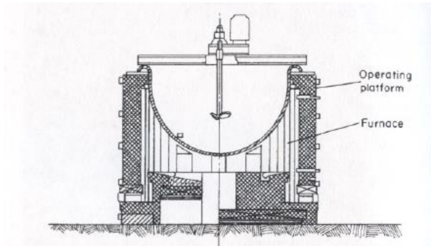
Figura 4. Paila típica usada en la refinación de plomo (Habashi F., 2002)
