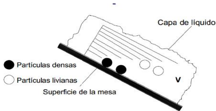
Figura 17. Esquema del comportamiento idealizado de las partículas según su tamaño en la mesa Wilfley (Velásquez S., 2018)
