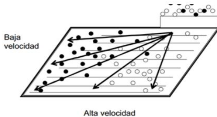
Figura 18. Esquema del comportamiento de la velocidad de las partículas según su tamaño; las partículas más densas viajan a una menor velocidad que las de menor densidad (Velásquez S. 2018)
