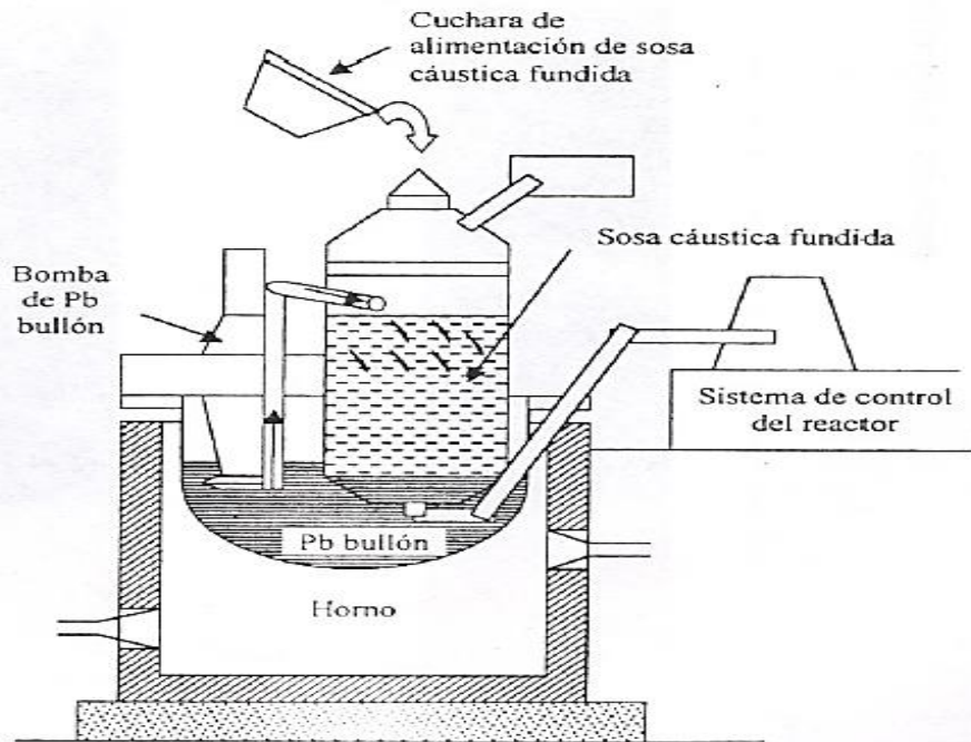
Figura 6. Paila utilizada durante el proceso Harris (Sancho, 2000)
