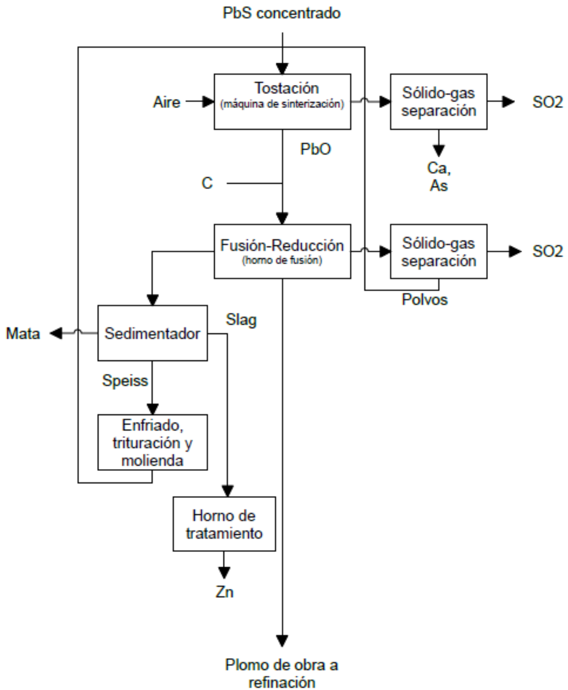
Diagrama 4. Secuencia del proceso pirometalúrgico para la obtención de plomo de obra (Habashi F., 2002)
