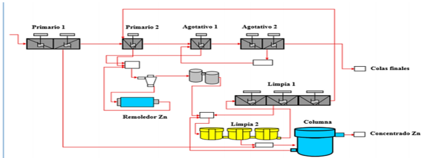
Diagrama 3. Circuito de flotación Zn Minera Tizapa (Roberto E., 2008)
