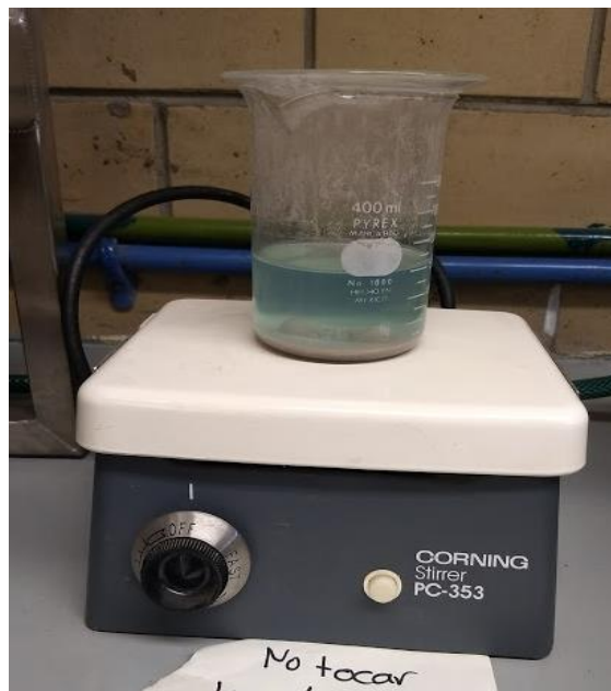
Fotografía 34. Lixiviación de la muestra con ácido sulfúrico (prueba preliminar)
