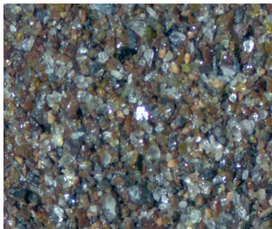
Fotografía 3. Superficie del residuo de la lixiviación de Pb, se observan con mayor detalle los óxidos de color marrón y en menor abundancia partículas de plata.
