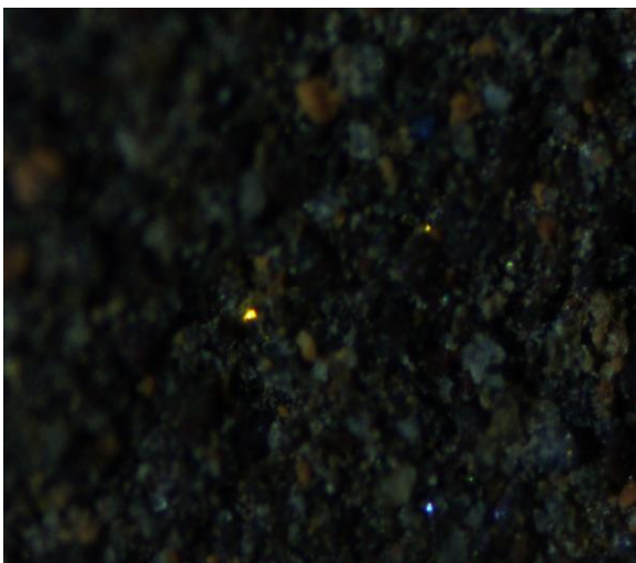
Fotografía 6. Superficie del residuo de la lixiviación ácida de Pb, se observan de forma no abundante partículas de oro.
