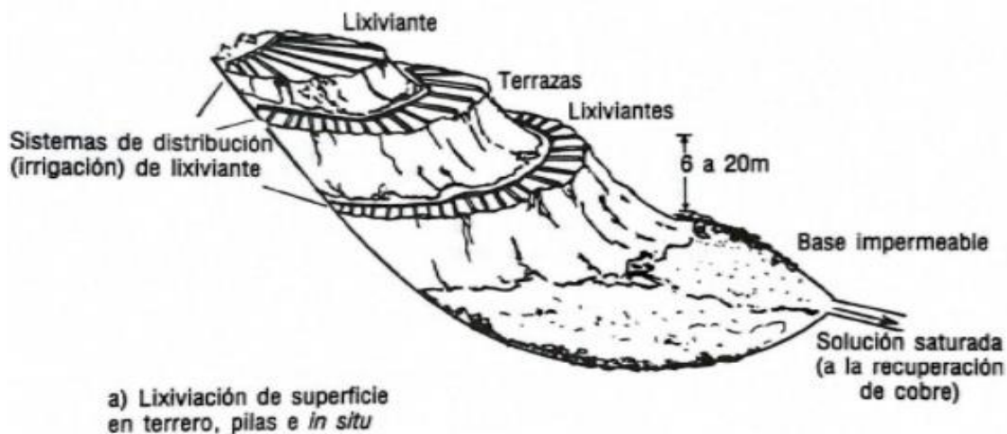
Figura 12. Esquema de un sistema de lixiviación de cobre en superficie tipo terrero (Biswas A. K., 1993)
