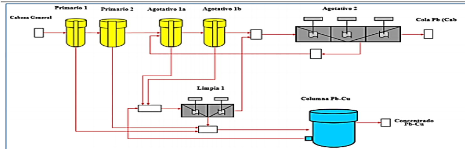
Diagrama 2. Circuito de flotación Pb-Cu Minera Tizapa (Roberto E., 2008)
