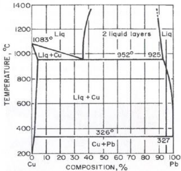
Gráfica 2. Relaciones de fases Pb-Cu según la temperatura (Habashi F., 2002)
