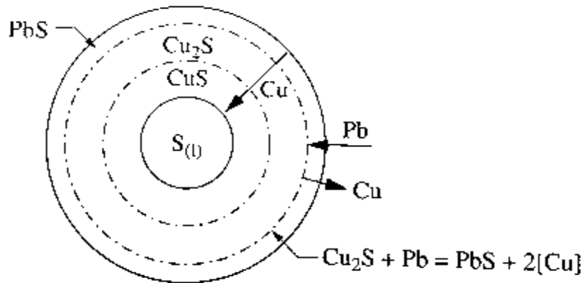
Figura 5. Comportamiento de los sulfuros de cobre y plomo durante la formación de mata (Vignes A. 2011)
