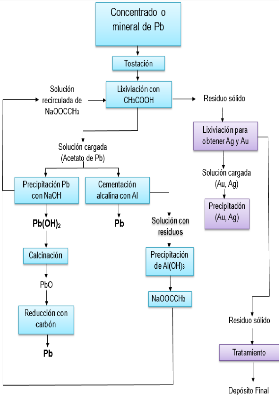
Diagrama 6. Proceso propuesto para la obtención de plomo a partir de una solución de acetato (García Villa M., 2016)
