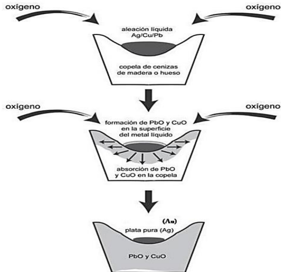
Figura 11. Esquema del proceso de copelación de oro y plata (LMS Consulting, 2018)
