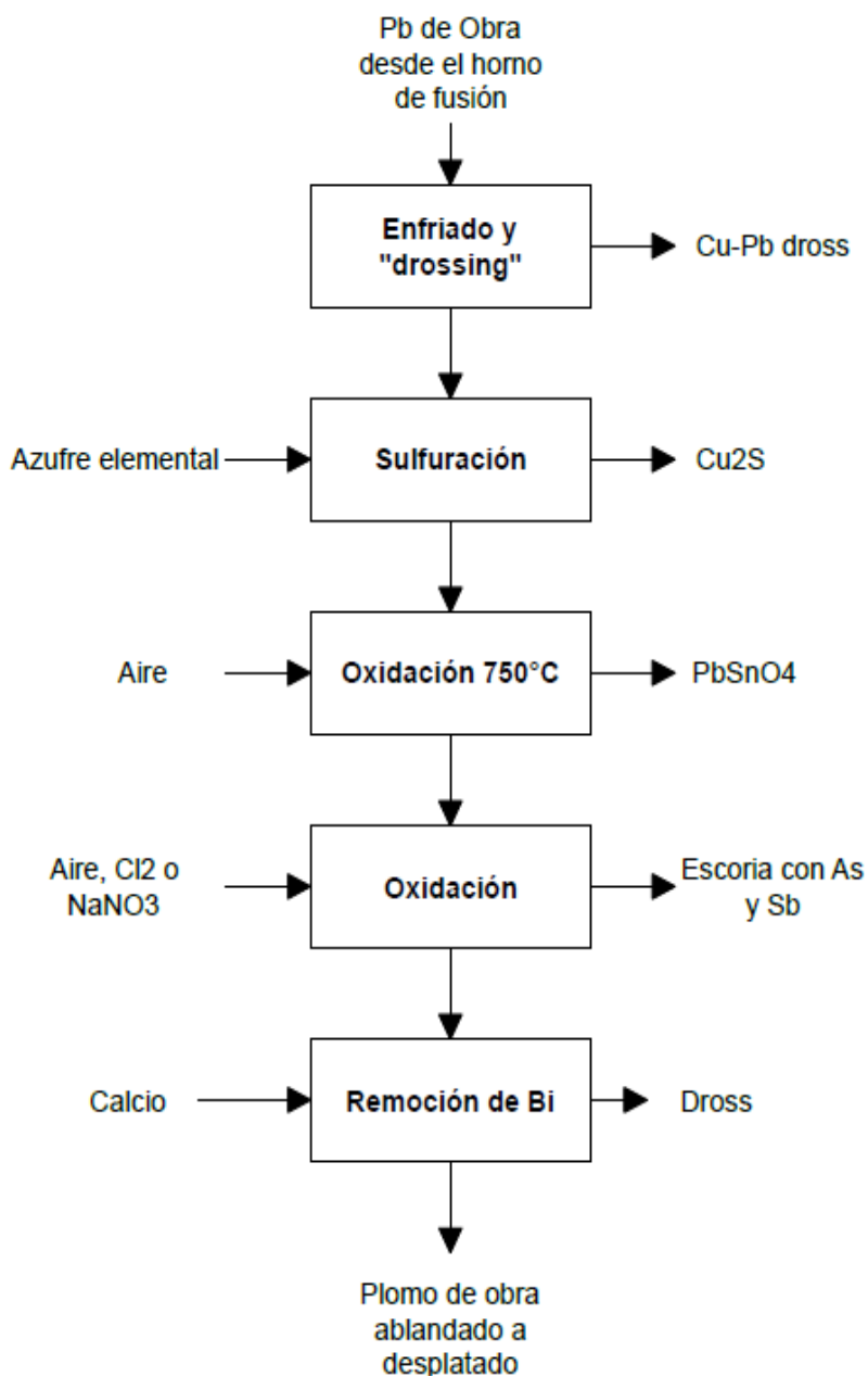
Diagrama 5. Secuencia del proceso pirometalúrgico del refinado de plomo de obra (Vignes A., 2011)
