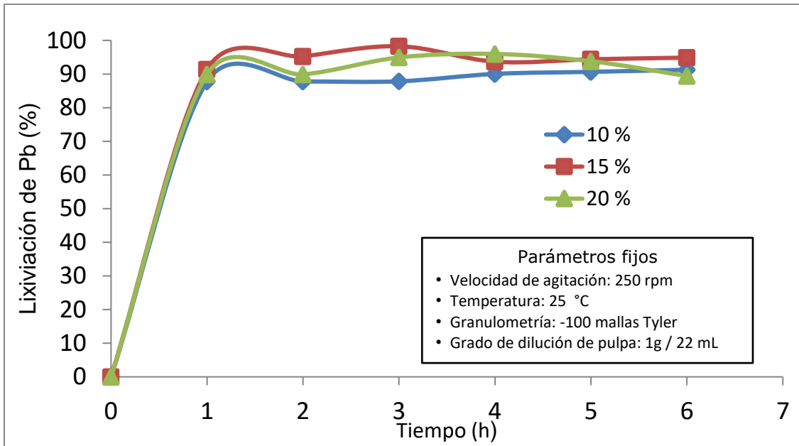
Gráfica 3. Efecto de la concentración de ácido acético en la intensidad de lixiviación de PbO (García Villa M., 2016)
