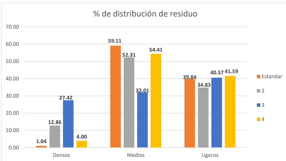
Gráfica 8. Comparativa de la distribución porcentual de las fracciones obtenidas en las pruebas gravimétricas
