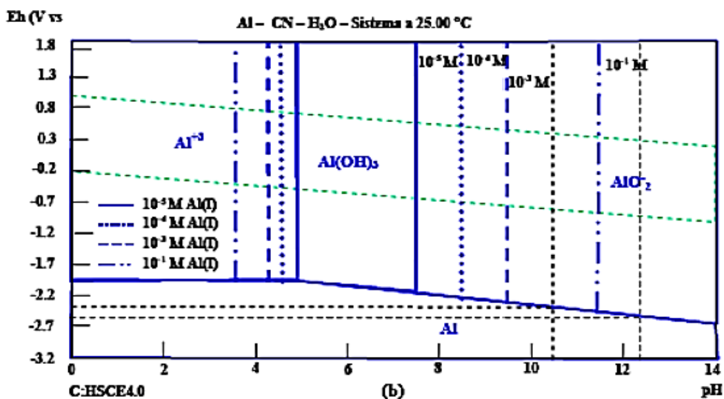
Figura 19. Diagramas de Pourbaix para la especie Al en una solución cianurada acuosa a concentraciones de: Al(I) variable y NaCN = 0.24 M (Pérez J. C., 2008)
