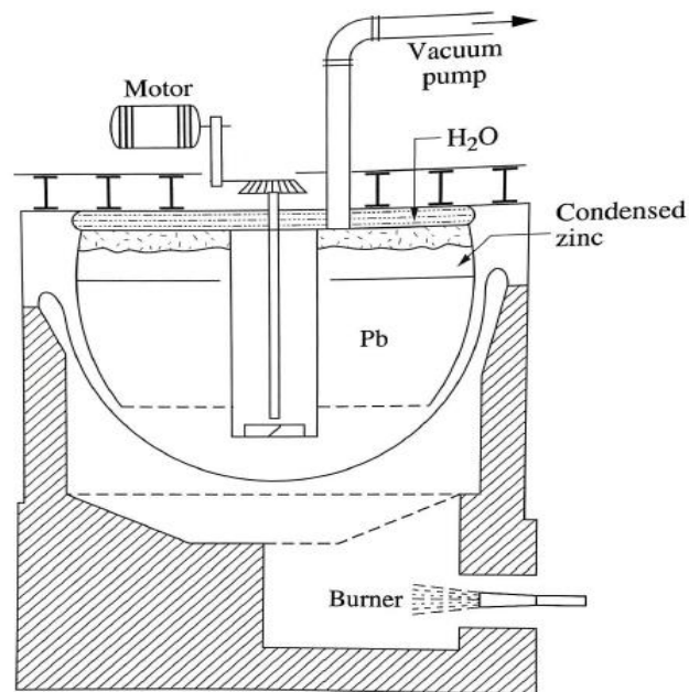
Figura 8. Paila al vacío utilizada en el proceso de descincado (Vignes A. 2011)
