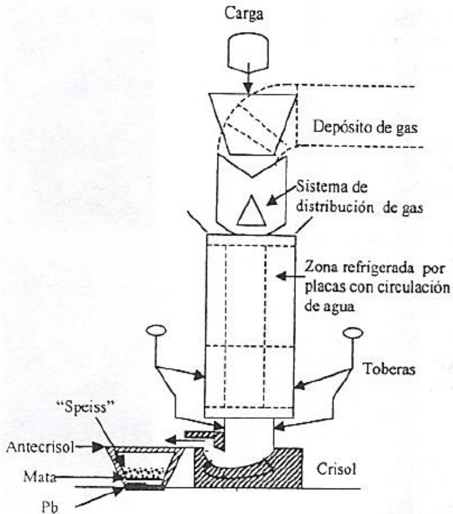
Figura 3. Alto horno de fusión-reducción de plomo (Sancho, 2000)
