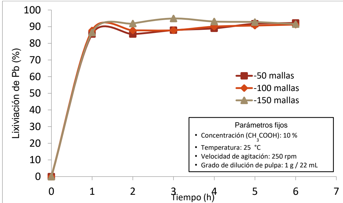
Gráfica 4. Efecto de la granulometría en la lixiviación de PbO (García Villa M., 2016)
