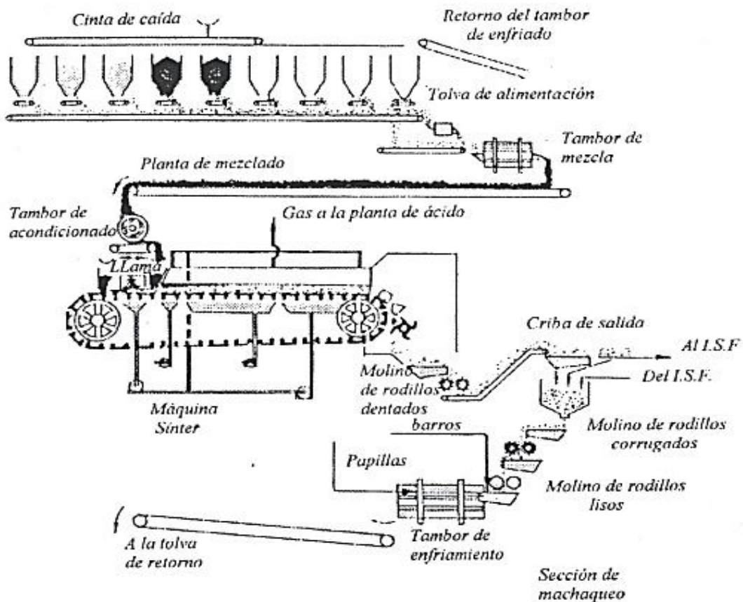
Figura 2. Máquina de tostación-sinterización Dwight-Lloyd (Lagos de la F., 2017)
