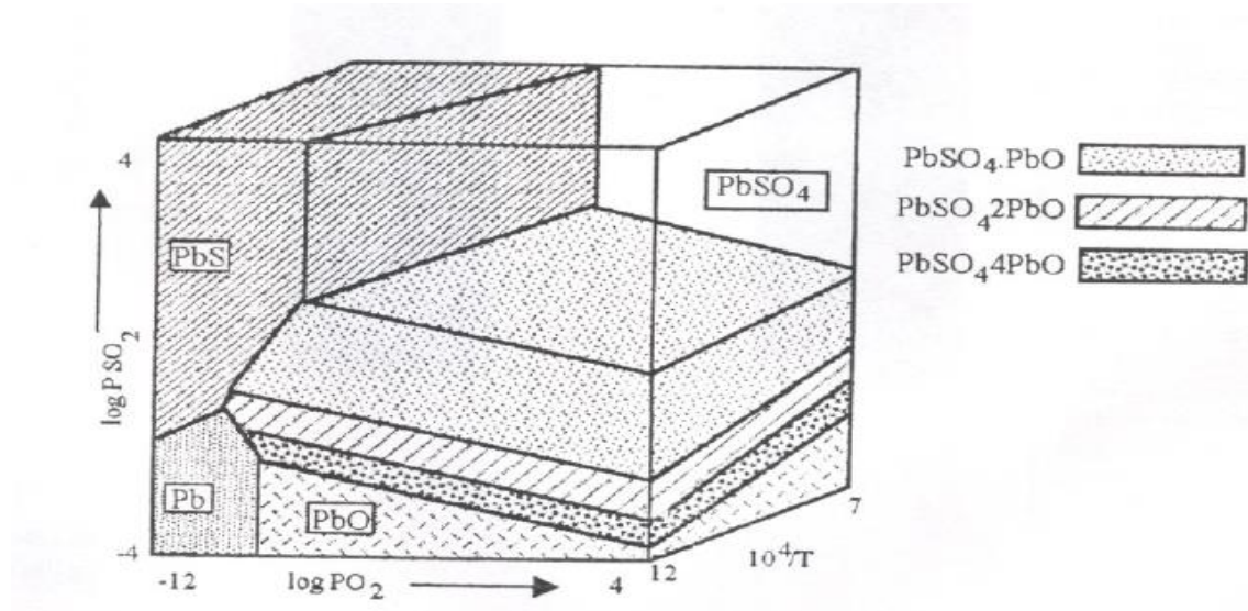
Figura 1. Diagrama de Kellogg para el sistema Pb-O-S (Sancho P., 2000)
