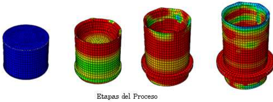
Figura 5.10: Etapas de la deformación en el proceso de extrusión combinado.
