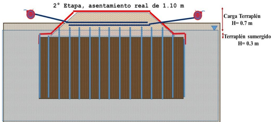
Figura 99.- “Sumersión del terraplén de tezontle durante la segunda etapa constructiva del panel de prueba de vacío (Menard Vacuum)”.
