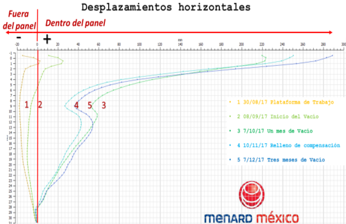
Figura 68.- “Historial de desplazamientos durante las diferentes etapas que cubren los primeros tres meses de aplicación del Vacío.” Fuente: Menard México.
