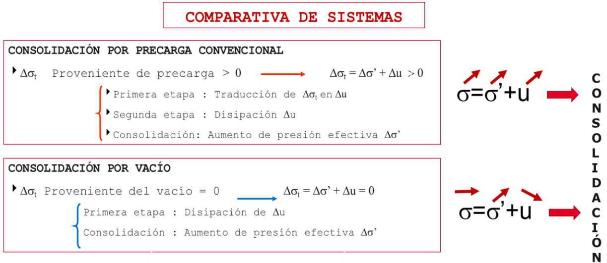
Figura 25.- “Comparativa de sistemas y análisis de esfuerzos.” Fuente: Menard México.
