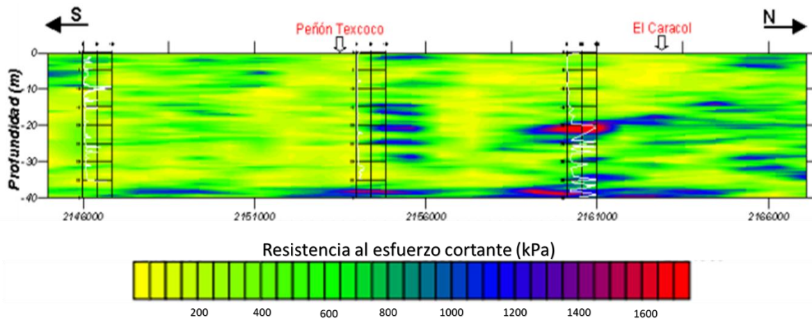
Figura 11.- “Resistencia al esfuerzo cortante del suelo arcilloso del Ex Lago de Texcoco”. Fuente: FI UNAM.
