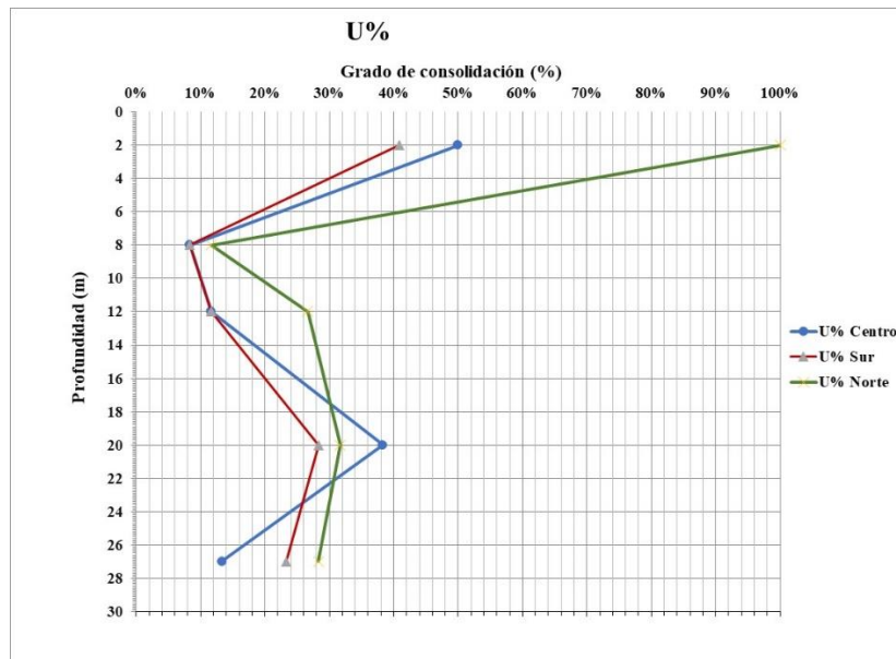
Figura 107.- “Grados de consolidación de cada Bahía, determinados con base a la variación de la presión intersticial registrada en los piezómetros electicos”.
