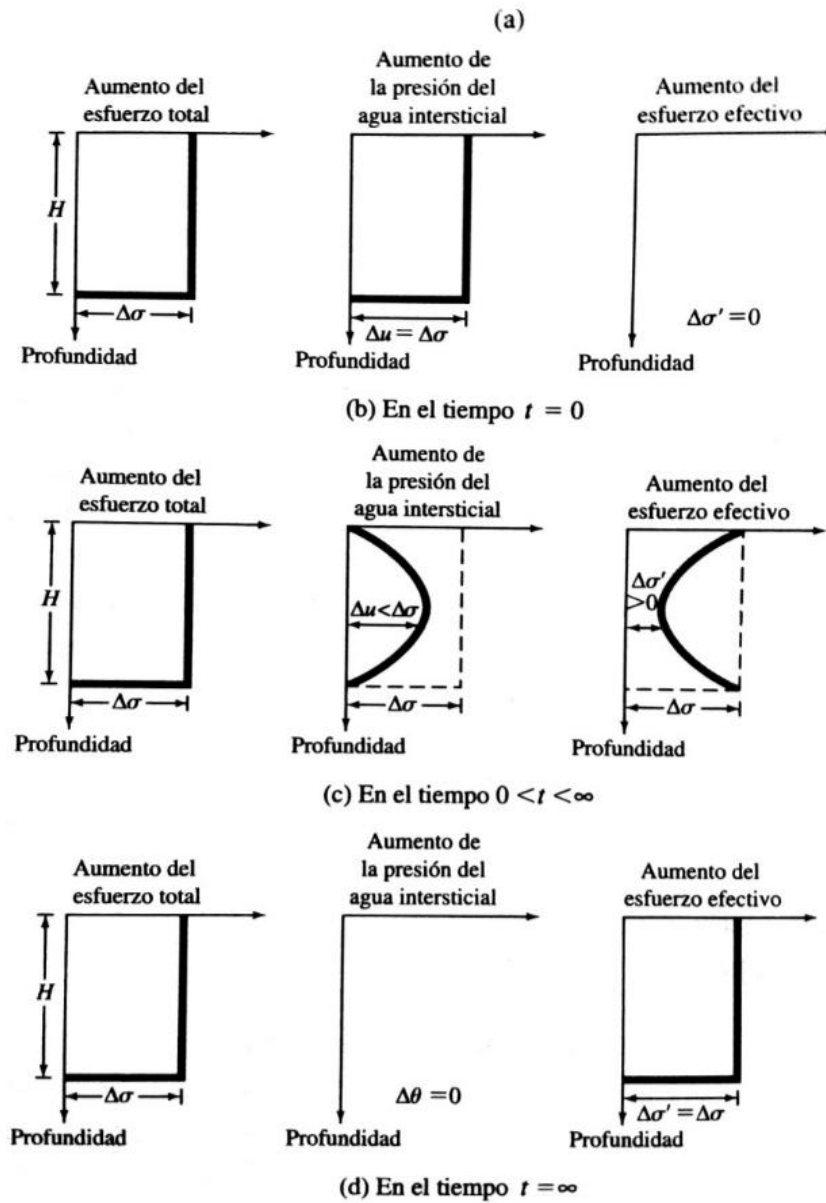
Figura 15.- “Variación del esfuerzo total, la presión intersticial y los esfuerzos efectivos durante un proceso de consolidación.”. Fuente: Braja Das, Fundamentos de ingeniería geotécnica.
