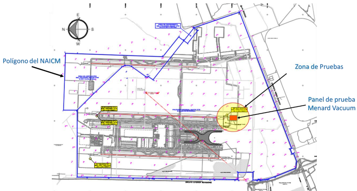
Figura 34.- “Ubicación de la zona de pruebas y de la prueba de Menard Vacuum, dentro del polígono del NAICM.” Fuente: GACM.
