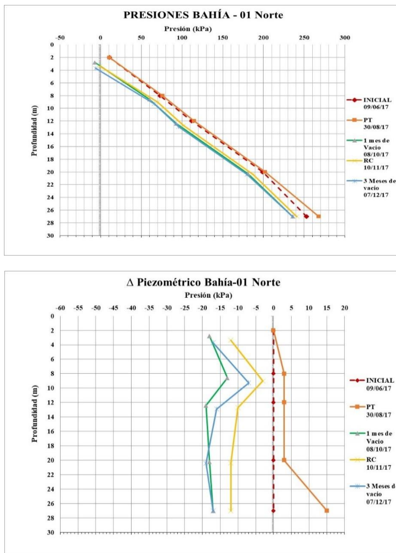
Figura 106.- “Variación de la presión intersticial en cada estrato, con base a cada etapa. Bahía Central”.
