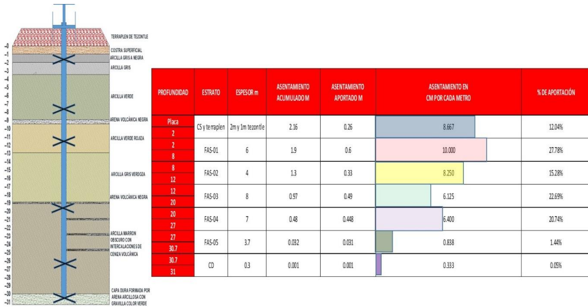
Figura 58.- “Porcentaje de aportación de cada uno de los estratos que se tienen monitoreados con las arañas magnéticas del extensómetro de la bahía Central. Así mismo se muestra la estratigrafía con la ubicación de las arañas magnéticas del extensómetro de la Bahía Central” Fuente: Menard México.
