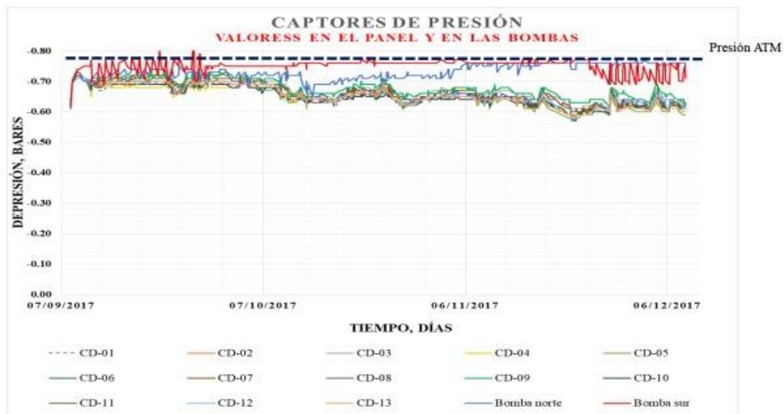
Figura 41.- “Gráfica del comportamiento de las presiones en el panel y las bombas de vacío, con escala vertical mínima y máxima, con el fin de notar la tendencia de las depresiones” Fuente: Menard México.
