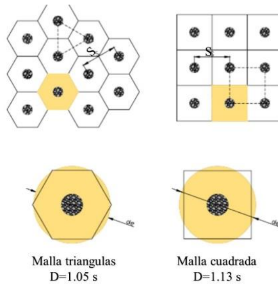
Figura 94.- “Diámetro de influencia de drenaje según el arreglo o malla de drenes verticales”.
