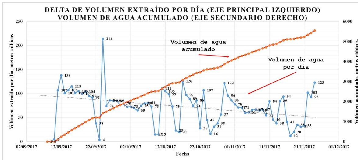
Figura 43.- “Variación del volumen de agua extraída total por cada día y volumen de agua total acumulado” Fuente: Menard México.
