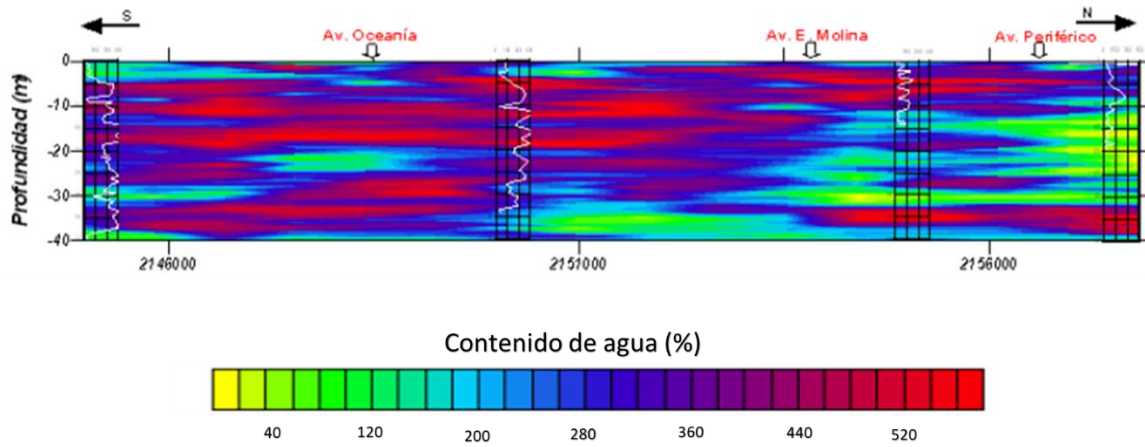
Figura 12.- “Contenido de agua del suelo arcilloso del Ex Lago de Texcoco”. Fuente: FI UNAM.
