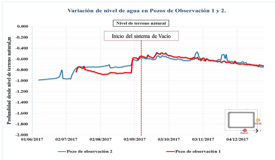
Figura 70.- “Comportamiento del Nivel freático durante la aplicación del Vacío.” Fuente: Menard México.
