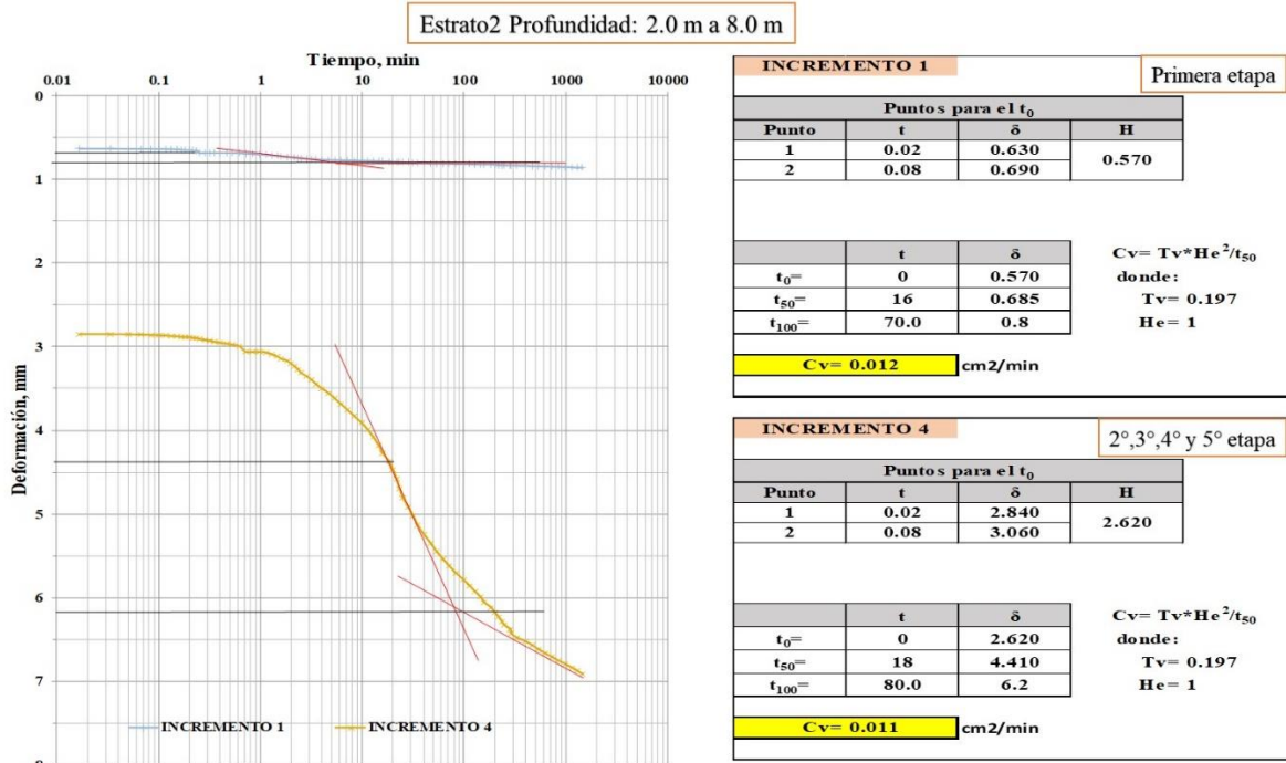
Figura 87.- “Coeficientes de Consolidación del estrato dos (2.0 m a 8.0 m), con base a la curva de compresibilidad y al incremento de cargas en el laboratorio, proporcional al incremento de carga real estimado en el sitio de prueba.
