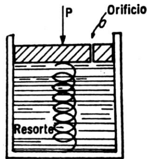
Figura 16.- “Esquema del modelo mecánico de Terzaghi para la comprensión del fenómeno de la consolidación.”. Fuente: Juárez Badillo, Mecánica de suelos Tomo I .
