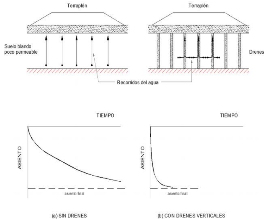
Figura 22.- “Terraplén sobre suelo blando poco permeable, sin drenes y con drenes verticales” Fuente: Uriel A. 1991.
