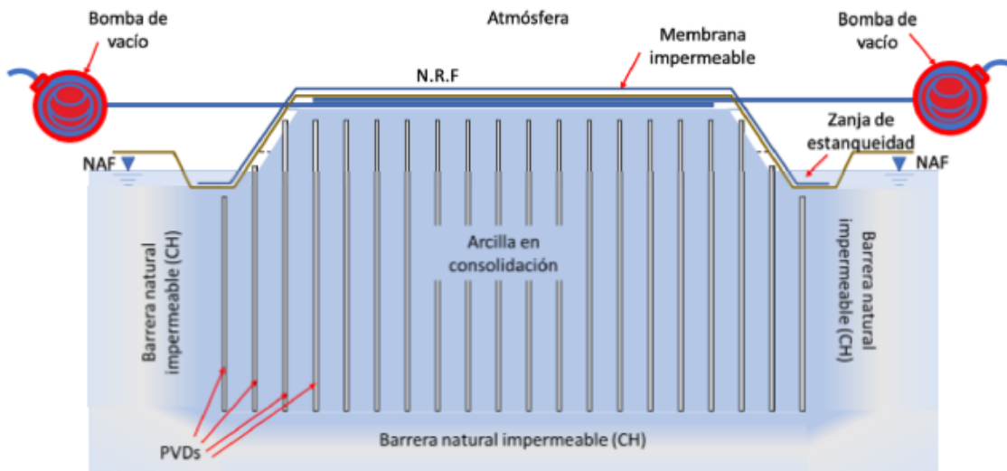
Figura 69.- “Comportamiento del Nivel freático fuera y dentro de la zona tratada durante la aplicación del Vacío.” Fuente: Menard México.
