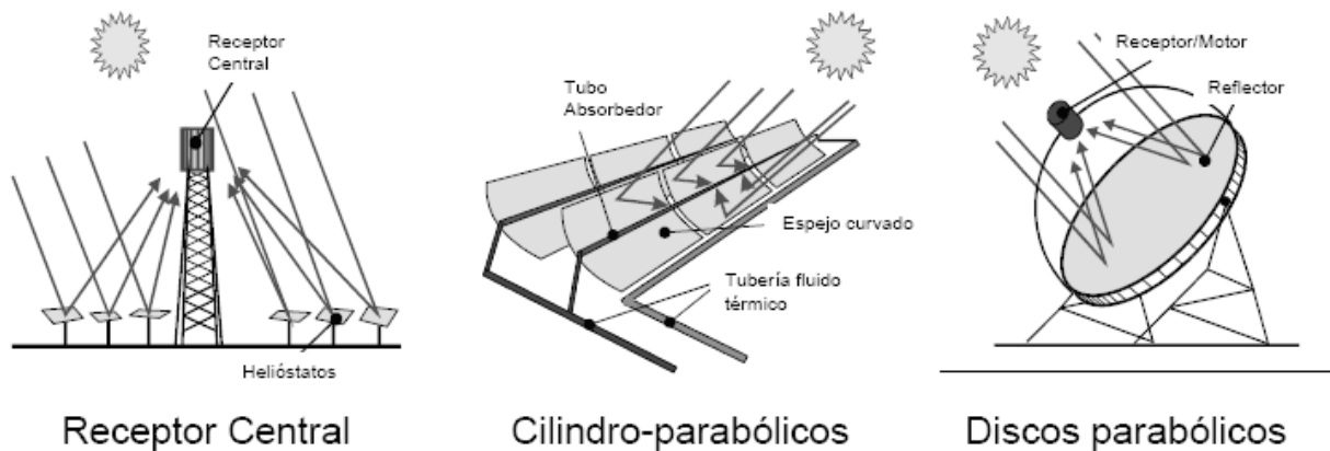
Fig.2 Configuraciones más habituales de los sistemas de concentración solar por reflexión (Romero, 2008)
