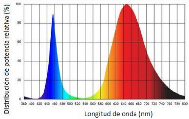
Figura 4.3.2 Espectro de emisión de luz led elegida
