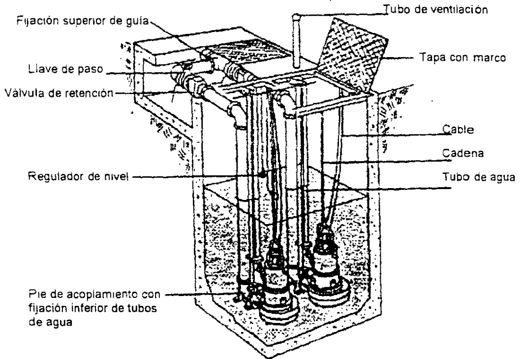
Fig. 4.14 Instalación de bombas con impulsores monocanal tipo Flygt
