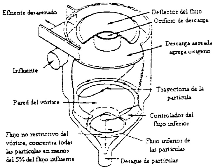
b) Tipo "Taza de Té" (Acero)
