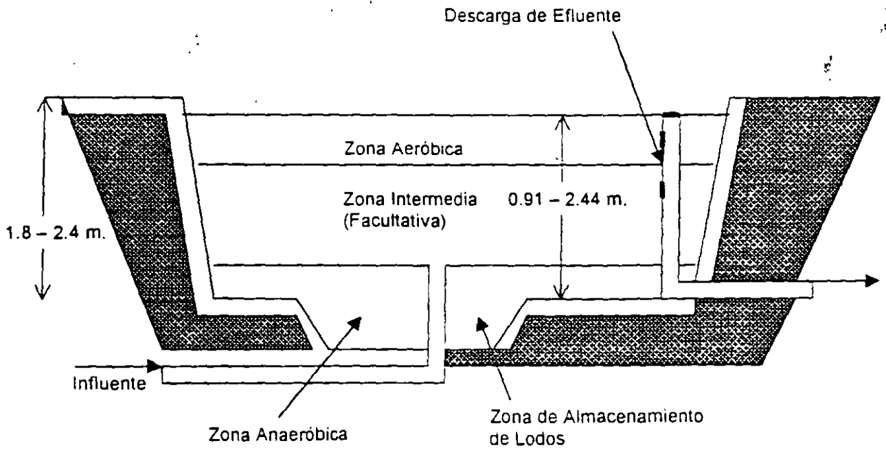
Fig 9.5 Laguna Facultativa (CNA)
