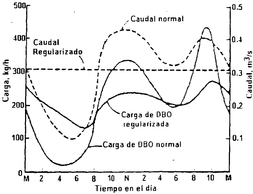
Figura 6.26 Graficación de los valores de caudal y carga de DBO normales y corregidos por igualación del flujo del ejemplo.
