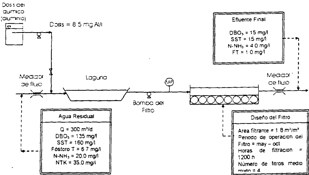
Fig. 9.8 Diagrama de flujo con el proceso New Hamburg
