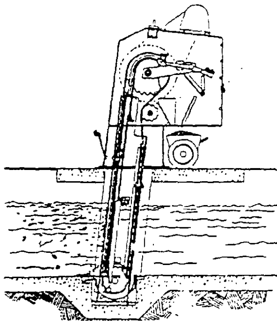
Figura 6.2 Rejilla mecánica de limpieza frontal
