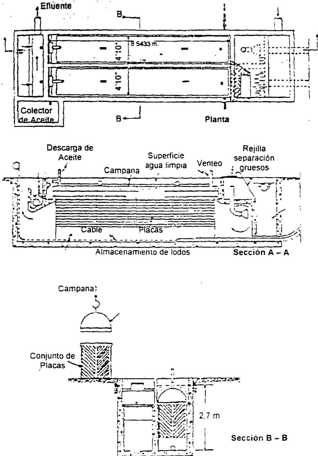
Fig. 6.20 Separador PPI
