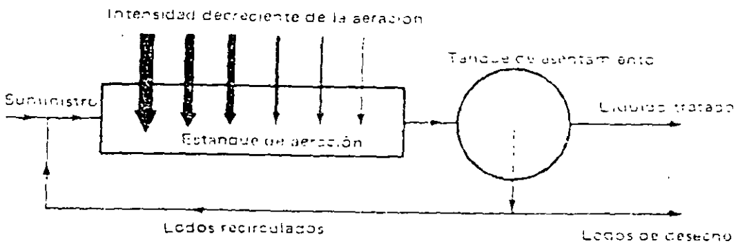
Figura 8.7 Aireación por etapas en un sistema de flujo pistón
