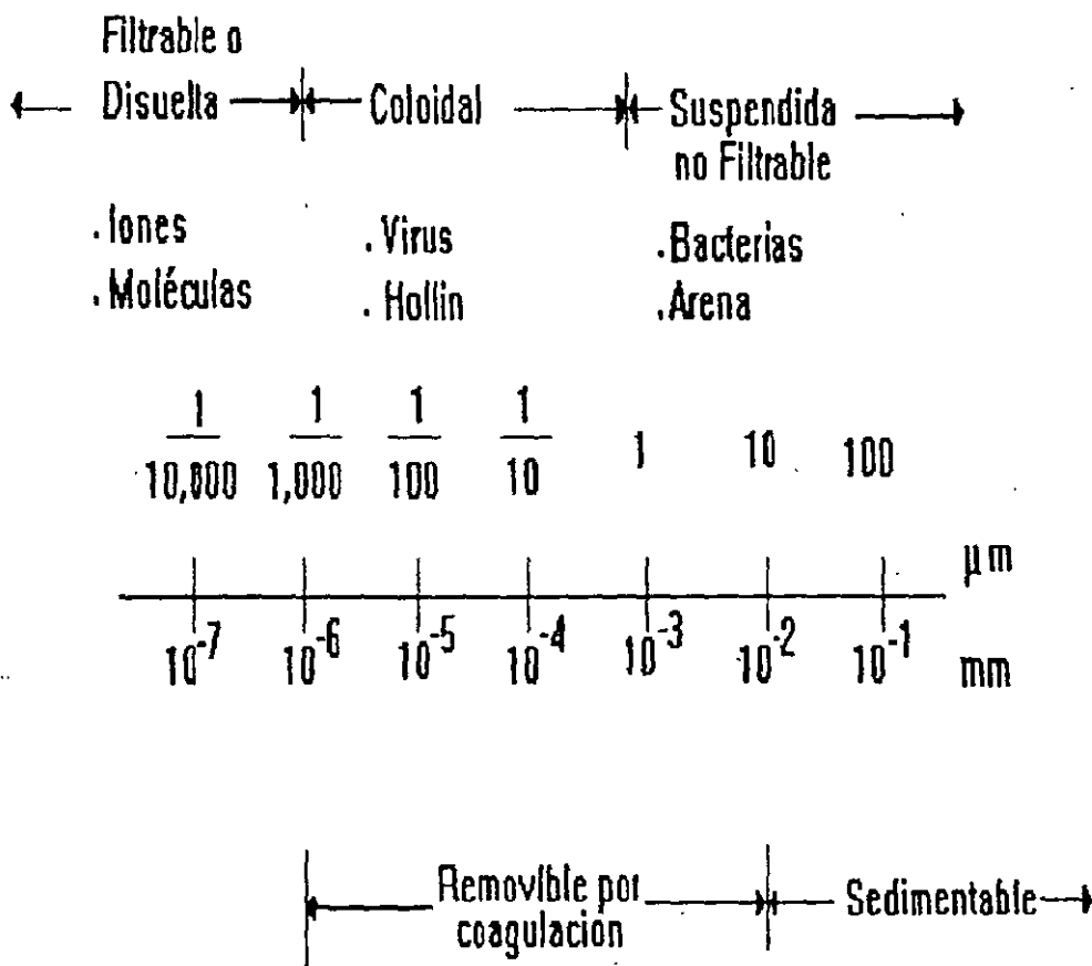
Fig. 2.2 Clasificación y tamaño de partículas presentes en el agua
