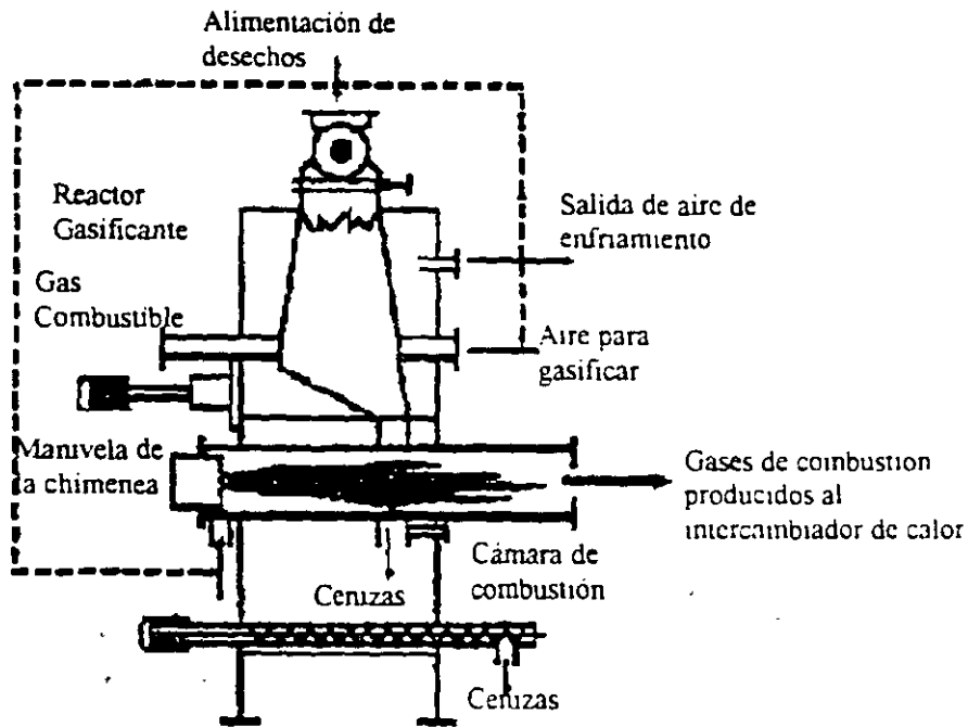
Figura 12.13 Gasificador de flujo cruzado (VER - cross - flow)
