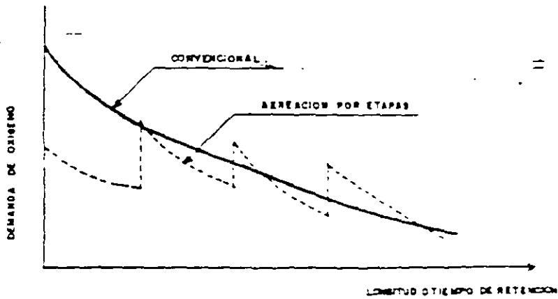
Figura 8.6 Demanda de oxígeno en el proceso de lodos activados
