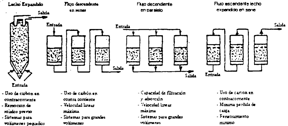
Fig. 10.7 Sistemas típicos de adsorción con carbón activado y sus atributos
