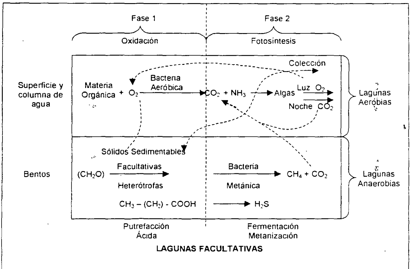
Figura 9.3 Actividades biológicas y clasificación de las lagunas de estabilización
