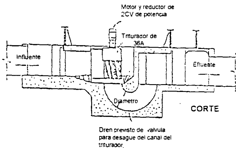
Figura 6.10 Planta y sección transversal de una instalación de trituración
