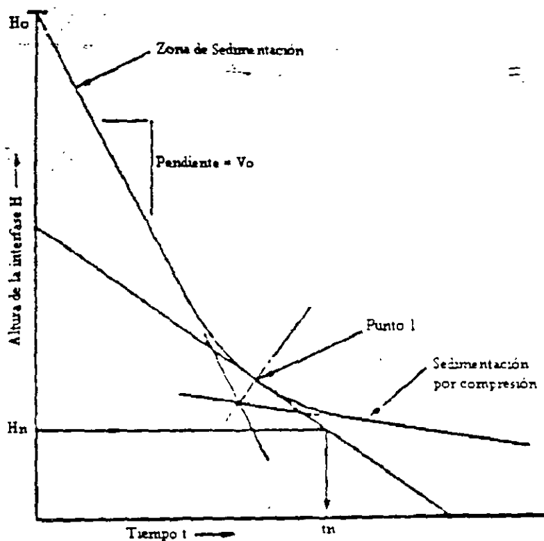
FIG. 7.14 Análisis de la curva de sedimentación en una suspensión concentrada, proceso batch.
