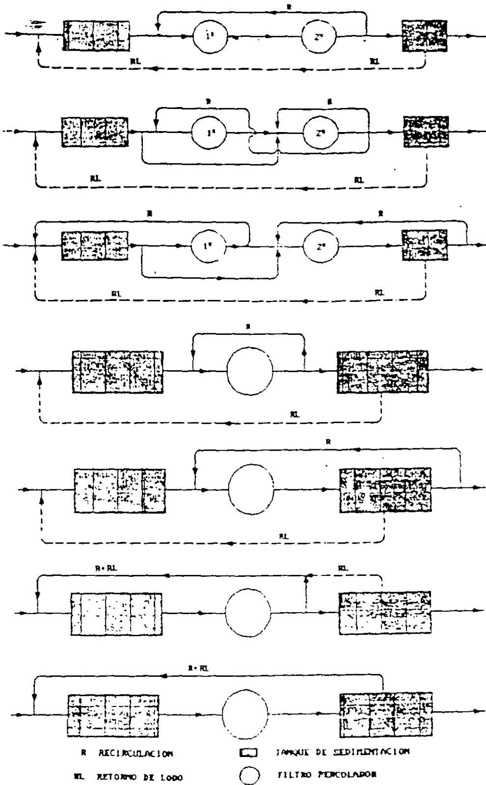
Fig. 6.23 Diferentes arreglos de los filtros percoladores
