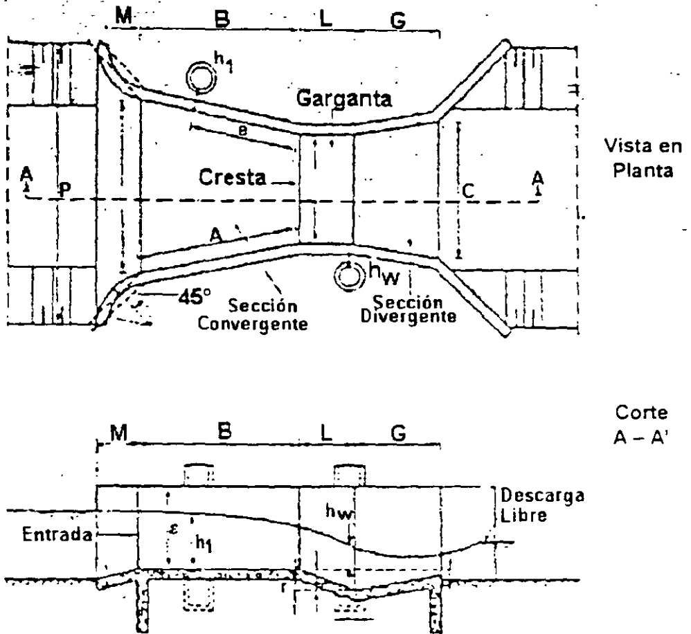
Figura 6.18 Geometria de un canal parshall
