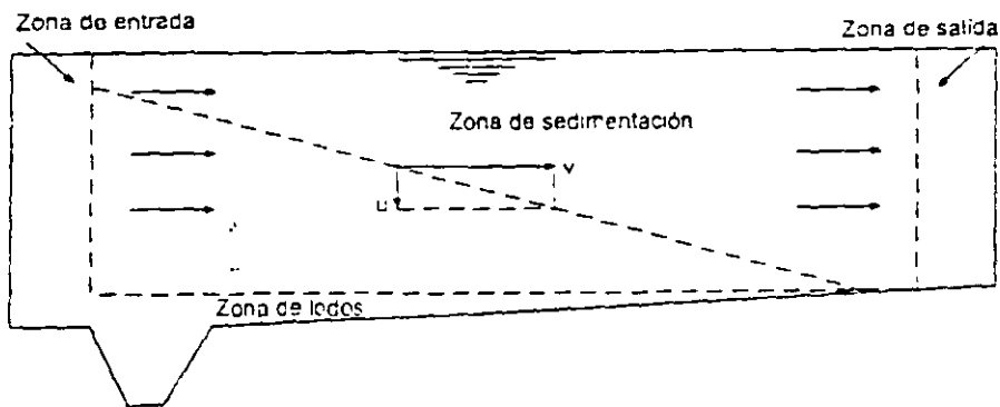
Figura 7 3 Zonas hipotéticas en un tanque sedimentador rectangular
