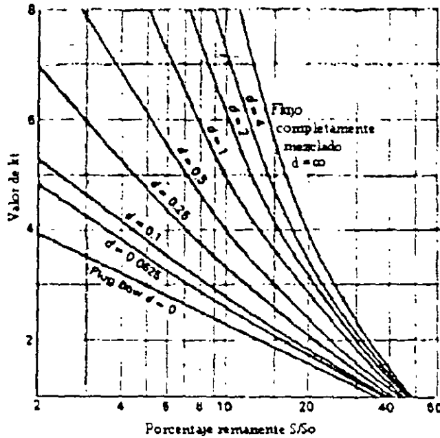
Fig. 9.6 Valores de kt en la ecuación de Wehener y Wilhelm, versus el remanente ( S/S_0 ) para varios factores de dispersión ( d )
