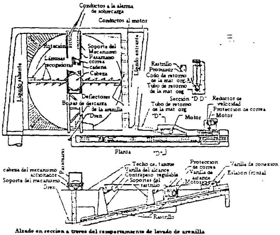
Figura 6.14 Desarenador de sección cuadrada o tanque de detritus
