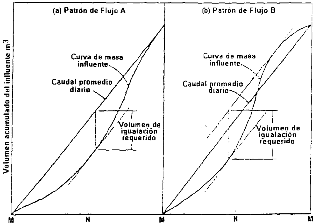
Fig. 6.24 Curvas de masas para la determinación del volumen de igualación requendo para dos patrones típicos de flujo.
