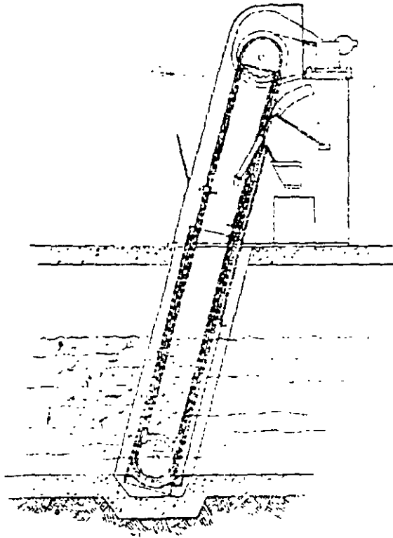
Figura 6.2 Rejilla mecánica de limpieza frontal
