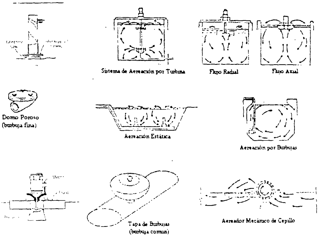
Fig. 8.15 Equipos aireadores
