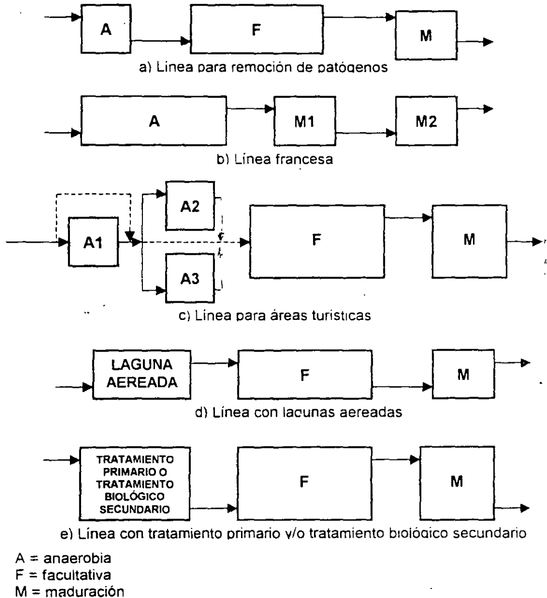
Figura 9.2 Arreglos comunes en sistemas lagunares
