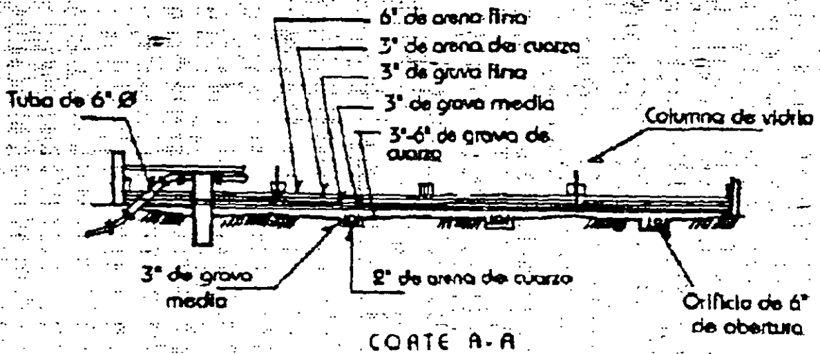
Fig. 12.8 Lecho de secado, corte A-A
