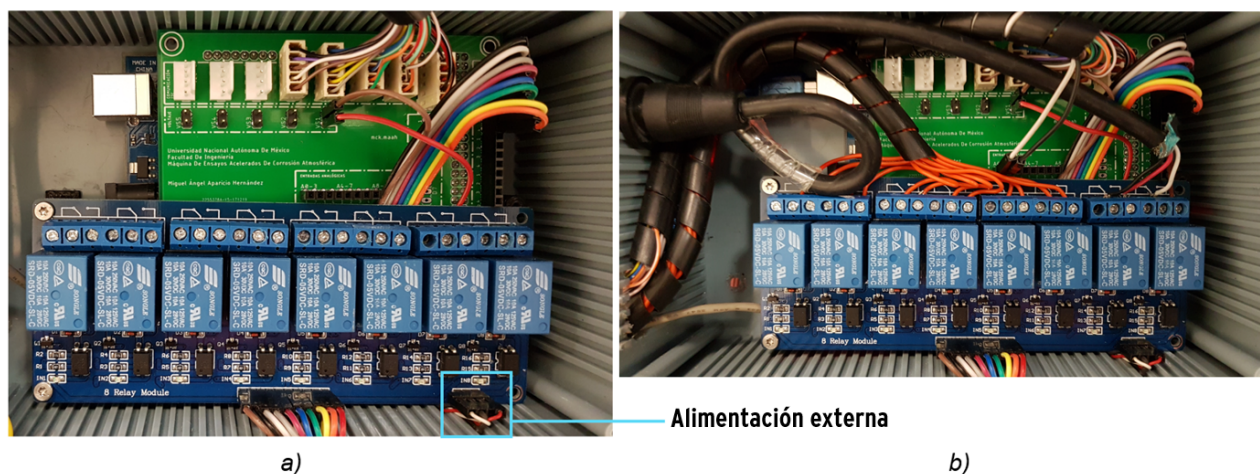
Fig.4.7 a) Relevadores y microcontrolador montados b) Conexiones realizadas de los relevadores a las válvulas de los gases
