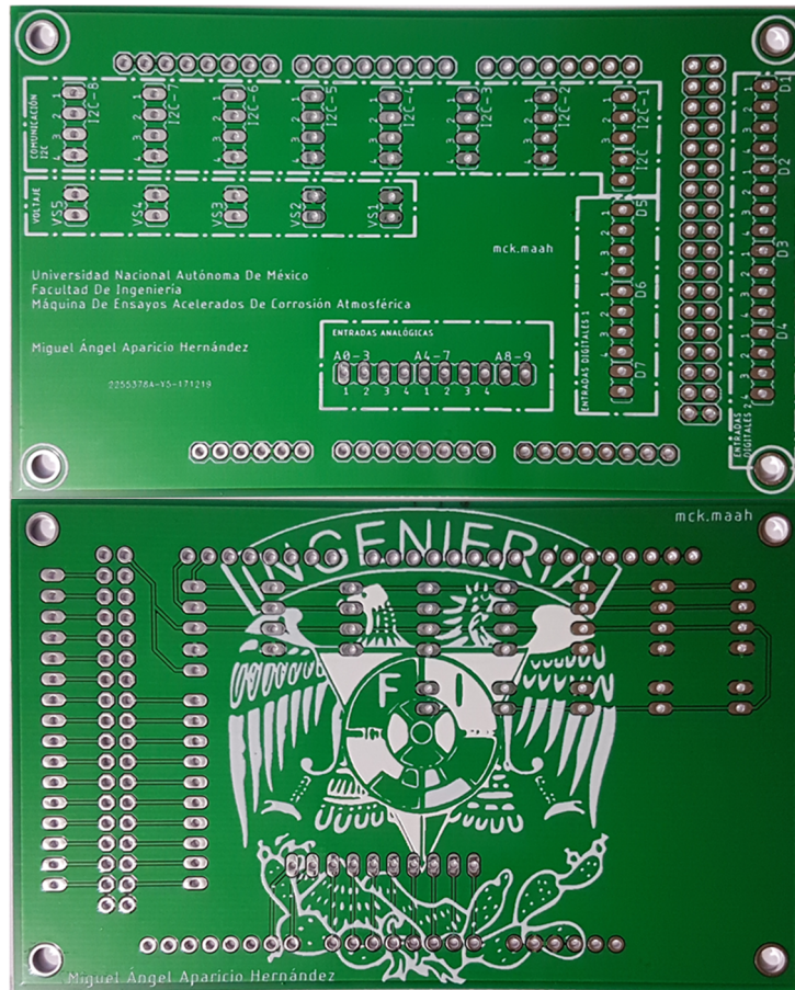
Fig.A.3 Tarjeta de expansión manufacturada
