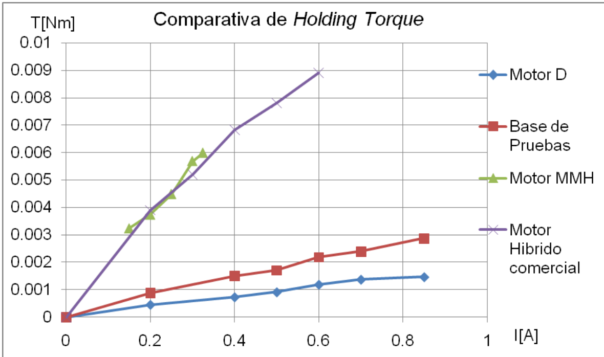
Figura 5.24. Gráfica comparativa de Holding Torque con dos estatores.
