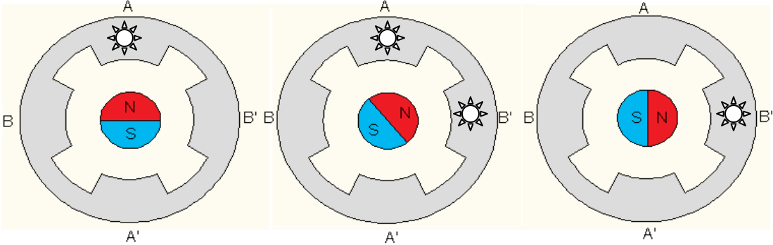
Figura 1.6. Funcionamiento de un motor a pasos MMP.
