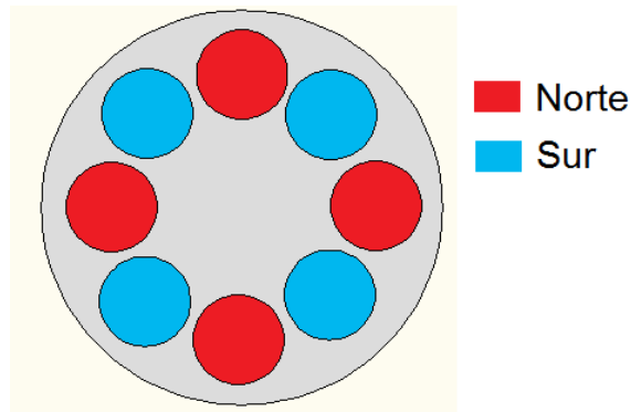
Figura 3.1. Posicionamiento de imanes en un rotor de un motor de imán permanente.
