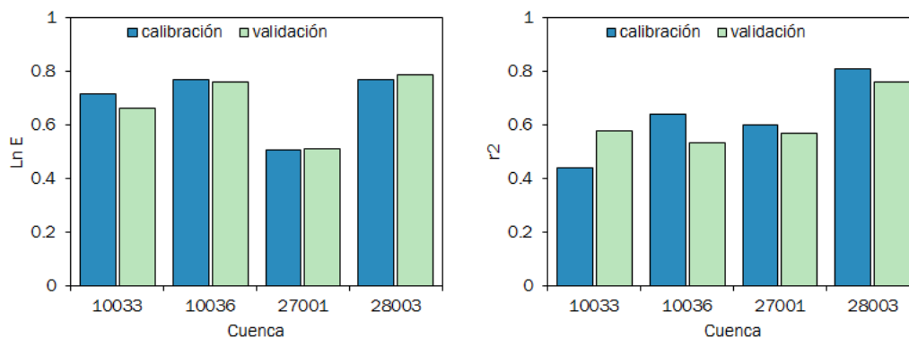
Figura 5-1. Valores del coeficiente de Nash-Sutcliffe Log (izquierda) y del coeficiente de determinación (derecha) para los diferentes periodos en las diferentes cuencas.
