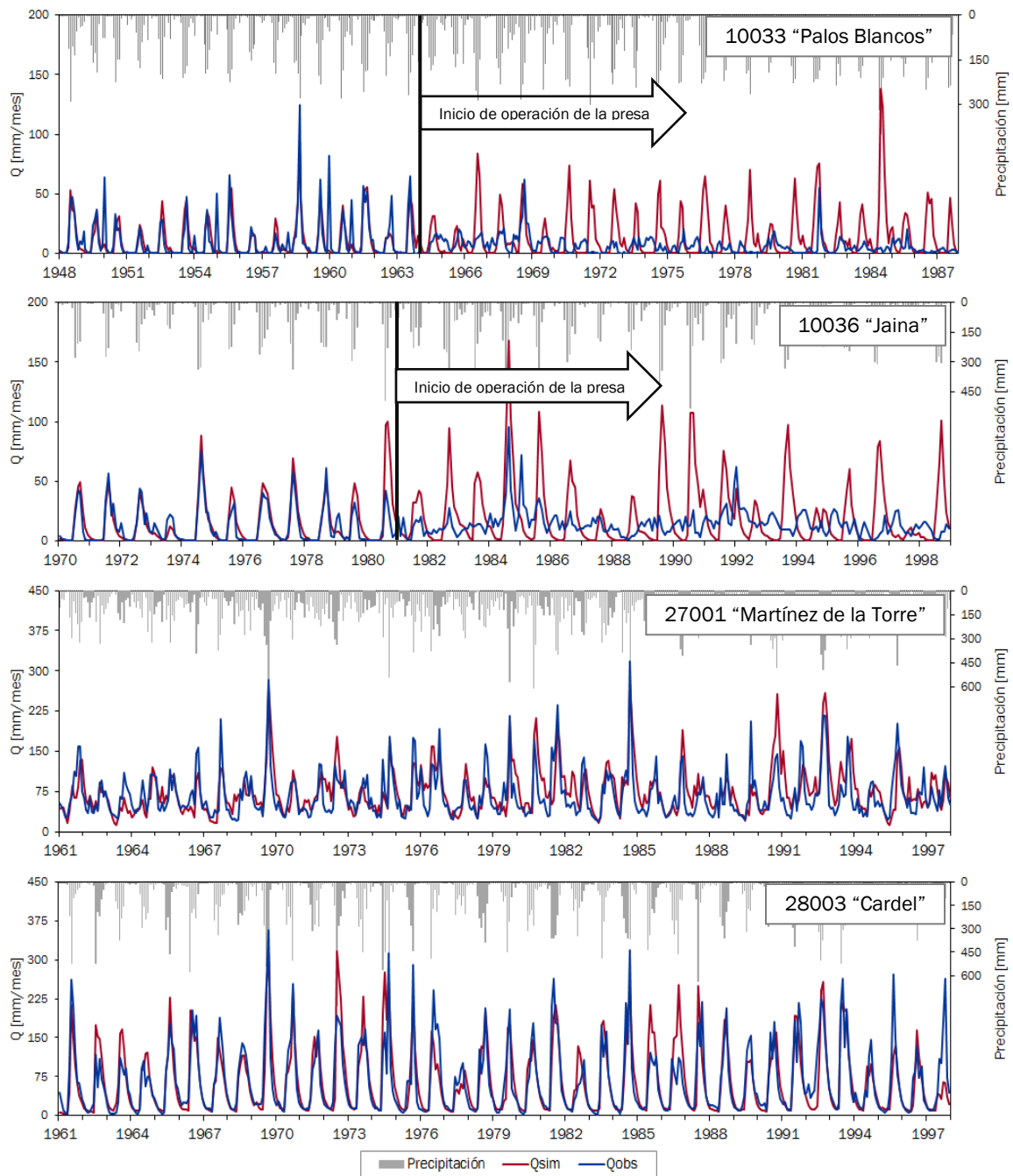
Figura 5-2. Esguerrimiento observado (línea azul) y simulado (línea roja) para cada una de las cuencas analizadas.
