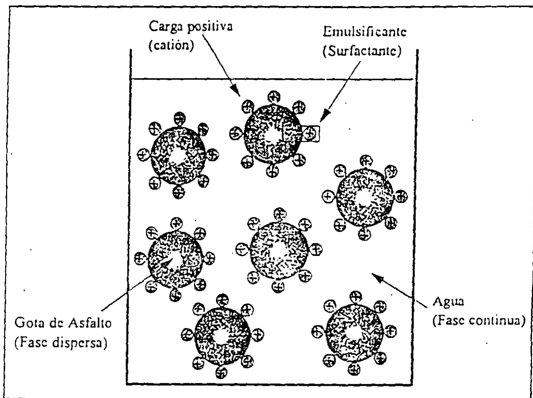
Figura 5.- Emulsión catiónica
