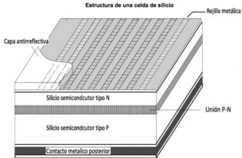
Figura 3.3 Estructura de una celda de silicio. Fuente: Propia.
