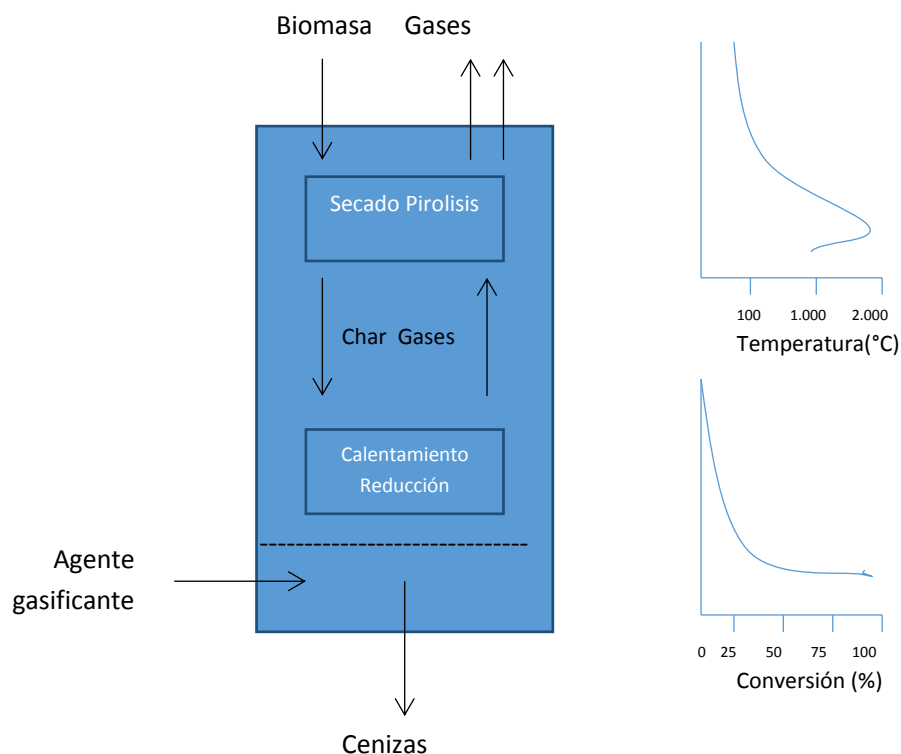
Figura 2.7 Flujo de materia y perfiles de temperatura y conversión en un reactor updraft (Bridgwater. 1989)
