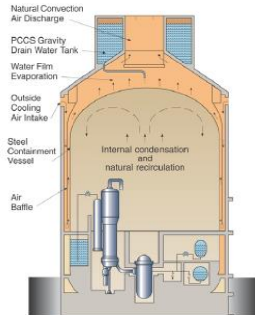
FIG 7 .Contención pasiva del reactor [11].
