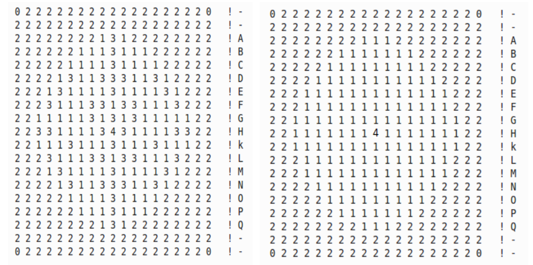
FIG 26. Núcleo al 70 y 100 % MOX.
