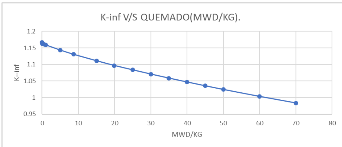
FIG 27. Cálculo de K_{\infty} contra quemado.
