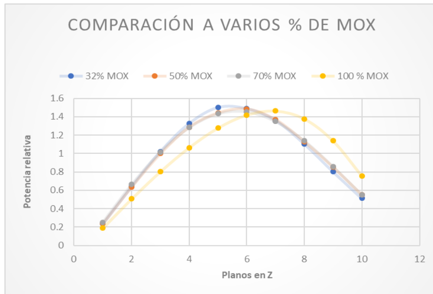
FIG 43. Comparación del factor pico de potencia axial para todos los escenarios.
