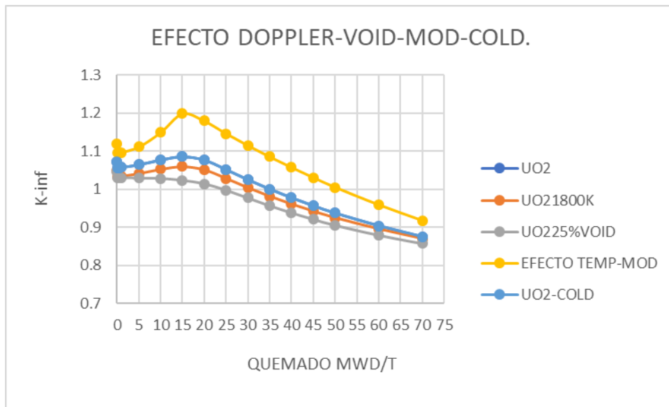
FIG 31. Comparación de diferentes condiciones de operación para el combustible UO 2 .
