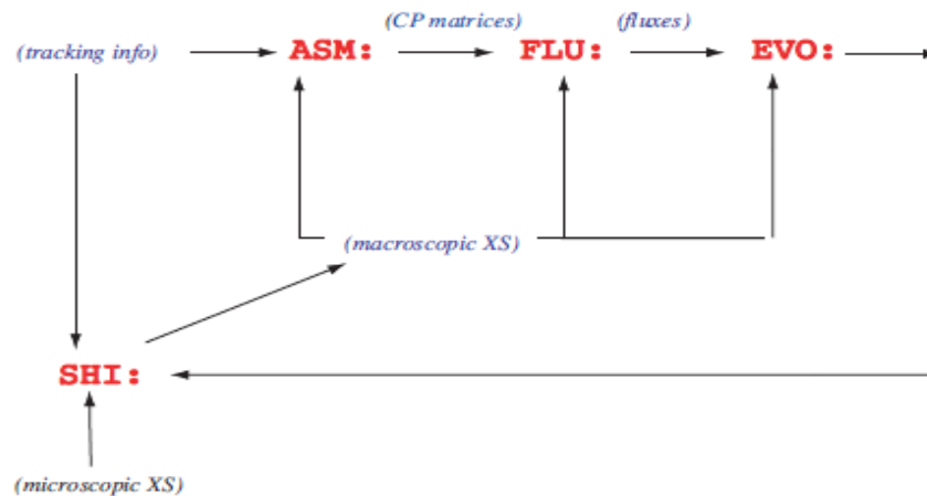
FIG 19. Secuencia de DRAGON, para ciclos de quemado [20].
