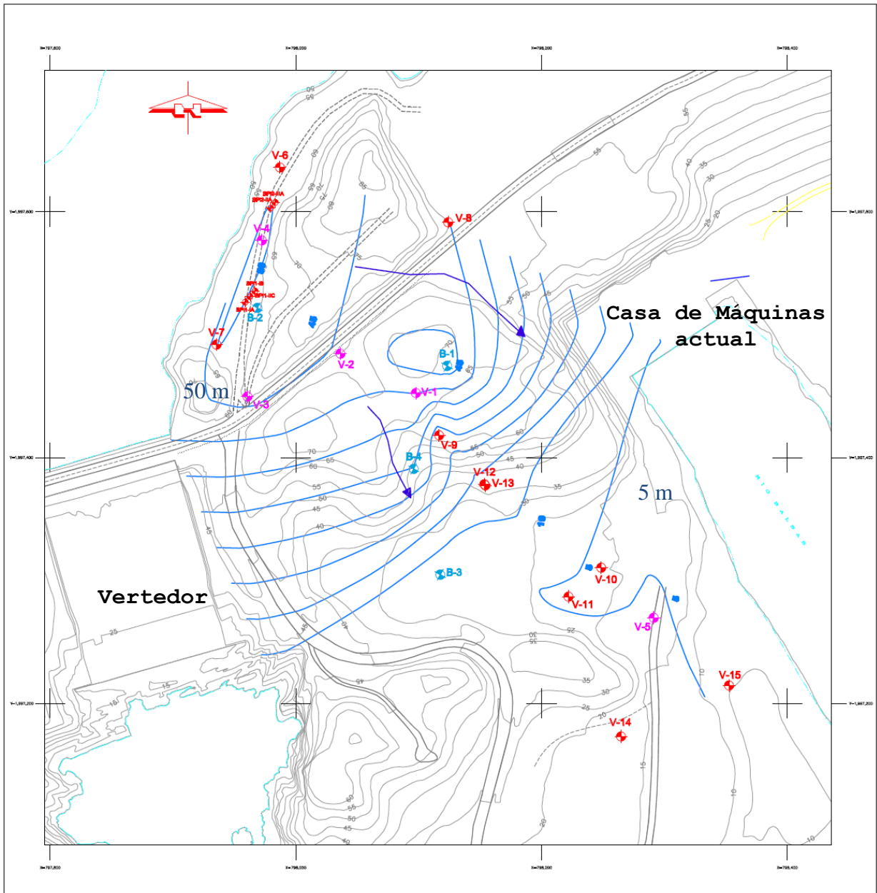
Figura III.5 - Niveles freáticos registrados en el mes de Agosto 2009.
