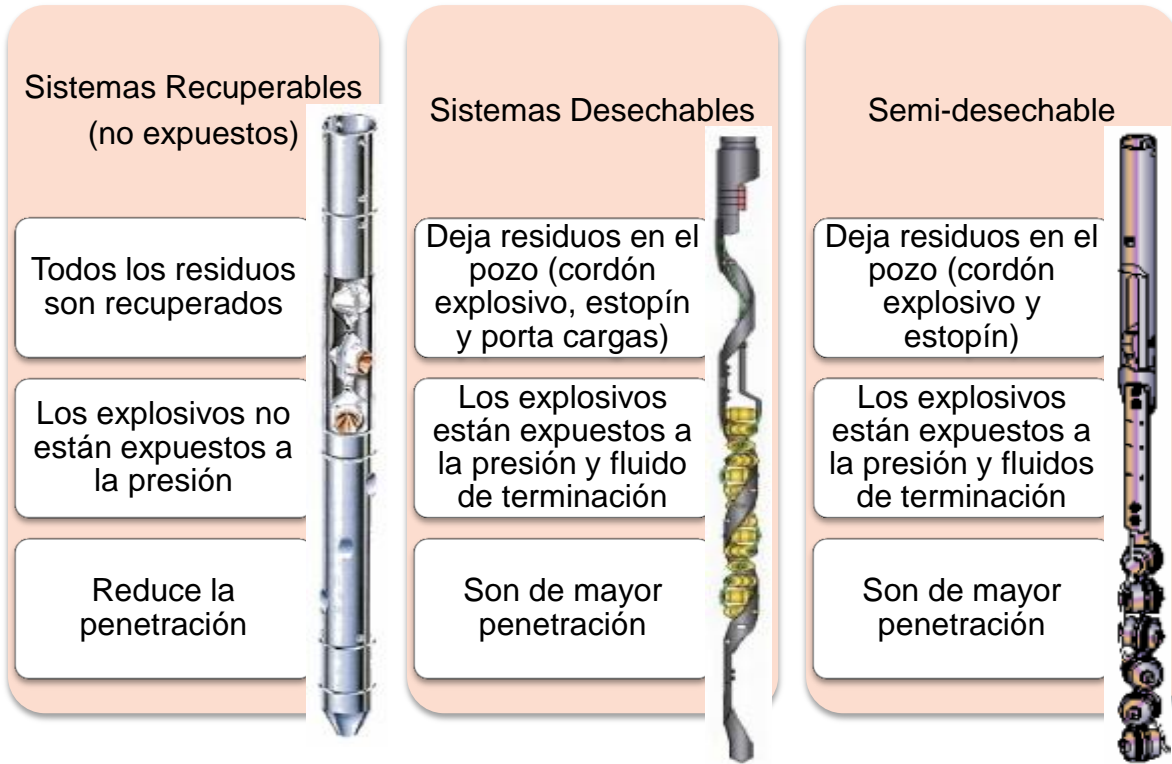
Figura 1.15 Sistemas de pistolas. 34
