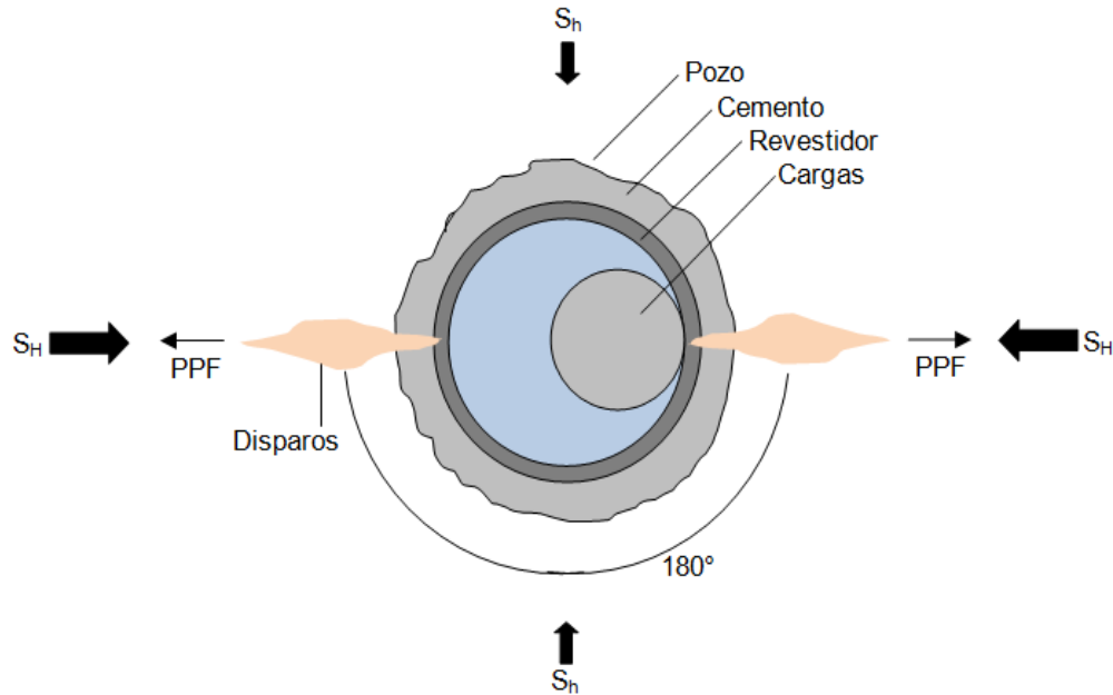
Figura 6.12 Fase de disparos de 180°. 10
