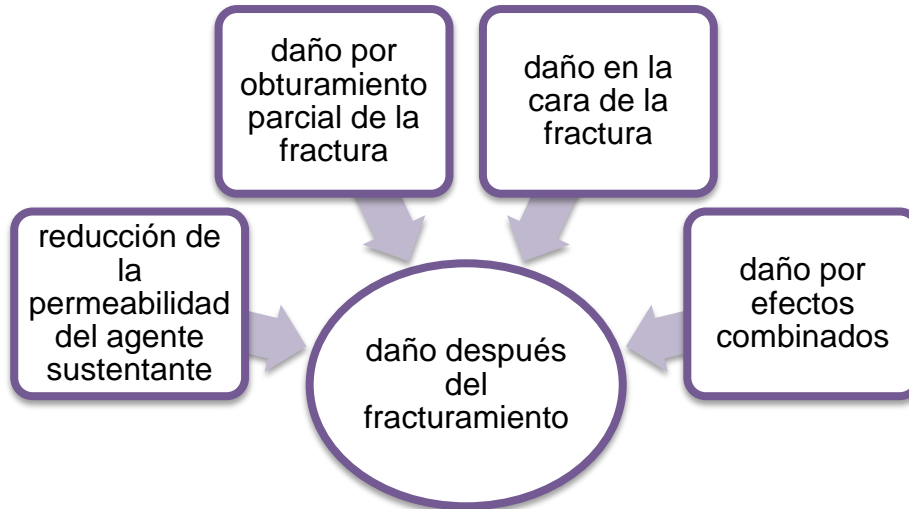
Figura 4.8 Tipos de daño.
