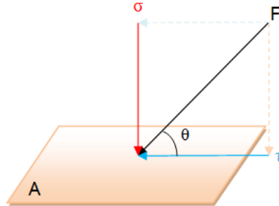
Figura 1.2 Vector de esfuerzo oblicuo.
