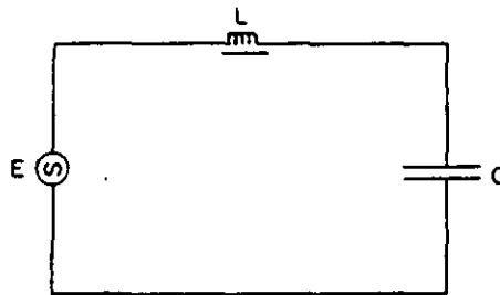
CIRCUITO TÍPICO FERORRESONANTE
