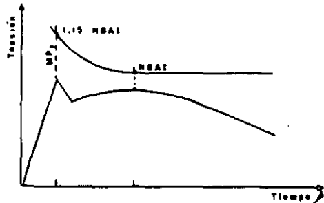
CURVA QUE MUESTRA LA COORDINACION DE LOS AISLAMIENTOS Y SU MARGEN DE PROTECCION.
