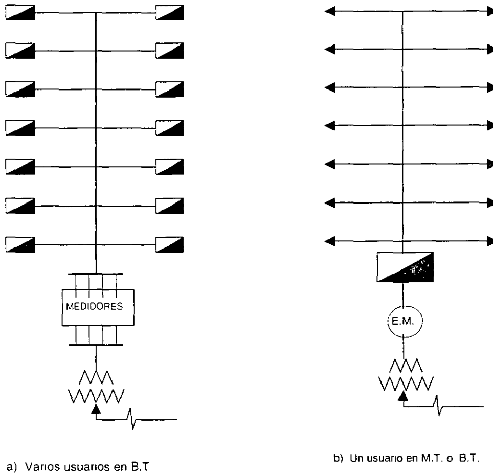
Figura 2.- Sistema radial para suministro de energía a edificios altos.
