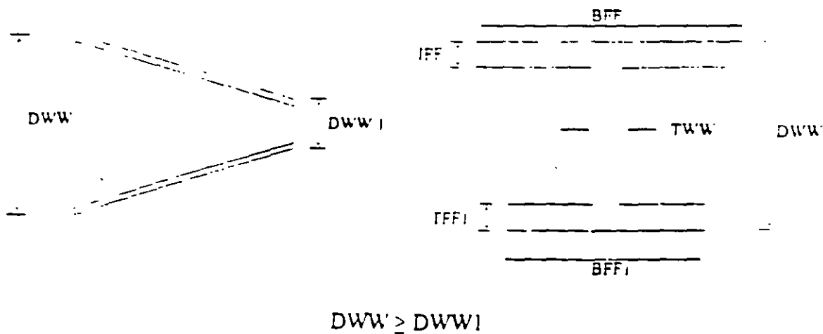
Figura 2.2 Caracteristicas de la seccion I de peralte variable
