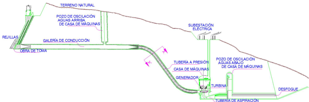
Figura 4.14 Perfil de obra de generación en caverna
