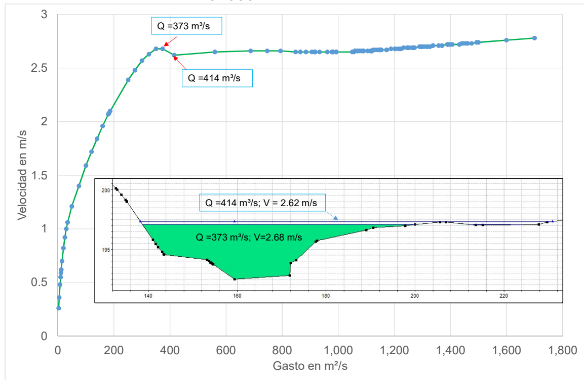
Figura 2.37 Sección transversal del cadenamiento 6+300 y comportamiento de su velocidad para diferentes gastos
