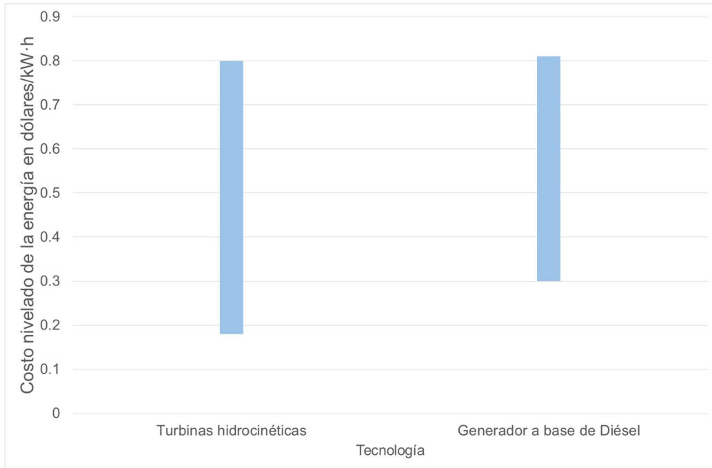
Figura 5.10 Rango de costos nivelados de la energía. Turbina hidrocinética vs generador a base de Diésel
