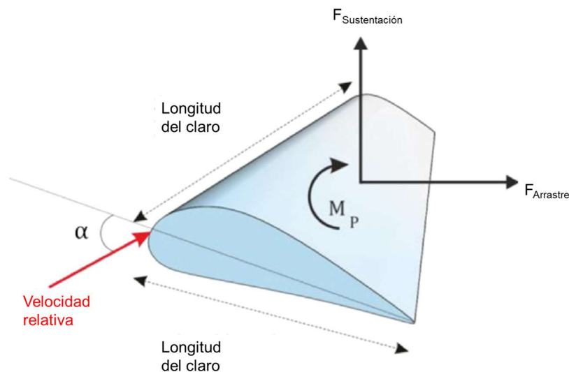
Figura 2.1 Fuerzas resultantes en una sección tipo de un álabes
