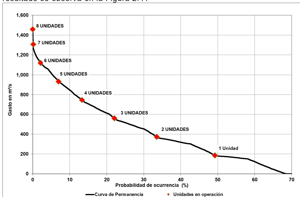
Figura 2.41 Permanencia de gastos turbinados de la C.H Chicoasén
