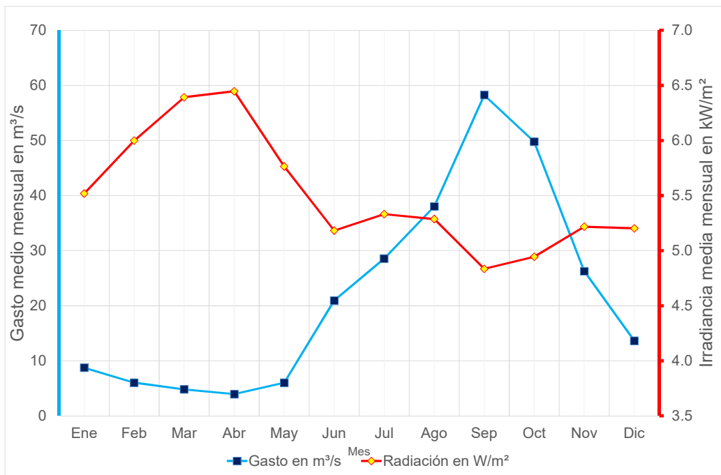
Figura 5.28 Gastos medios mensuales vs irradiancia mediamensual sobre sitio en el río Novillero
