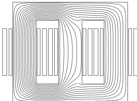
Figura 5.7: Distribución del flujo magnético ( \omega t = 0 ) a carga nominal.
