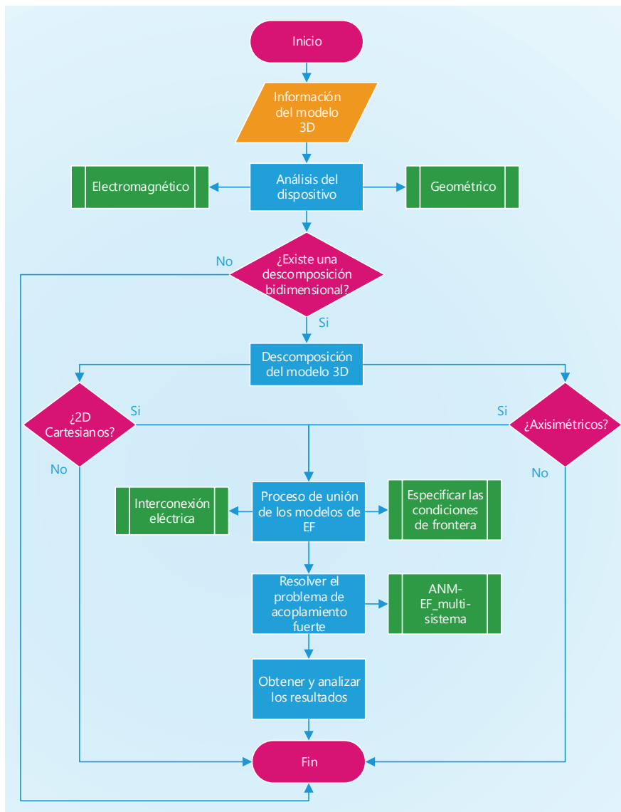
Figura 5.1: Diagrama de flujo del proceso mediante descomposición bidimensional.
