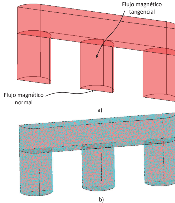
Figura F.1: Modelo 3D de EF: a) geometría y condiciones de frontera, b) mallado.
