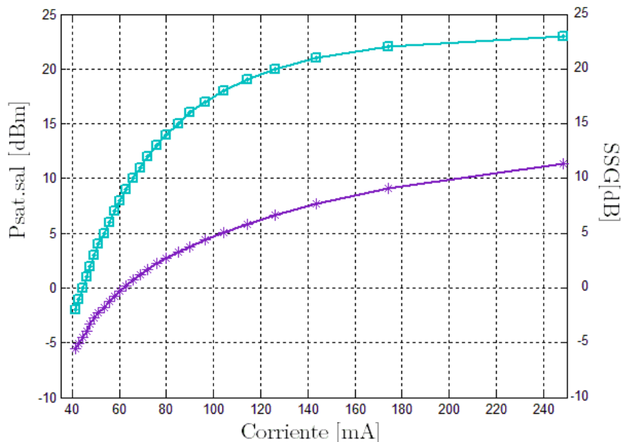
Figura 4.1 SSG (cuadros) y potencia de salida (asteriscos) como función de la corriente inyectada al SOA.
