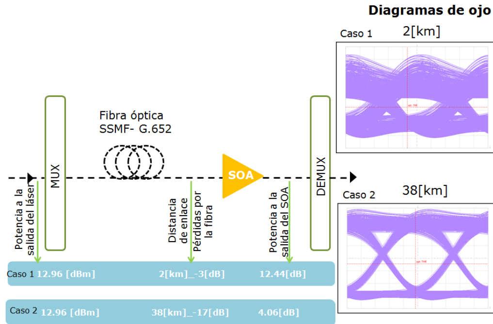
Figura 3.3.4 No linealidades en el SOA.
