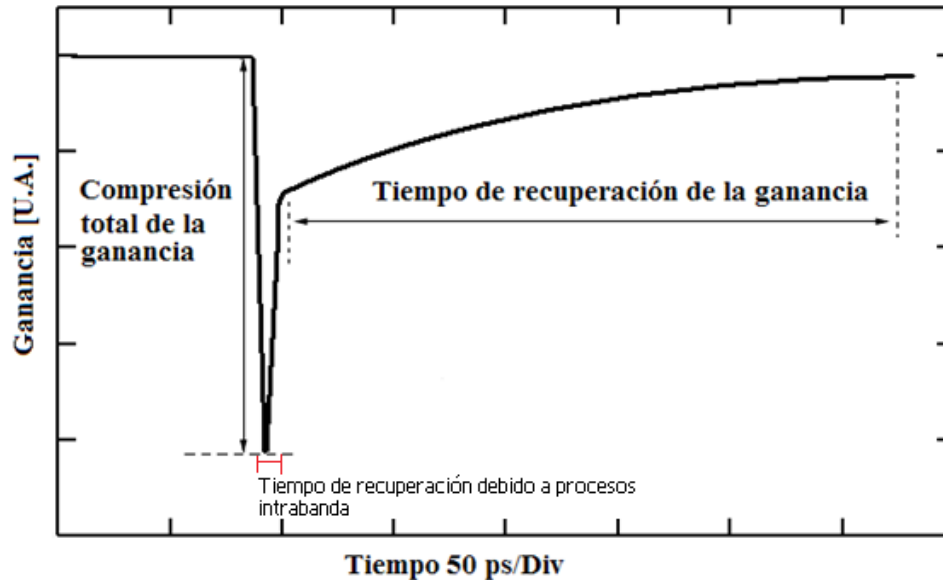
Figura 2.2.3 Tiempo de recuperación de la ganancia en un SOA.
