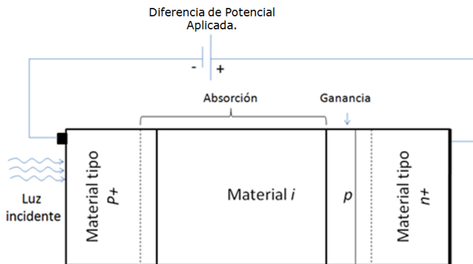
Figura 1.3.12 APD Fotodiodo de Avalancha.
