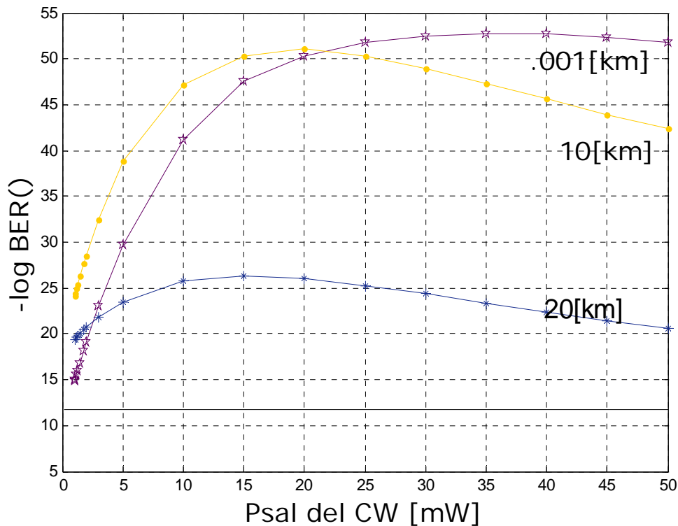
Figura 4.5 Tasa de bit en error vs P_{\text{sal}} del CW [dbm].
