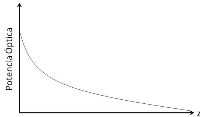
Figura 1.3.9 Comportamiento exponencial decreciente de la potencia óptica en función de la distancia dentro del foto-diodo.
