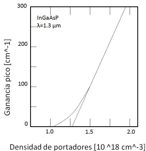
Figura 2.2.1 Gráfica de la ganancia pico vs densidad de portadores N.
