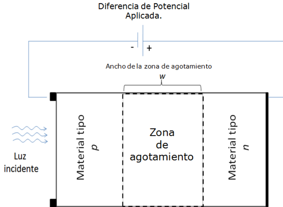
Figura 1.3.8 Esquema de un fotodiodo p-n (inyección inversa de corriente).
