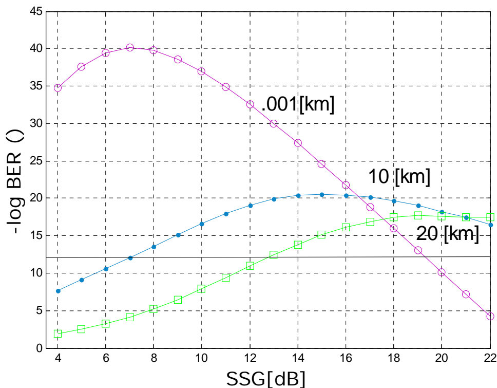
Figura 4.3 Tasa de bit en error -\log BER () vs SOA SSG [dB].
