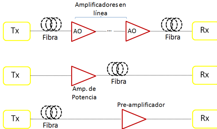
Figura 1.4.1 Aplicaciones de un Amplificador óptico. Amplificadores en línea, como un repetidor de un transmisor de potencia y como un preamplificador para el receptor.
