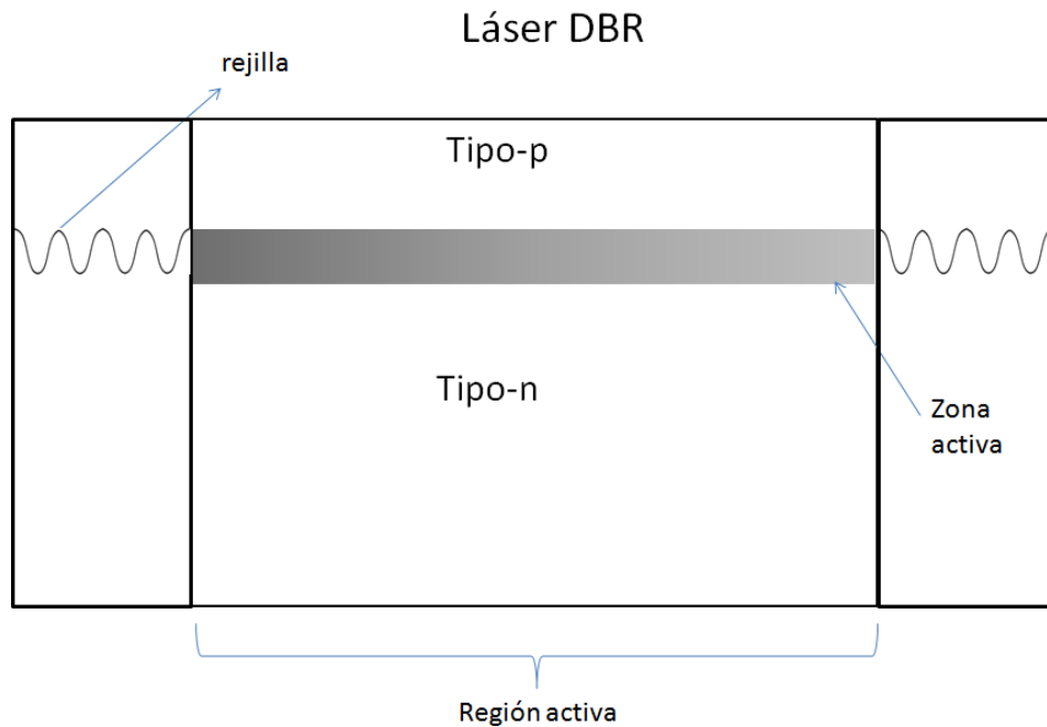
Figura 1.3.3 Estructura láser DBR.
