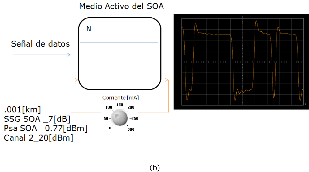
Figura 4.2 (a) Comportamiento de la señal al pasar por el SOA sin asistencia, (b) utilizando sistema de asistencia electrónico.
