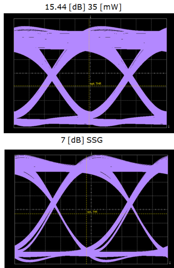
Figura 4.1.3 Diagramas de ojo de más alto desempeño para .001 [km]. Arriba esquema óptico, abajo esquema electrónico.
