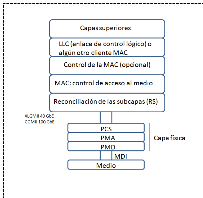
Figura 3.1.1 arquitectura típica de Ethernet.
