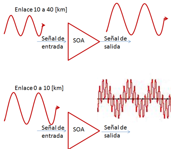
Figura 3.3.1 Comportamiento lineal del SOA (figura superior) y comportamiento no lineal (figura inferior).
