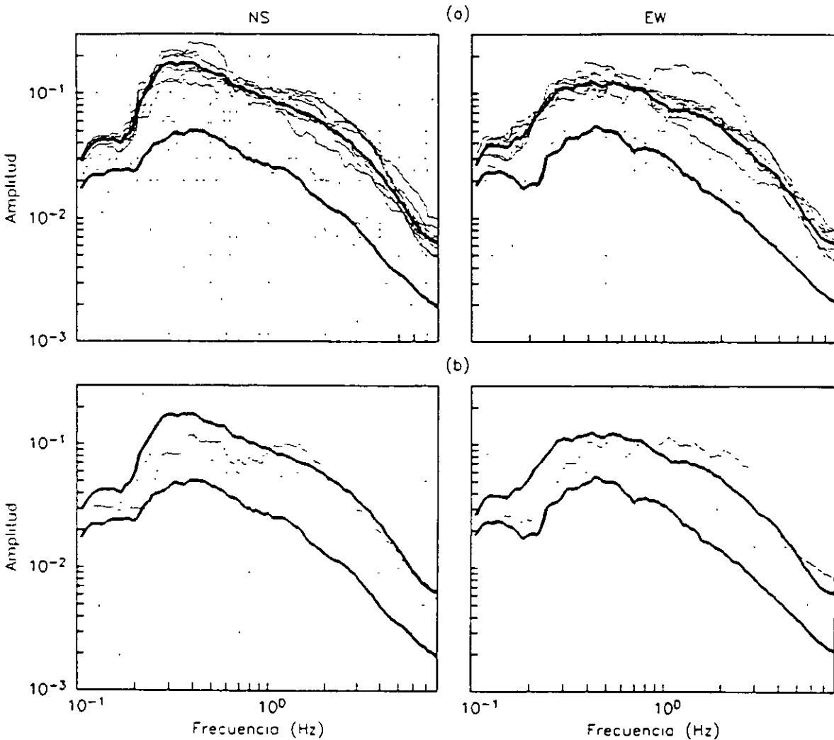
Fig 7. Espectros de Fourier en terreno firme para el sismo del 14 de septiembre de 1995. (a) Espectros de sitios localizados en el sur y suroeste (líneas superiores) y en el norte de la ciudad (líneas inferiores). Con trazo grueso se muestran los espectros promedio para ambos grupos, (b) Espectros promedio y de estaciones en sitios intermedios (18 y 28)
