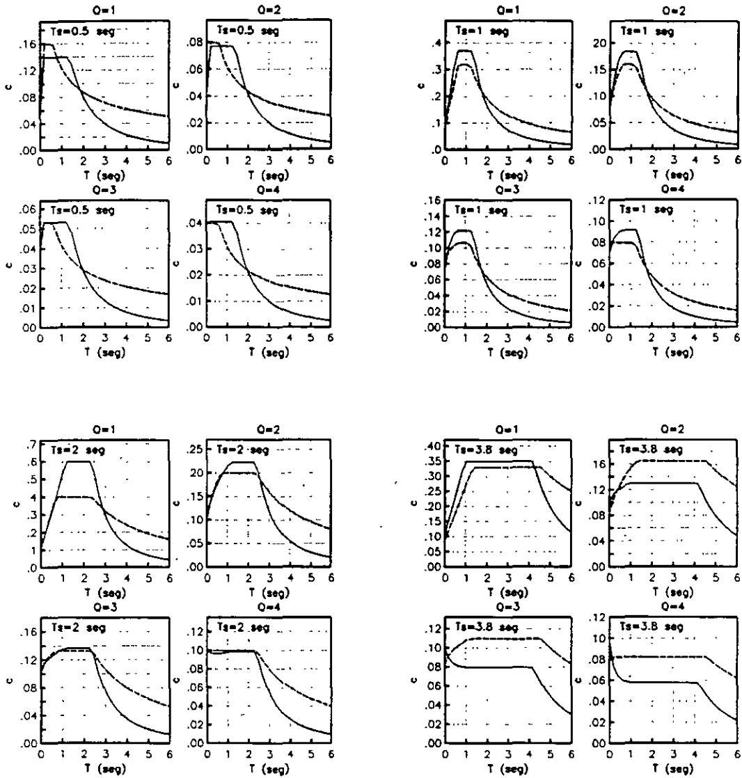
Figura 8. Espectros de diseño (resistencia necesaria) para sitios con diversos periodos predominantes del suelo, T_s , y para varias ductilidades. Línea continua (negra): espectros propuestos en el presente trabajo; línea discontinua (roja) espectros obtenidos del apéndice A4 de las Normas Técnicas Complementarias para Diseño por Sismo vigentes en el DF
