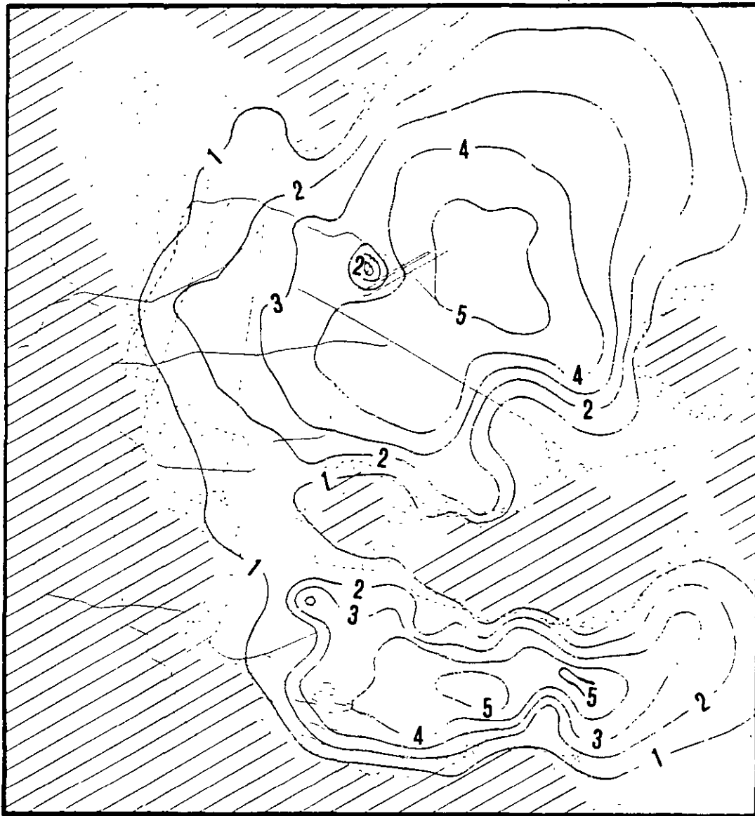
Fig 13. Mapa de la ciudad de México con curvas de igual periodo basada en datos de sismos y de vibración ambiental
