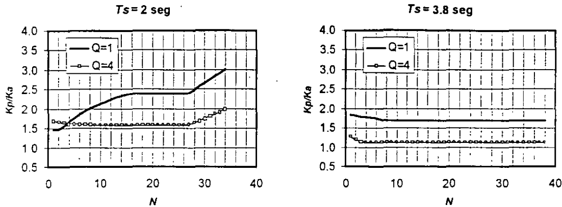
Figura 11. Relación entre la rigidez mínima requerida en la presente propuesta, K_p , y la rigidez requerida por las NTC vigentes utilizando el apéndice A4, K_r . Se presentan los casos de T_s=2 y 3.8 seg, y ductilidades, Q , de 1 y 4, para distintos valores de N , el número de pisos. Las distorsiones permisibles son: en la propuesta que se hace, 0.015 al colapso y 0.004 en servicio; para las NTC vigentes, 0.012.
