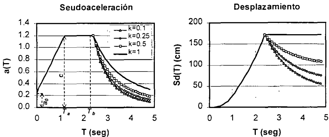
Figura 3 Formas características de los espectros de peligro uniforme suavizados, tanto de pseudoaceleración como de desplazamiento. Nótese la variación de las ordenadas para T > T_b dependiendo del parámetro k .
