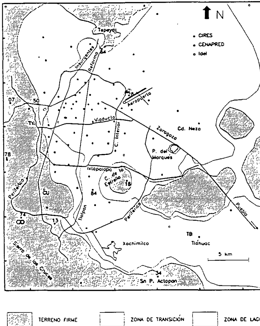
Fig 2 El valle de México: zonas geotécnicas, sitios de referencia y estaciones acelerométricas utilizadas en este trabajo
