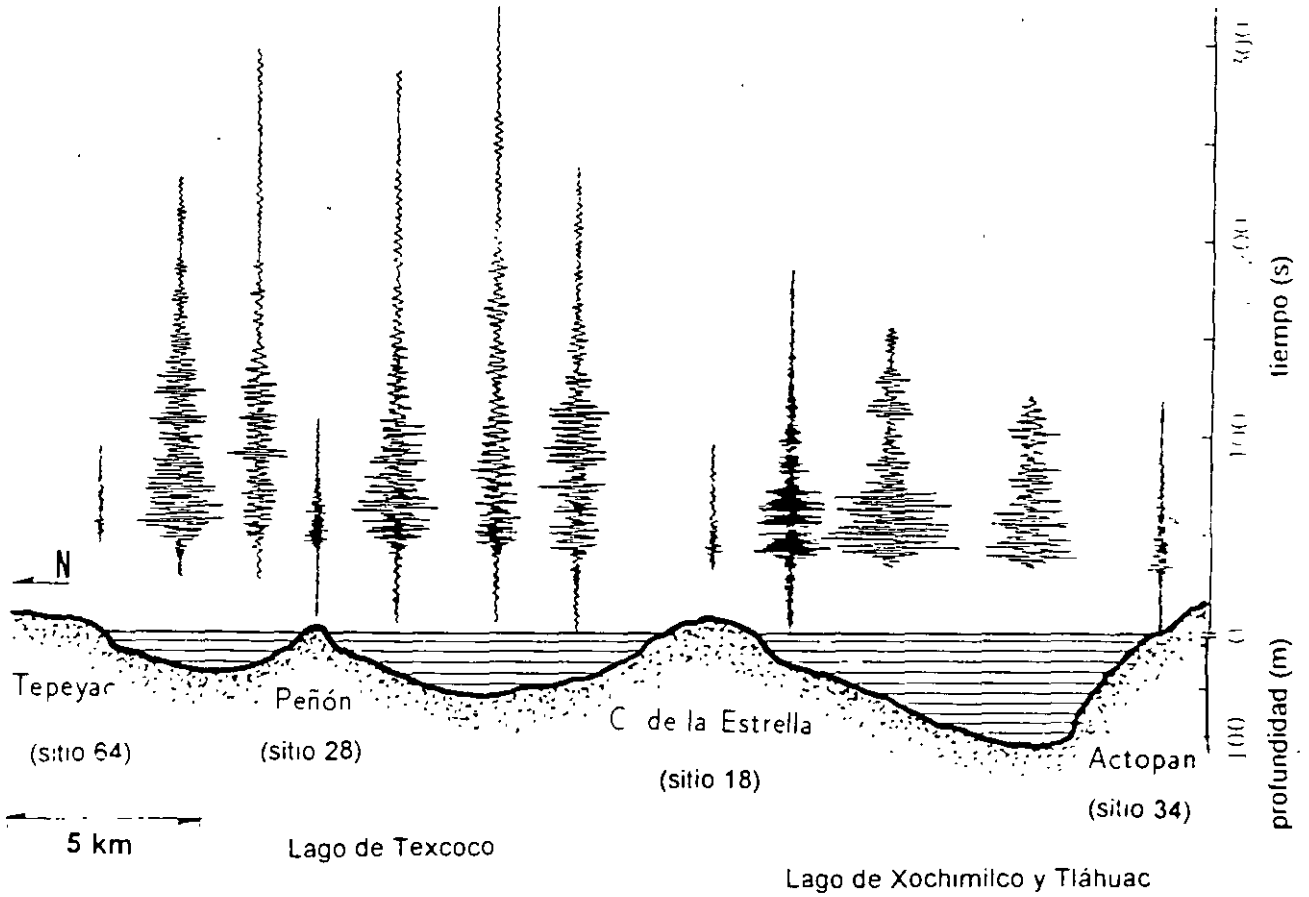
Fig 10. Aceleraciones del terreno en una sección norte-sur del valle (B-B' en la figura 2) para el sismo del 25 de abril de 1989, componente norte-sur
