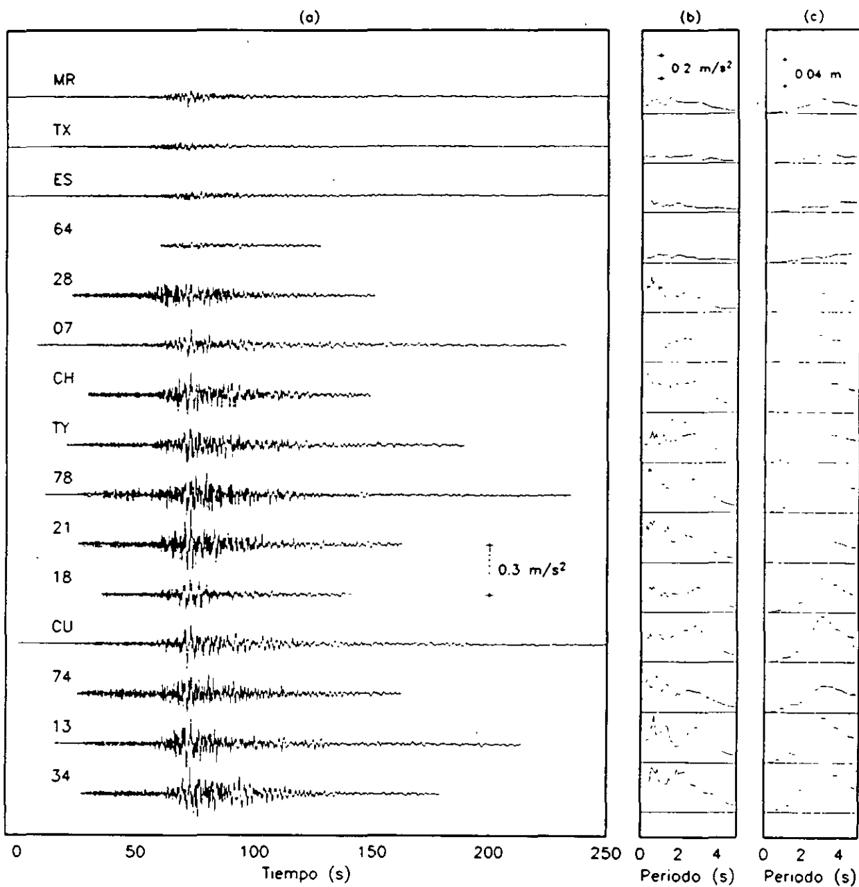
Fig 5. Movimiento en terreno firme en la ciudad de México durante el sismo del 14 de septiembre de 1995, componente norte-sur: (a) Acelerogramas, (b) Espectros de respuesta de aceleración. (c) Espectros de respuesta de desplazamiento
