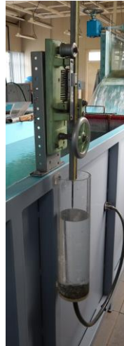
c) Limnómetro de punta
