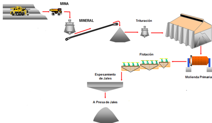
Figura 1. Diagrama de flujo del proceso de mineral y generación del jal (Grupo México)
