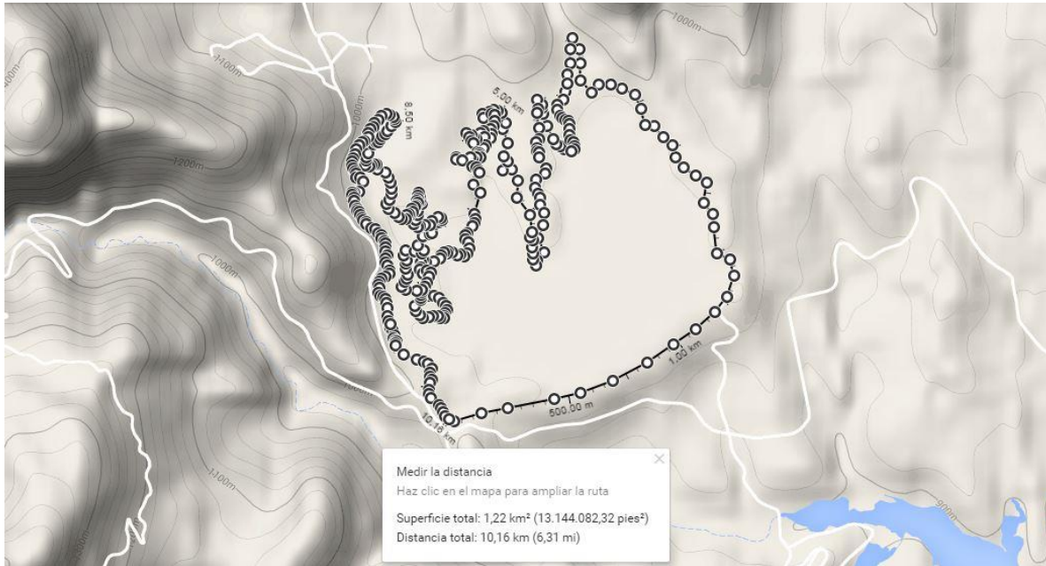
Figura 41. Delimitación del depósito de jales.
