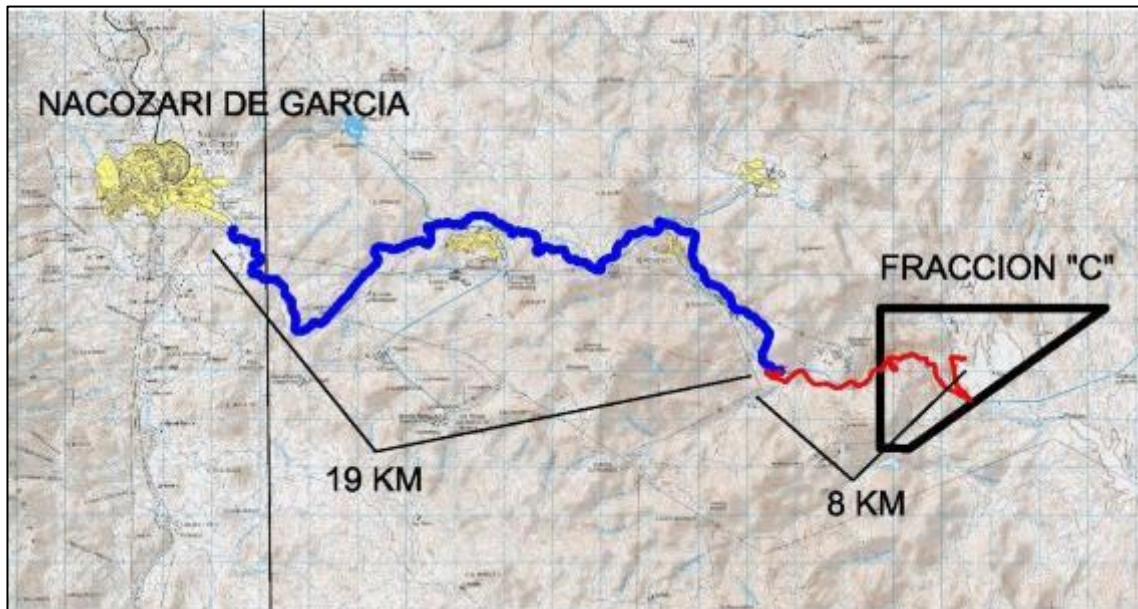
Figura 20. Vías de acceso hacia el depósito de jales 1-2-3.
