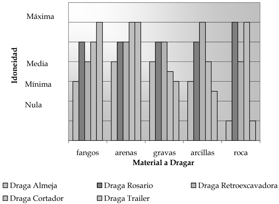
Figura 2.10. Idoneidad de varios tipos de dragas.
