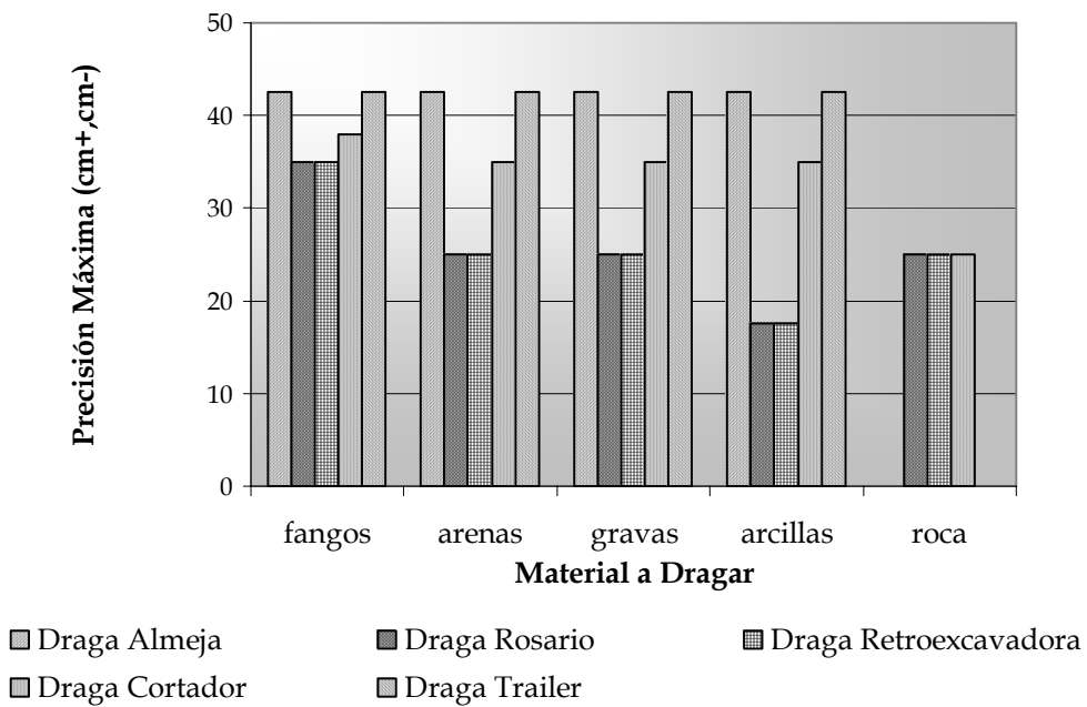
Figura 2.11. Precisión máxima de varios tipos de dragas.
