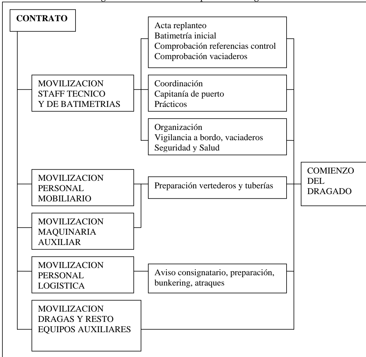
Figura 4.4. Actividades previas al dragado.
