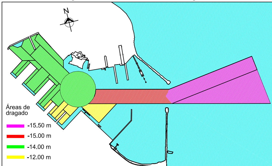
Figura 6.2. Distribución de áreas de dragado.
