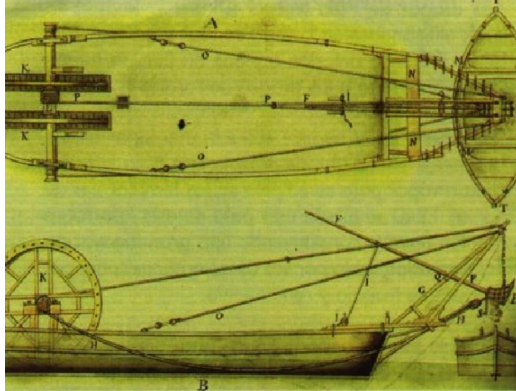
Figura 1.2. Proyecto de una máquina con una sola pala para dragar, diseñada para el Puerto de Ceuta.
