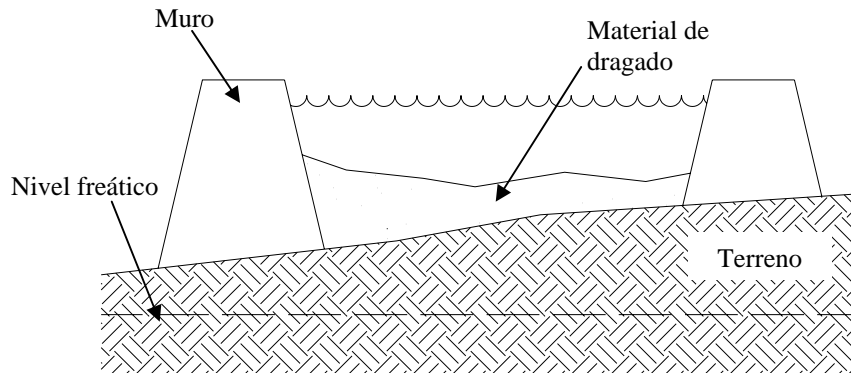
Figura 5.3. Esquema recinto en tierra.
