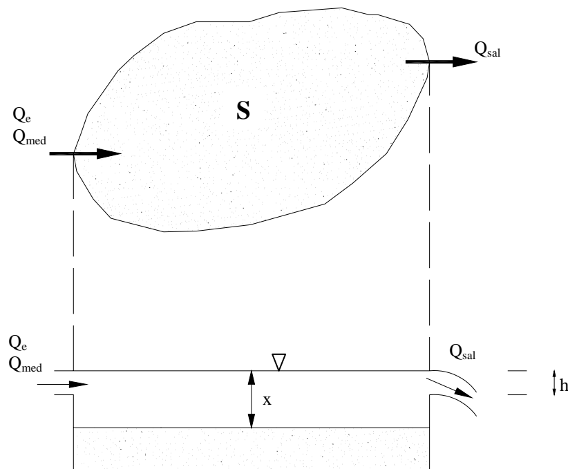
Figura 5.9. Esquema teórico de un recinto.
