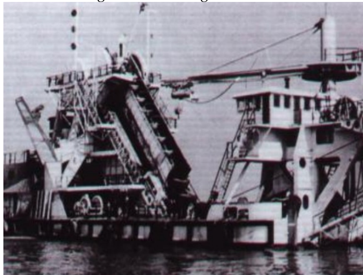
Figura 1.4. Draga de rosario.
