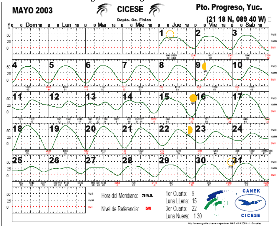
Figura 3.4. Registro de mareas.
