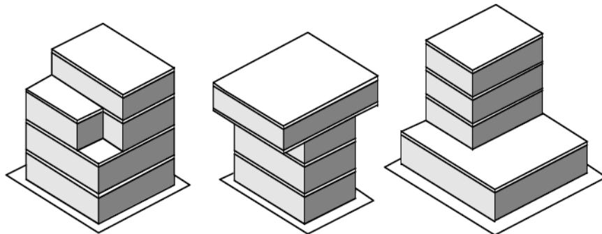
Figura 4.4 Formas irregulares en elevación
