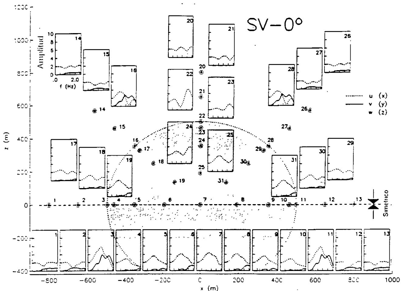
Fig 9 Amplificación en la superficie de una montaña tridimensional en forma de domo para incidencia vertical de ondas SV
