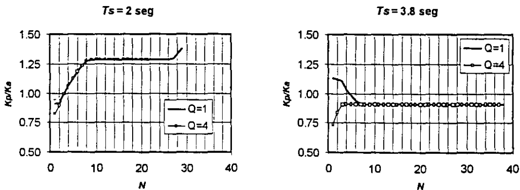
Figura 10. Relación entre la rigidez mínima requerida en la presente propuesta, K_p , y la rigidez requerida por las NTC vigentes utilizando el apéndice A4, K_o . Se presentan los casos de T_s=2 y 3.8 seg, y ductilidades, Q , de 1 y 4, para distintos valores de N , el número de pisos. Las distorsiones permisibles son: en la propuesta que se hace, 0.030 al colapso y 0.004 en servicio; para las NTC vigentes, 0.012.
