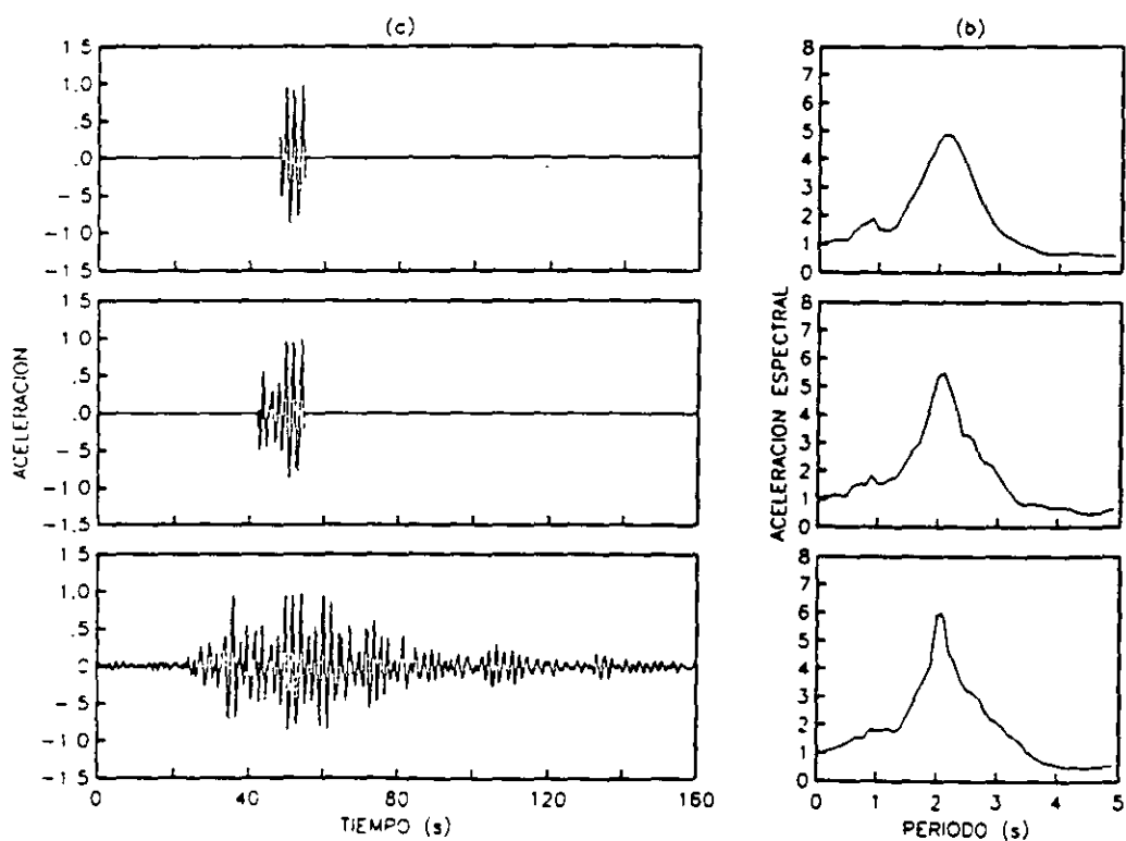
Fig 15. Registro del componente norte-sur del sismo del 19 de septiembre de 1985 en el sitio SC (Secretaria de Comunicaciones y Transportes) y espectros de respuesta calculados con distintas partes del registro
