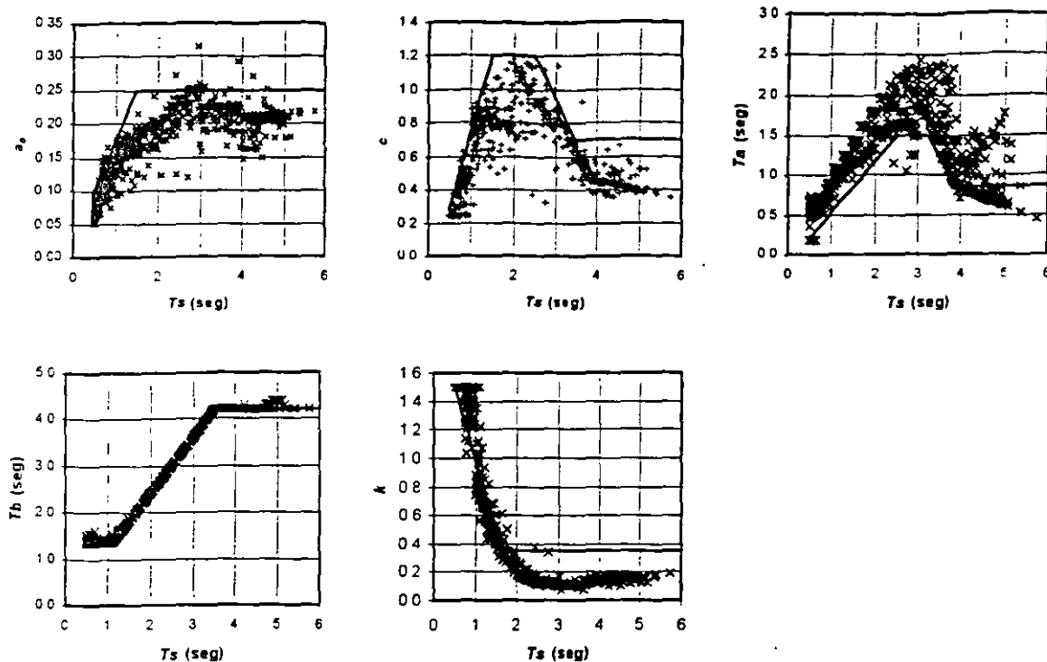
Figura 4 Puntos: relación entre los parámetros que definen los espectros de peligro uniforme suavizados y el periodo predominante del suelo, T_s . Líneas rectas: ajustes propuestos para especificar espectros de diseño.
