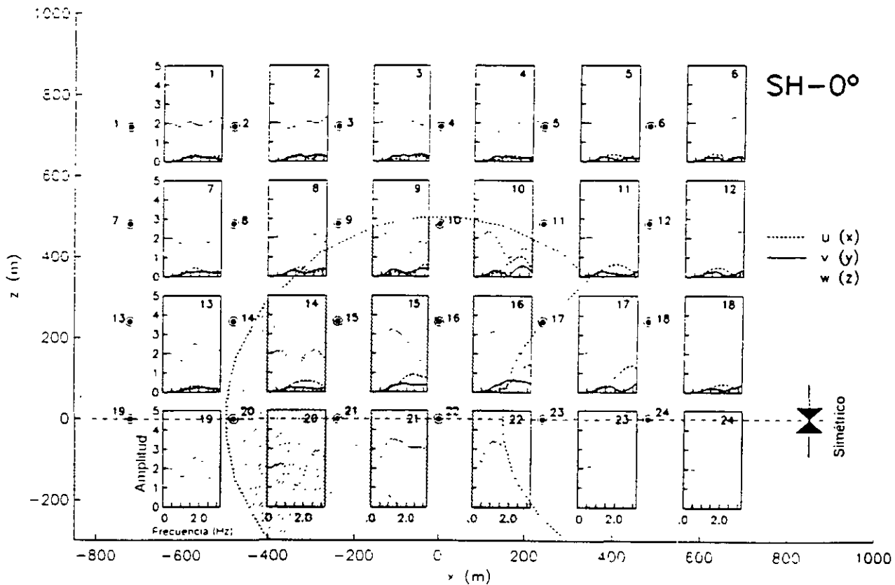
Fig 12 Amplificación en la superficie de la montaña tridimensional en forma de herradura ante incidencia vertical de ondas SH
