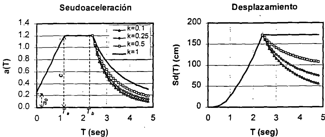
Figura 3. Formas características de los espectros de peligro uniforme suavizados, tanto de seudoaceleración como de desplazamiento. Nótese la variación de las ordenadas para T > T_b , dependiendo del parámetro k
