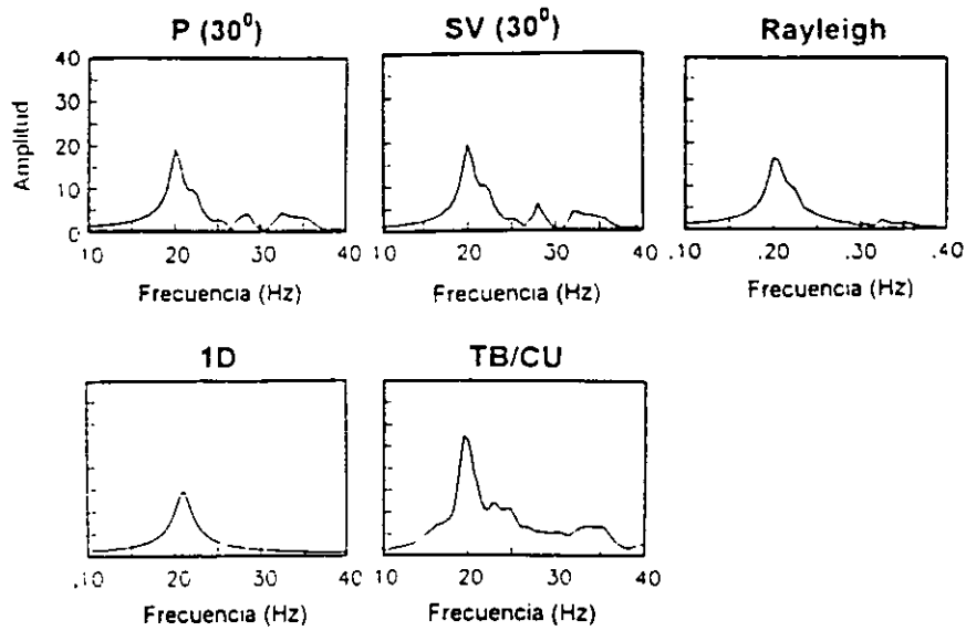
Fig 6 De izquierda a derecha: funciones de trasferencia calculadas para ondas P, SV y Rayleigh, función de trasferencia unidimensional y cociente espectral entre TB y CU
