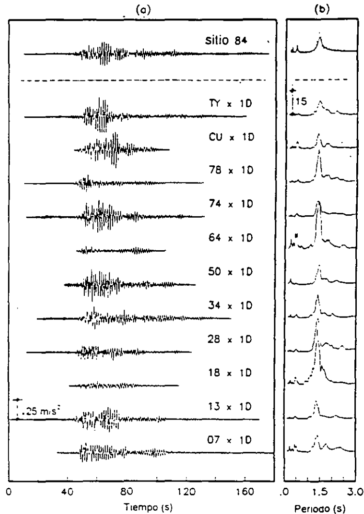
Fig 3 Componente norte-sur del sismo del 25 de abril de 1989: (a) Registro en el sitio 84 (arriba) y respuestas 1D en el tiempo usando once sitios en zona I como referencia: (b) Con línea continua el cociente espectral promedio y con línea punteada la función de trasferencia unidimensional (arriba) y cocientes espectrales entre cada registro de referencia y la estación 84
