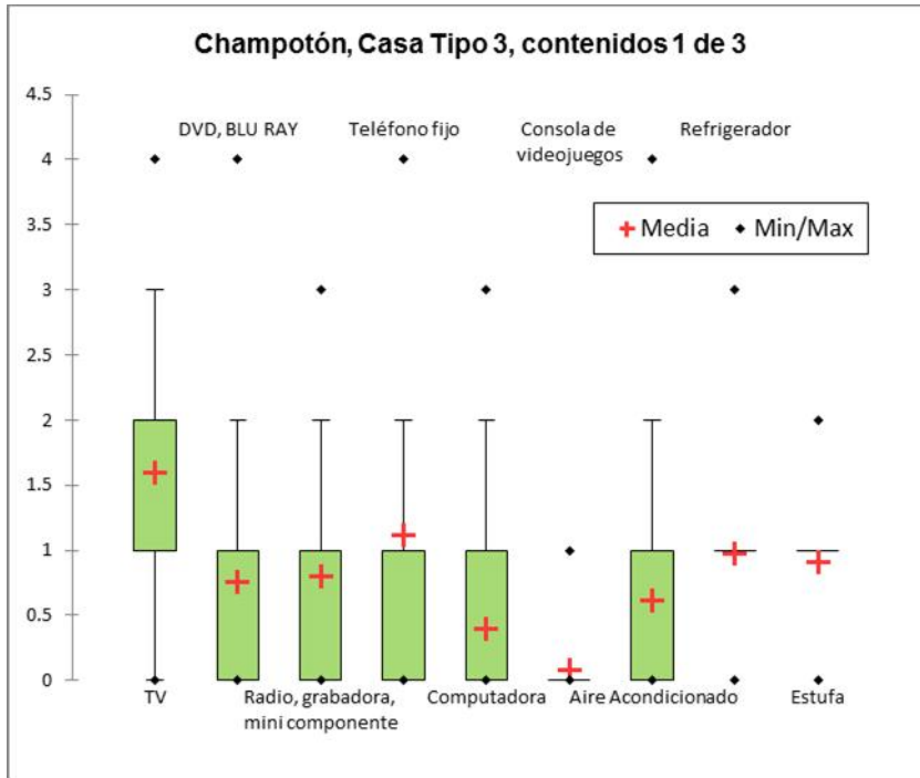
Figura 38. Contenidos parciales para vivienda tipo 3, ciudad de Champotón
