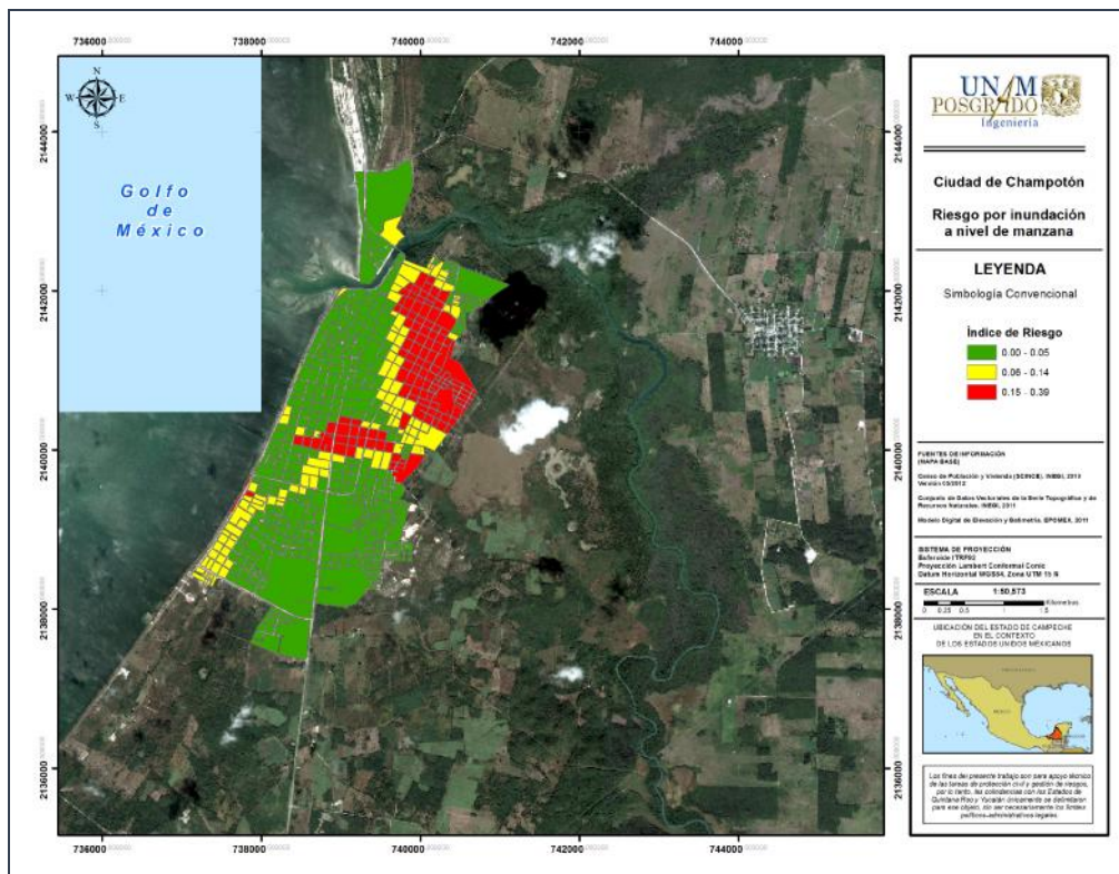
Figura 54. Índice de riesgo desbordamiento del Río Champotón en la ciudad de Champotón
