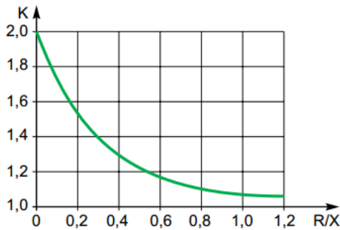
Figura 5.3a Variación del factor k en función de la relación X/R
