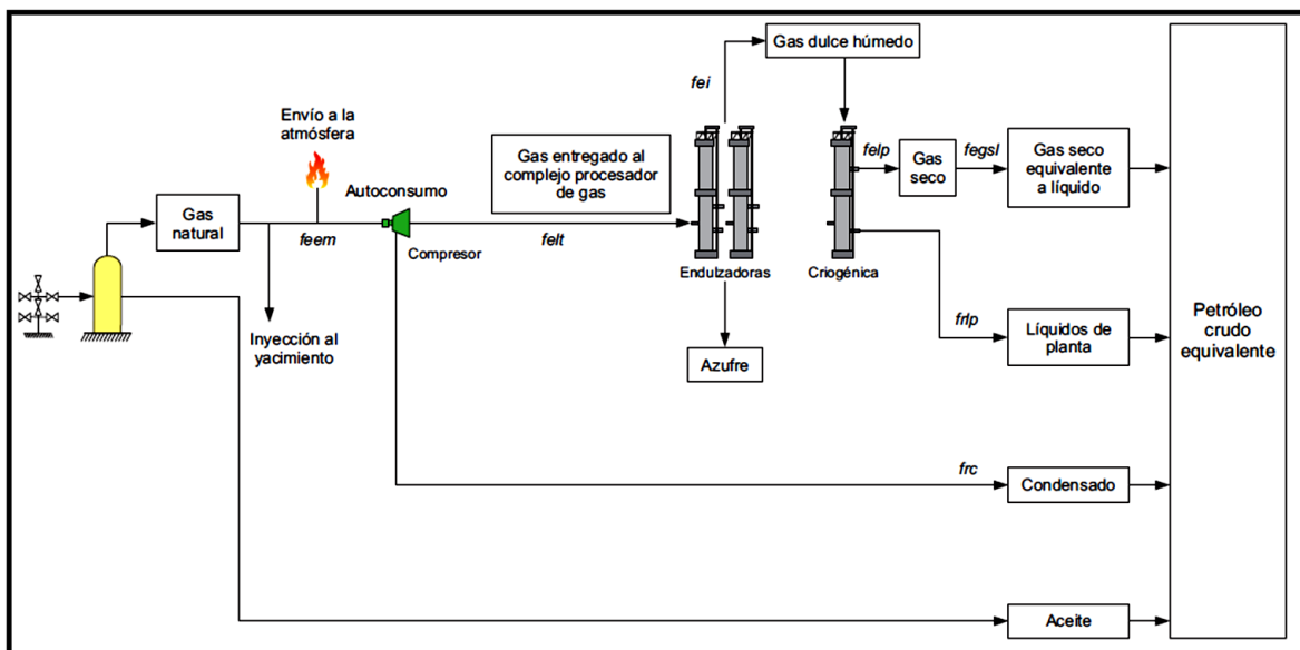
Figura 5.7-1. Elementos para el cálculo del Petróleo Crudo Equivalente, en todo el circuito desde la boca del pozo hasta el centro procesador de gas. En función de la eficiencia de operación de cada etapa será la magnitud del factor de rendimiento o encogimiento.
