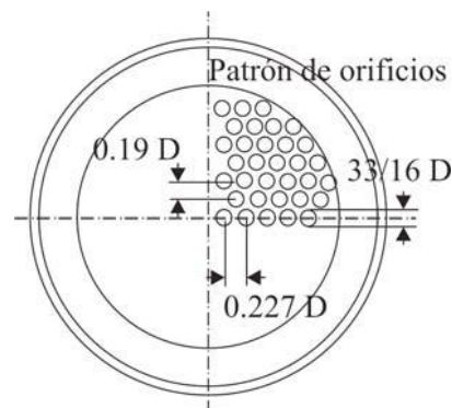
Figura 2. Diseño genérico del plato rompedor [18].
