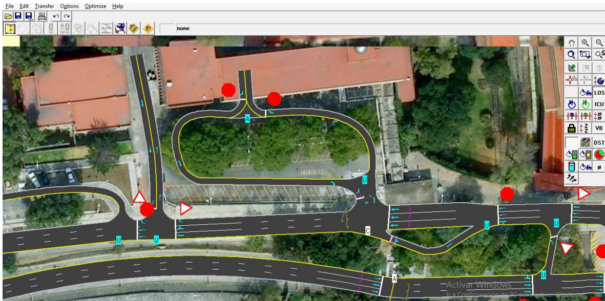
Ilustración 47 Niveles de servicio, solución 1
