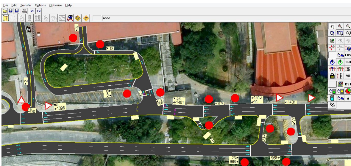
Ilustración 38 Sentidos y volúmenes vehiculares, estado actual en Syncro 7
