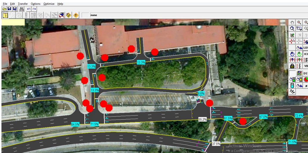
Ilustración 68 Capacidad de la vía
