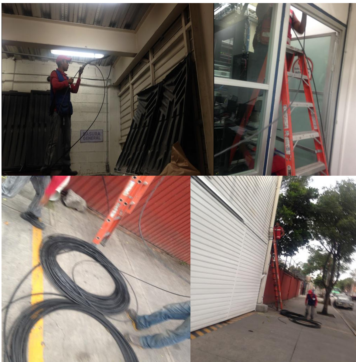
Fotografía 4.2.5b Tendido e instalación de fibra óptica hasta site de nave 3
