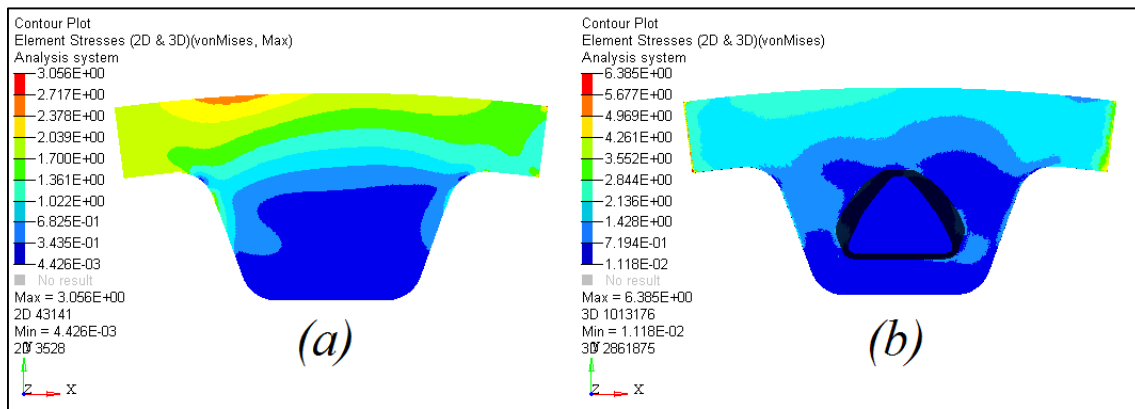
Figura 4.10. Distribución de esfuerzos, en megapascales (MPa), para las cargas T_1 y F_1(45.7521^\circ) . (a) Antes de la optimización. (b) Después de la optimización.
