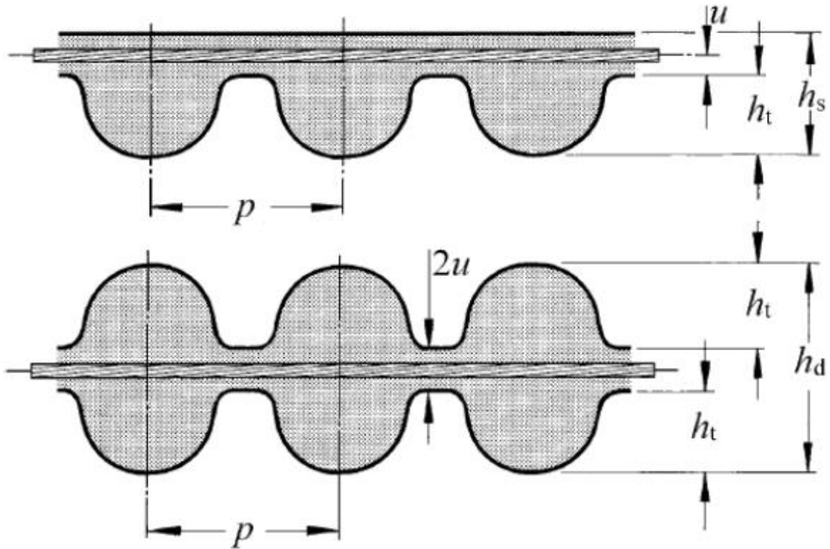
Figura 1.3. Bandas dentadas con dientes de perfil parabólico HTD; acotándose el paso p , el valor u , la altura de un solo diente h_t y la altura total de la banda h_s o h_d , bien sea banda dentada sencilla ( s ), o bien sea banda dentada doble ( d ) [1].
