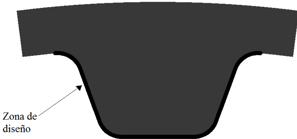
Figura 3.14. Zona de diseño para optimización de forma del diente XXH.
