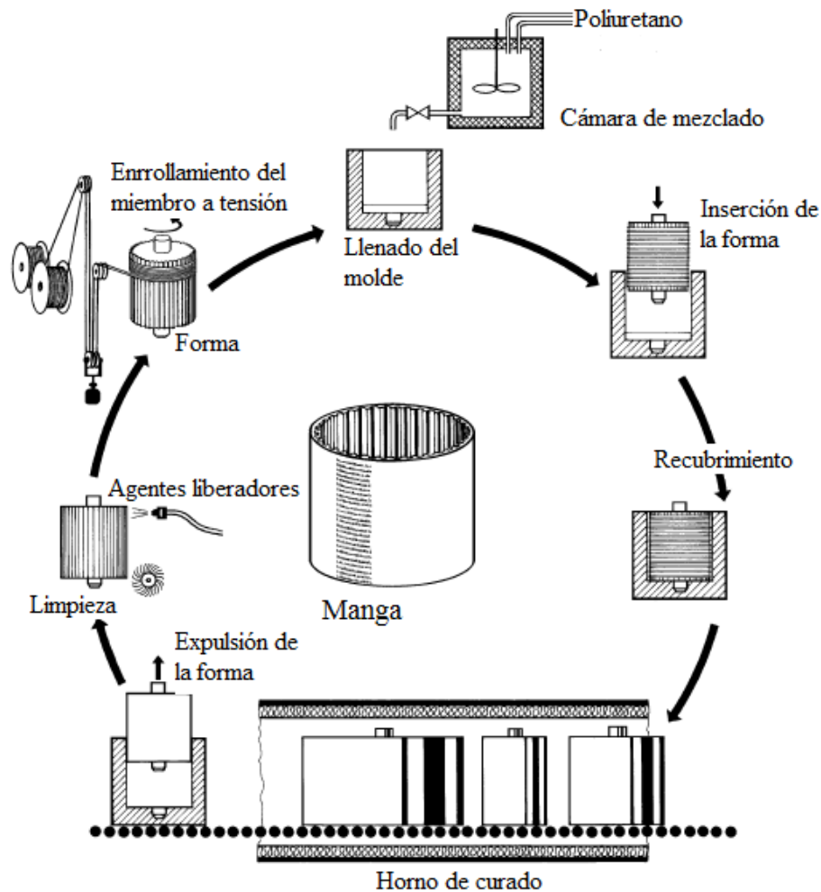
Figura 2.2. Fabricación de las bandas por fundición [6].
