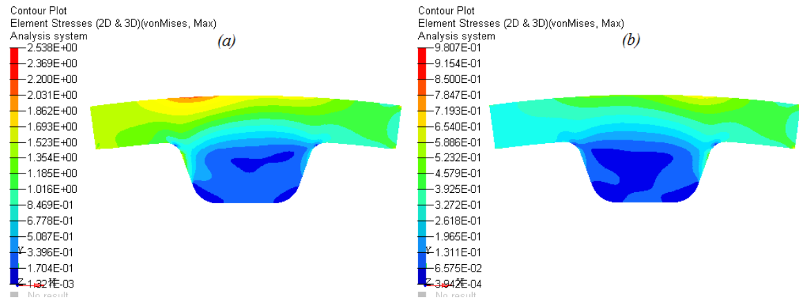
Figura 3.8. Distribución de esfuerzos, en megapascales (MPa), para (a) T_1 y F_1(46.70^\circ) , (b) T_2 y F_{1,b}(46.70^\circ) .
