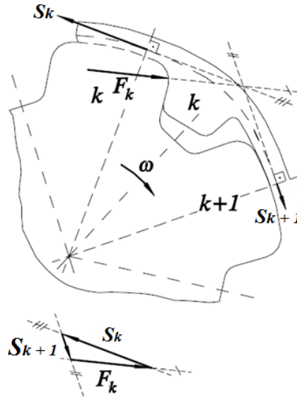
Figura 2.6. Cargas que actúan en el k -ésimo diente de una banda [7].
