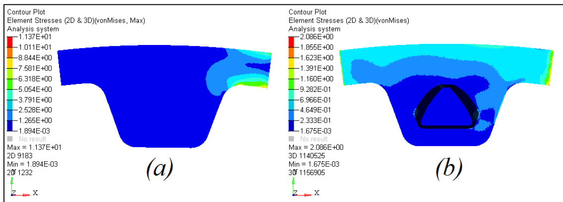
Figura 4.11. Distribución de esfuerzos, en megapascales (MPa), para las cargas T_2 y F_{1,b}(45.7521^\circ) . (a) Antes de la optimización. (b) Después de la optimización.
