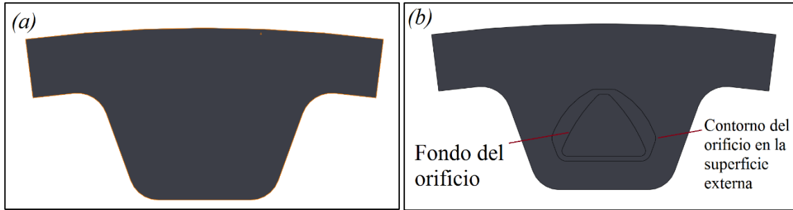
Figura 4.9. (a) Diente XXH antes de la optimización. (b) Diente XXH después de la optimización.
