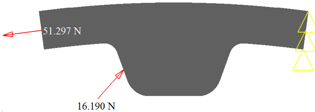
Figura 3.3. (c) Cargas aplicadas en el diente L cuando \gamma = 48.71^\circ .
