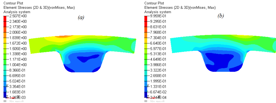
Figura 3.7. Distribución de esfuerzos, en megapascales (MPa), para (a) T_1 y F_1(44.60^\circ) , (b) T_2 y F_{1,b}(44.60^\circ) .
