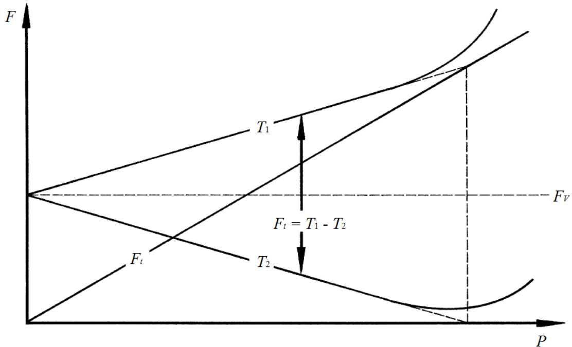
Figura 2.5. Fuerzas como función de potencia [6].
