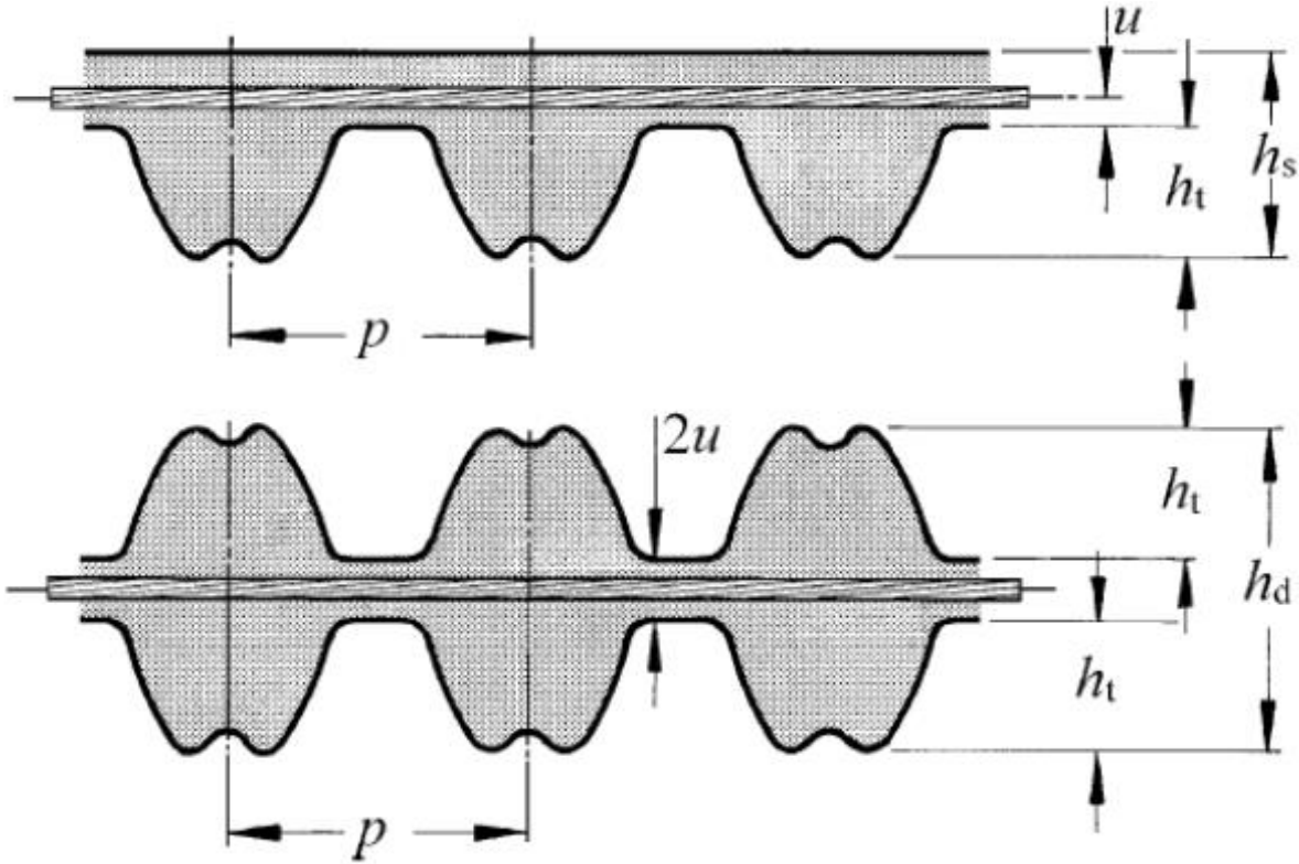
Figura 1.4. Bandas dentadas con dientes de doble perfil parabólico RPP; acotándose el paso p , el valor u , la altura de un solo diente h_t y la altura total de la banda h_s o h_d , ya sea banda dentada sencilla ( s ), o sea banda dentada doble ( d ) [1].
