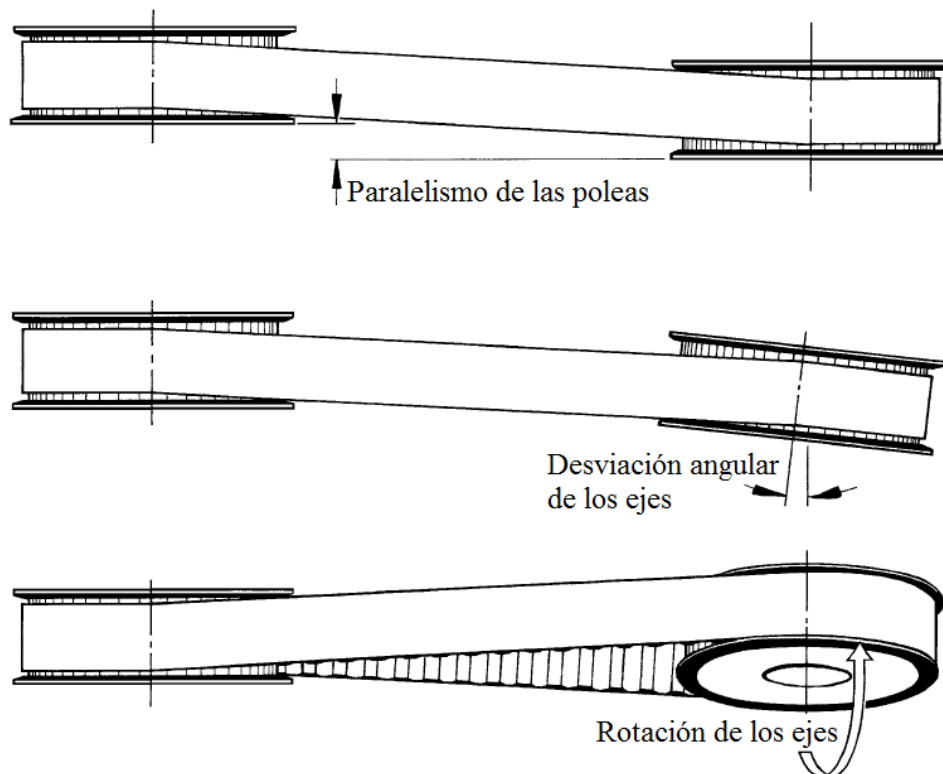
Figura 2.7. Desalineación de los ejes [6].
