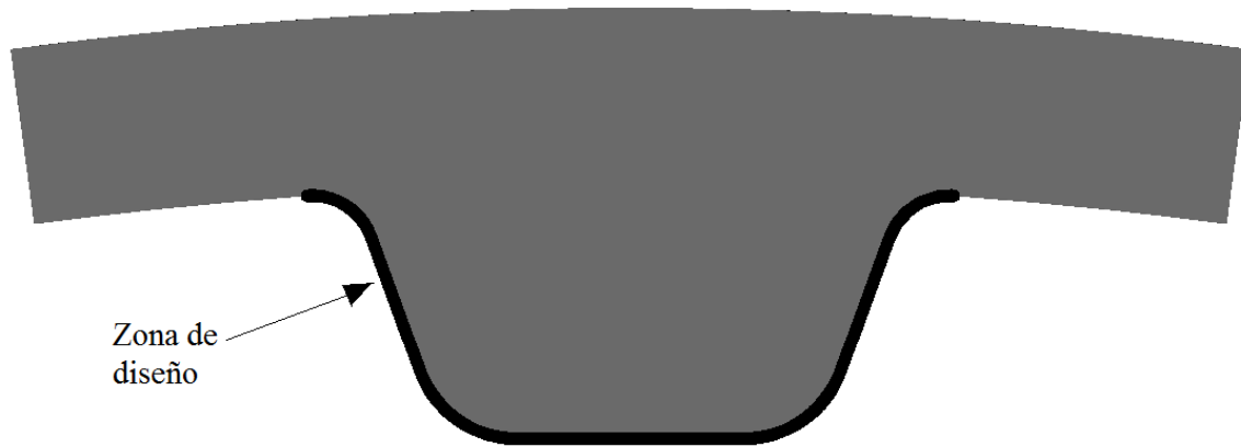
Figura 3.13. Zona de diseño para optimización de forma del diente L.
