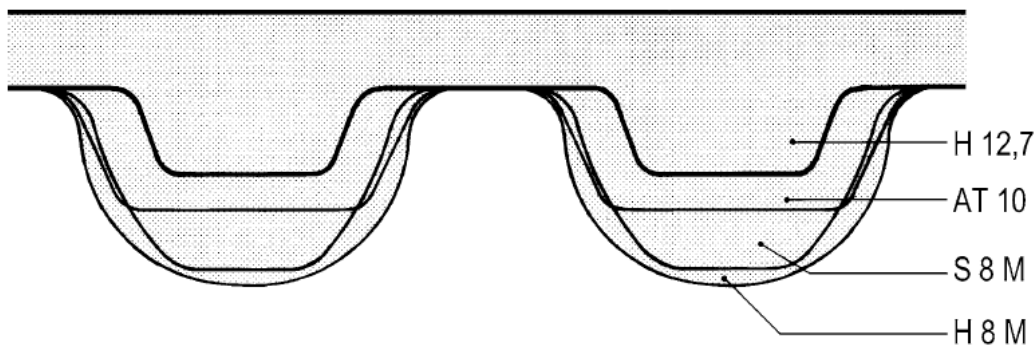
Figura I.1. Comparación de la altura del diente entre distintos modelos de bandas [1].
