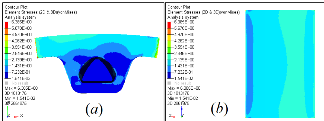
Figura 4.5. Vista frontal (a) y vista superior (b) de las distribuciones de esfuerzos de von Mises (en unidades de MPa) para la fuerza F_1(49.4973^\circ) aplicada en el flanco izquierdo del diente. En la vista superior se puede apreciar que la distribución de esfuerzos en el ancho de la banda es simétrica y, por lo tanto, la banda no abandonará la polea (sección 2.6).
