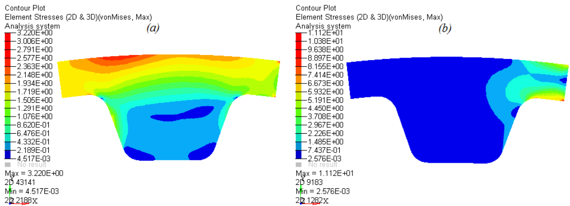
Figura 3.12. Distribución de esfuerzos, en megapascales (MPa), para (a) T_1 y F_1(52.9871^\circ) , (b) T_2 y F_{1,b}(52.9871^\circ) .
