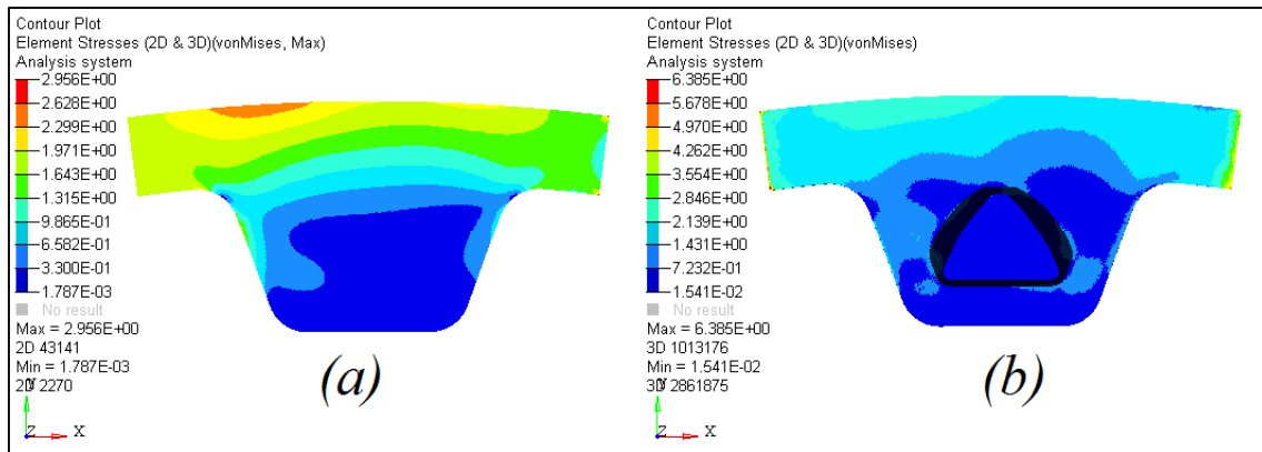
Figura 4.12. Distribución de esfuerzos, en megapascales (MPa), para las cargas T_1 y F_1(49.4973^\circ) . (a) Antes de la optimización. (b) Después de la optimización.
