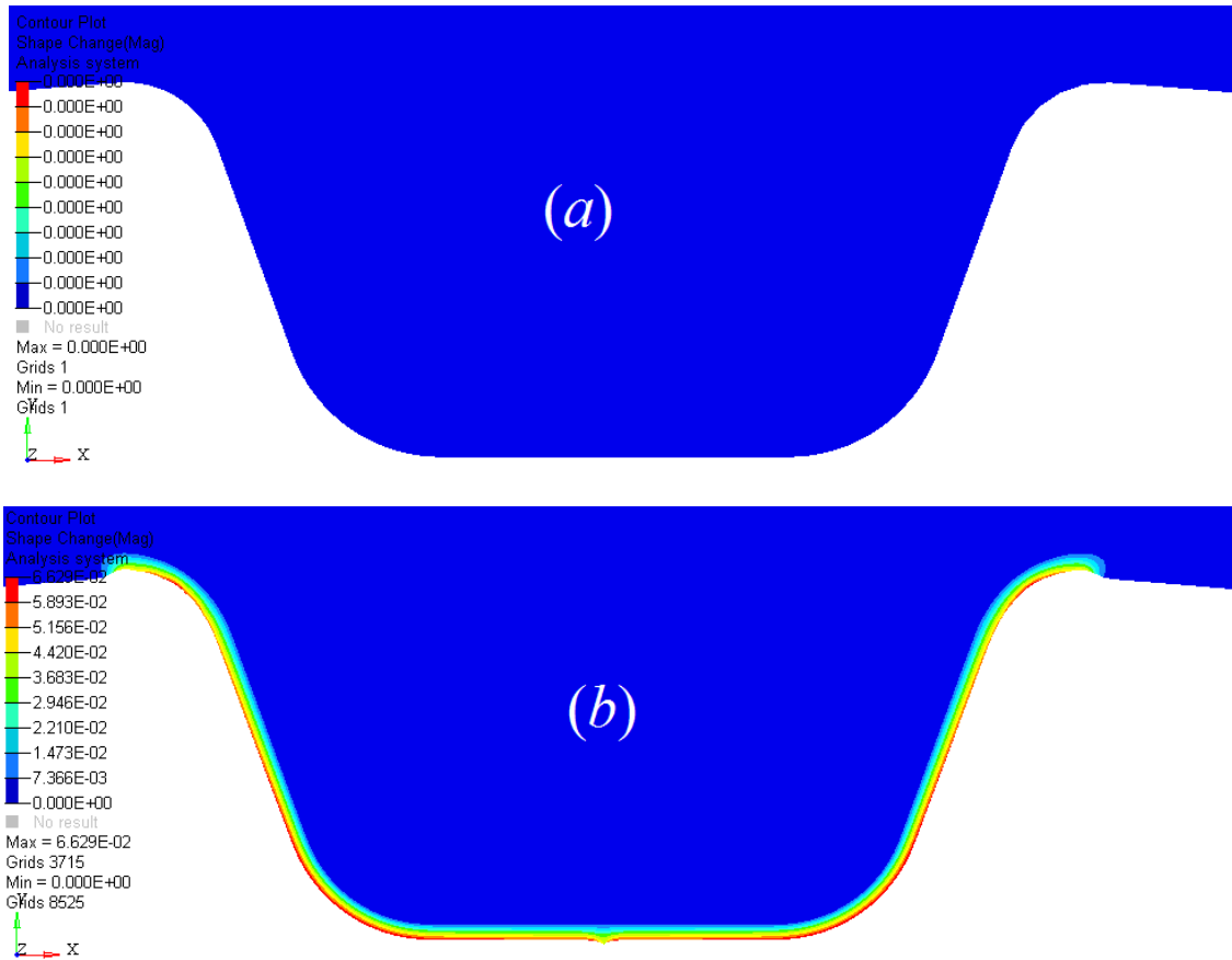
Figura 3.17. (a) Forma inicial del diente durante la optimización (iteración cero). (b) Forma final del diente durante la optimización.
