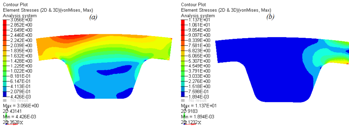
Figura 3.10. Distribución de esfuerzos, en megapascales (MPa), para (a) T_1 y F_1(45.7521^\circ) , (b) T_2 y F_{1,b}(45.7521^\circ) .
