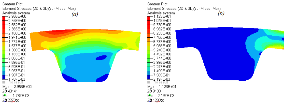
Figura 3.11. Distribución de esfuerzos, en megapascales (MPa), para (a) T_1 y F_1(49.4973^\circ) , (b) T_2 y F_{1,b}(49.4973^\circ) .
