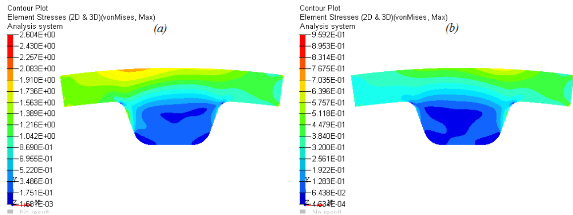
Figura 3.9. Distribución de esfuerzos, en megapascales (MPa), para (a) T_1 y F_1(48.71^\circ) , (b) T_2 y F_{1,b}(48.71^\circ) .
