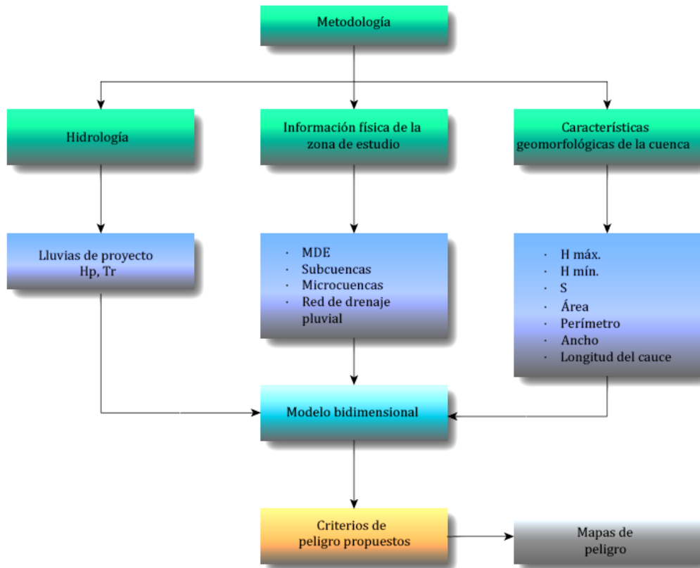
Figura 5-10 Metodología propuesta para la generación de mapas de peligro por inundación
