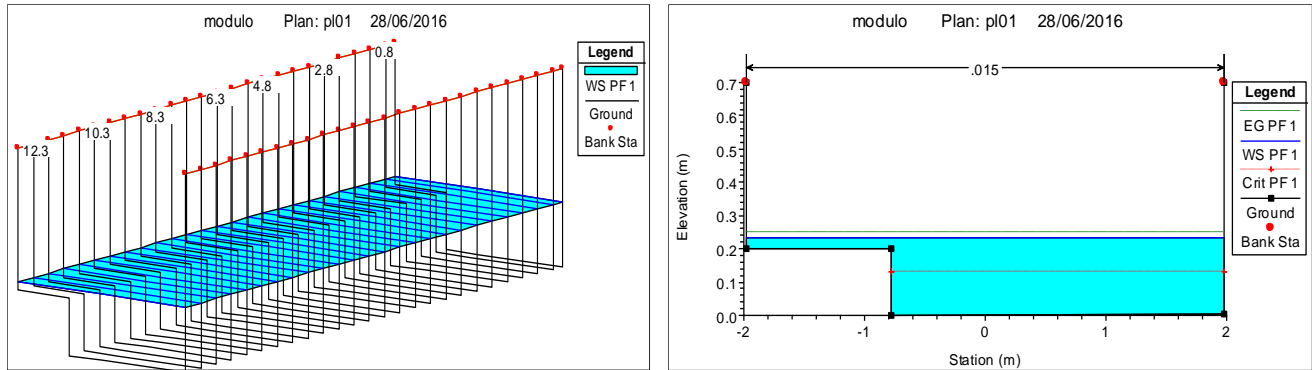
Figura 4-71 Perfil longitudinal y sección transversal del módulo experimental en HEC – RAS para 400 l/s
