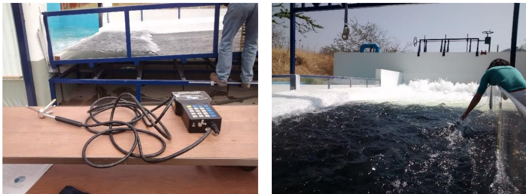
Figura 4-100 FlowTracker y empleo para medición de variables de velocidad
