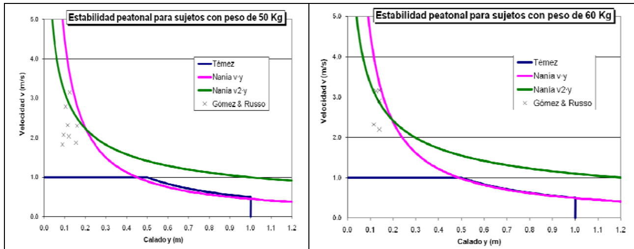
Figura 2-11 Regímenes de riesgo propuesto como una función de la profundidad y la velocidad
