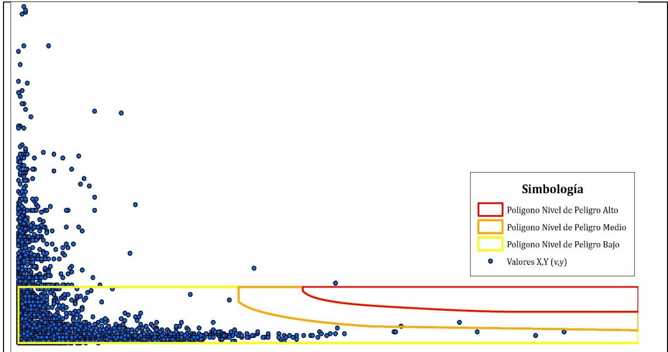
Figura 5-16 Dispersión de puntos x,y (Velocidad y Tirantes)
