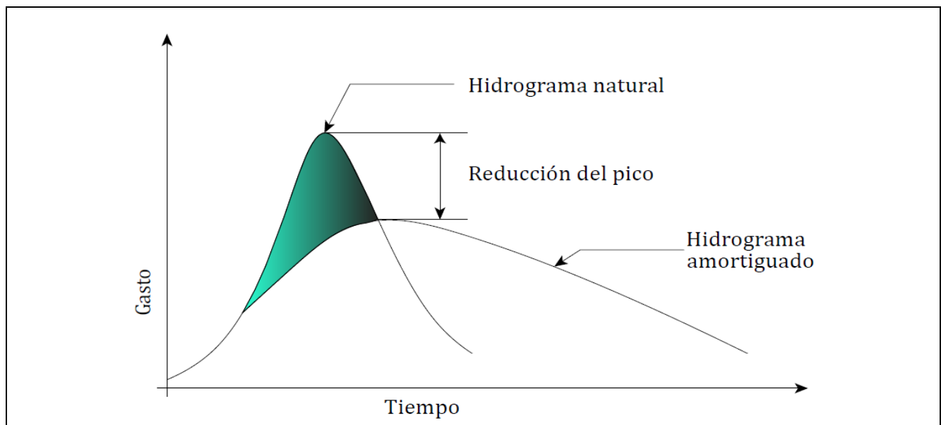
Figura 3-5 Comportamiento de hidrogramas en un reservorio
