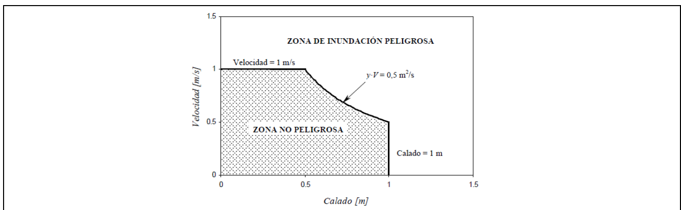
Figura 2-1 Nomograma de peligro por inundación. (Témez, 1992)
