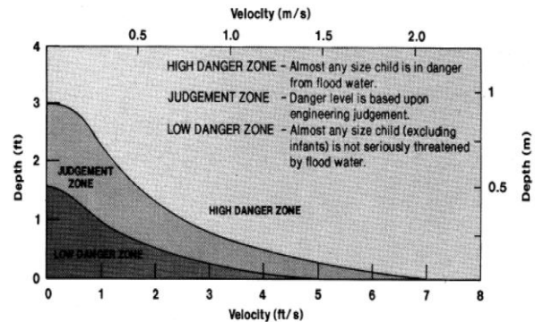
Figura 2-15 Representación de tirante - velocidad relación nivel de peligro de inundaciones en niños
