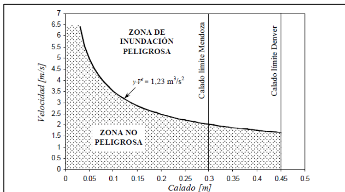
Figura 2-9 Criterio propuesto para la delimitación de la zona de inundación peligrosa
