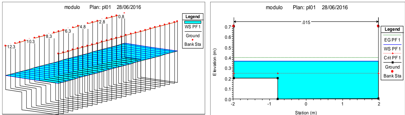
Figura 4-72 Perfil longitudinal y sección transversal del módulo experimental en HEC – RAS para 1000 l/s Fuente: elaboración propia.
