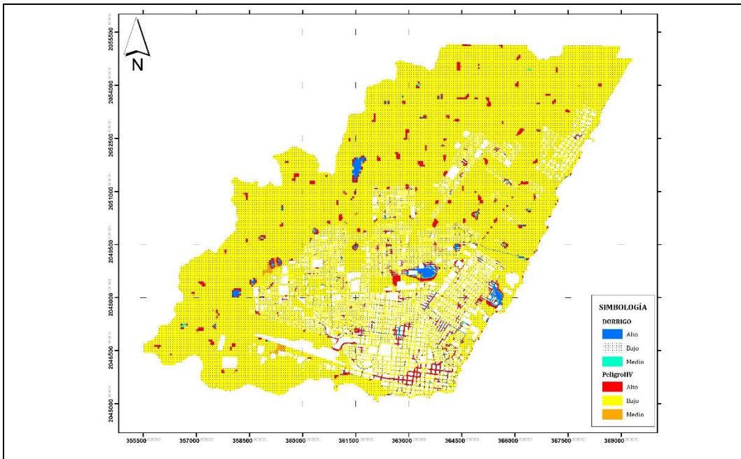
Figura 6-15 Comparativa de mapas de peligro (Dorrigo vs IMTA) para un Tr de 5 años (Mujeres)
