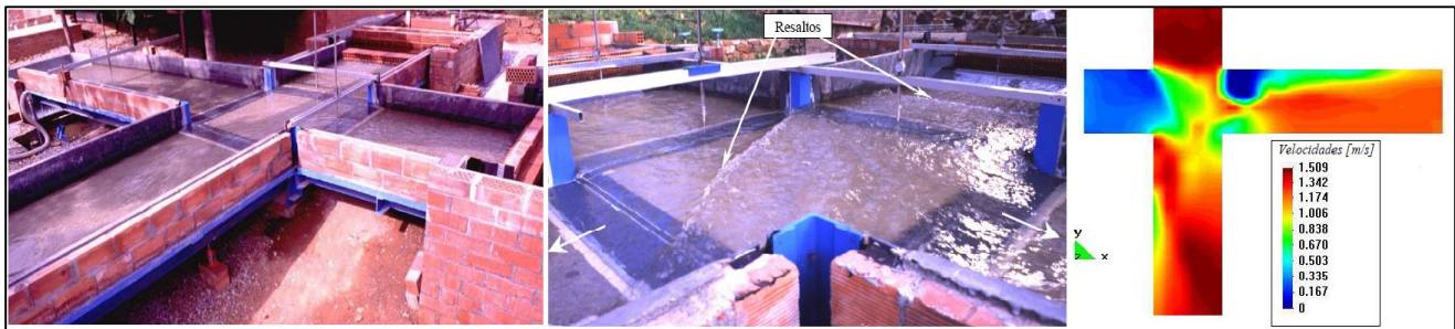
Figura 2-8 Módulos experimental y modelo numérico (distribución de tirantes y velocidades)
