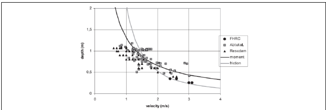
Figura 2-7 Combinaciones de tirante - velocidad
