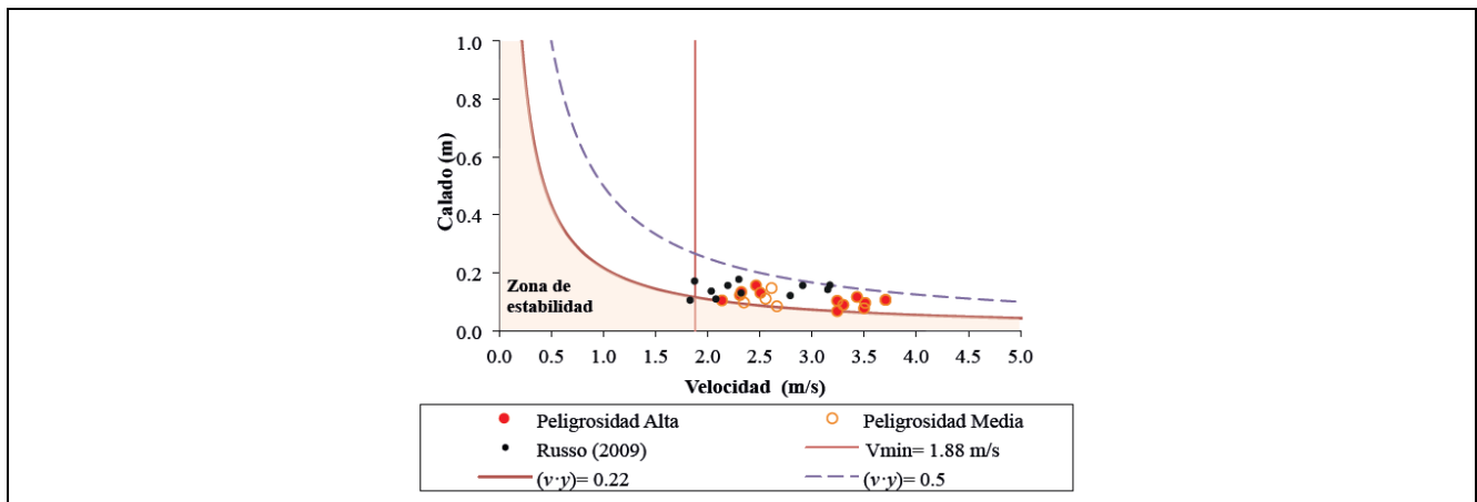
Figura 2-13 Representación de las condiciones hidráulicas (velocidad y tirante) que han generado situaciones de peligro medio y alto. Velocidad crítica 1.88 m/s
