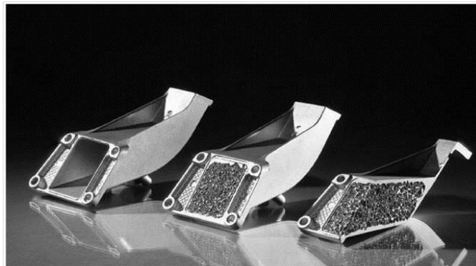
Figura 3: Parachoques con núcleo de espuma metálica [4].
