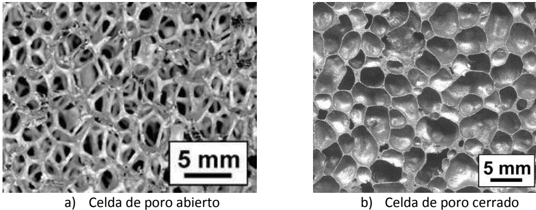
Figura 1: Tipos de celdas en espumas metálicas [1].
