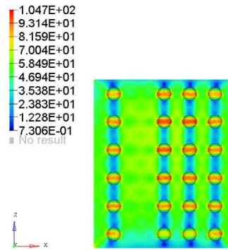
Figura 24: Resultados de esfuerzo - probeta de 120 poros.
