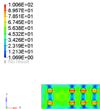
Figura 26: Resultados de esfuerzo - probeta de 40 poros.
