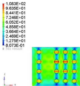
Figura 25: Resultados de esfuerzo - probeta de 80 poros.
