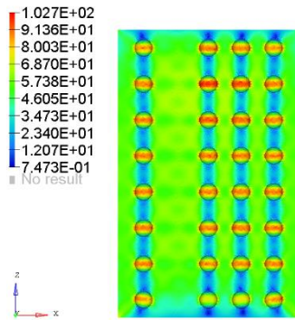
Figura 23: Resultados de esfuerzo - probeta de 160 poros.
