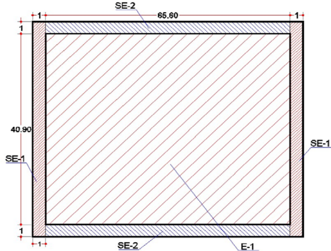
Excavación a 50 cm de prof.
