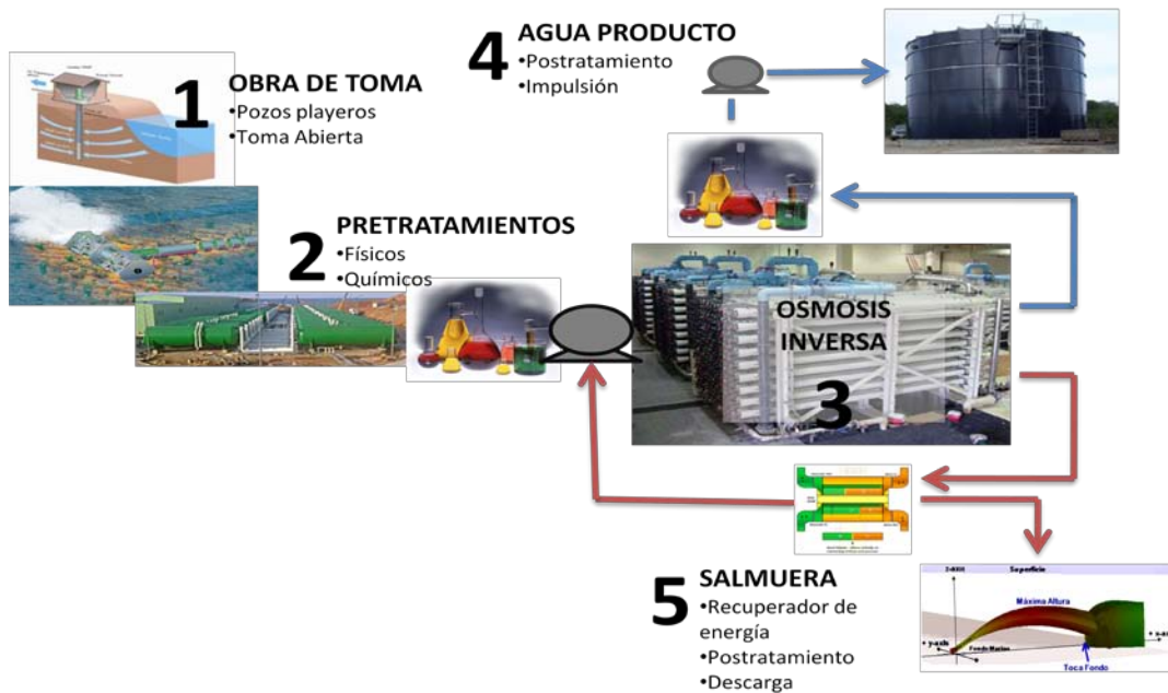
Figura 1: Diagrama de desalación
